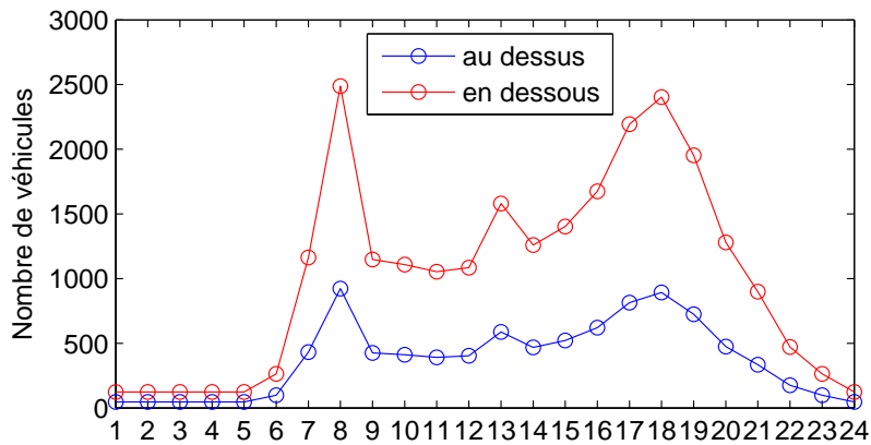
Figure 3.3.16: Distribution journalière du trafic pour la famille B (FCTUC 2012, SBRI 2013a).
