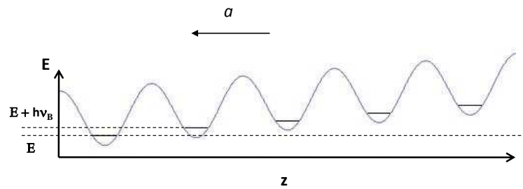
FIG. 1.1 – Levée de la dégénérescence des niveaux atomiques en présence d'une accélération.
