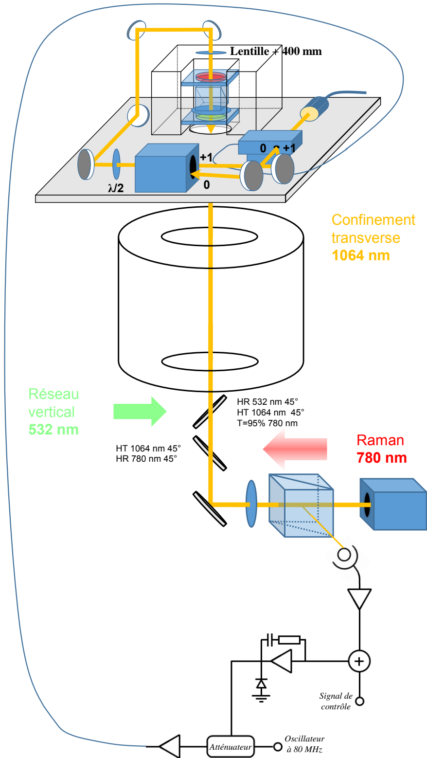
FIG. 4.19 – Banc optique et schéma de principe de l'asservissement en puissance du laser réalisant le confinement transverse des atomes.
