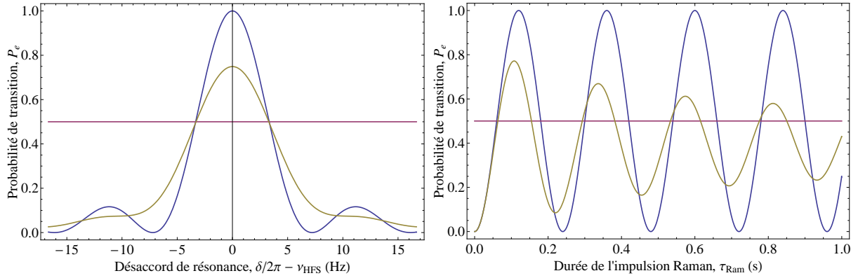
FIG. 2.24 – À gauche : Transformée de Fourier de l'impulsion Raman carrée de durée \tau_{\text{Ram}} = 120 ms lors du balayage du désaccord des Raman \delta = \omega_{R1} - \omega_{R2} - \omega_{\text{HFS}} . À droite : Oscillations de Rabi entre les deux niveaux d'énergie de l'atome en fonction de la durée d'application des Raman pour \delta = 0 Hz. Pour \Omega_R/2\pi = 4,2 Hz pour \delta = 0 et \sigma_{\text{inhom}} = 2,5 Hz, avec (en jaune foncé) ou sans (en bleu) inhomogénéités de déplacements lumineux différentiels.
