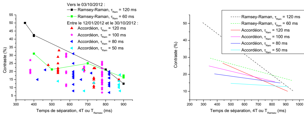
FIG. 5.37 – Franges d'interférence en sortie de l'interféromètre Accordéon en fonction de la durée d'interrogation 4T pour différentes durées d'impulsion \tau_{\text{Ram}} . Le contraste d'un interféromètre de Ramsey-Raman à la même période de l'année y est comparé aussi. Droite : les points de mesures ; gauche : les droites de régression linéaire de chacun des groupes de mesures.
