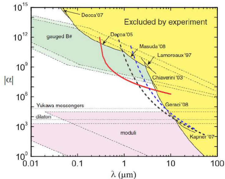
FIG. 1.5 – Plan (\alpha - \lambda) dans la plage des faibles distances. Les courbes bleu, rouge et noir sont différentes sensibilités accessibles par l'expérience ForCa-G selon différentes configurations [Messina et al. , 2011].
