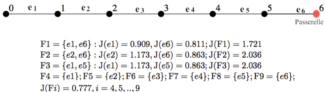
FIGURE 5.1.: Illustration d'un exemple d'ordonnancement avec contrôle de puissance : la consommation énergétique d'un nœud dépend de l'intensité d'interférences générée par les autres communications.
