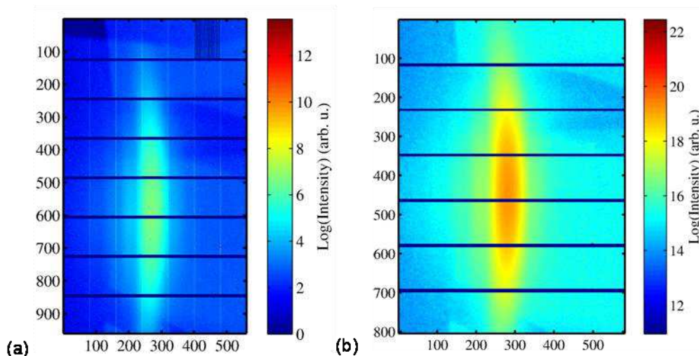
Figure 2.11. (a) Image brute collectée par le XPAD autour du pic 002Pd 2 Si/Si(111) (à 8 keV). (b) Image après correction géométrique.
