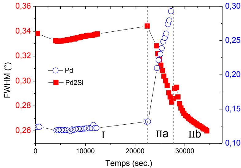
Figure 3.7. Largeur à mi-hauteur dans la direction 2θ des pics de Bragg 002\text{Pd}_2\text{Si} (carrés rouges et échelle de gauche) et 111\text{Pd} (ronds bleus et échelle de droite) d'un échantillon de \text{Pd}(48\text{ nm})/\text{Si}(111) recuit in situ sur la ligne DiffAbs.
