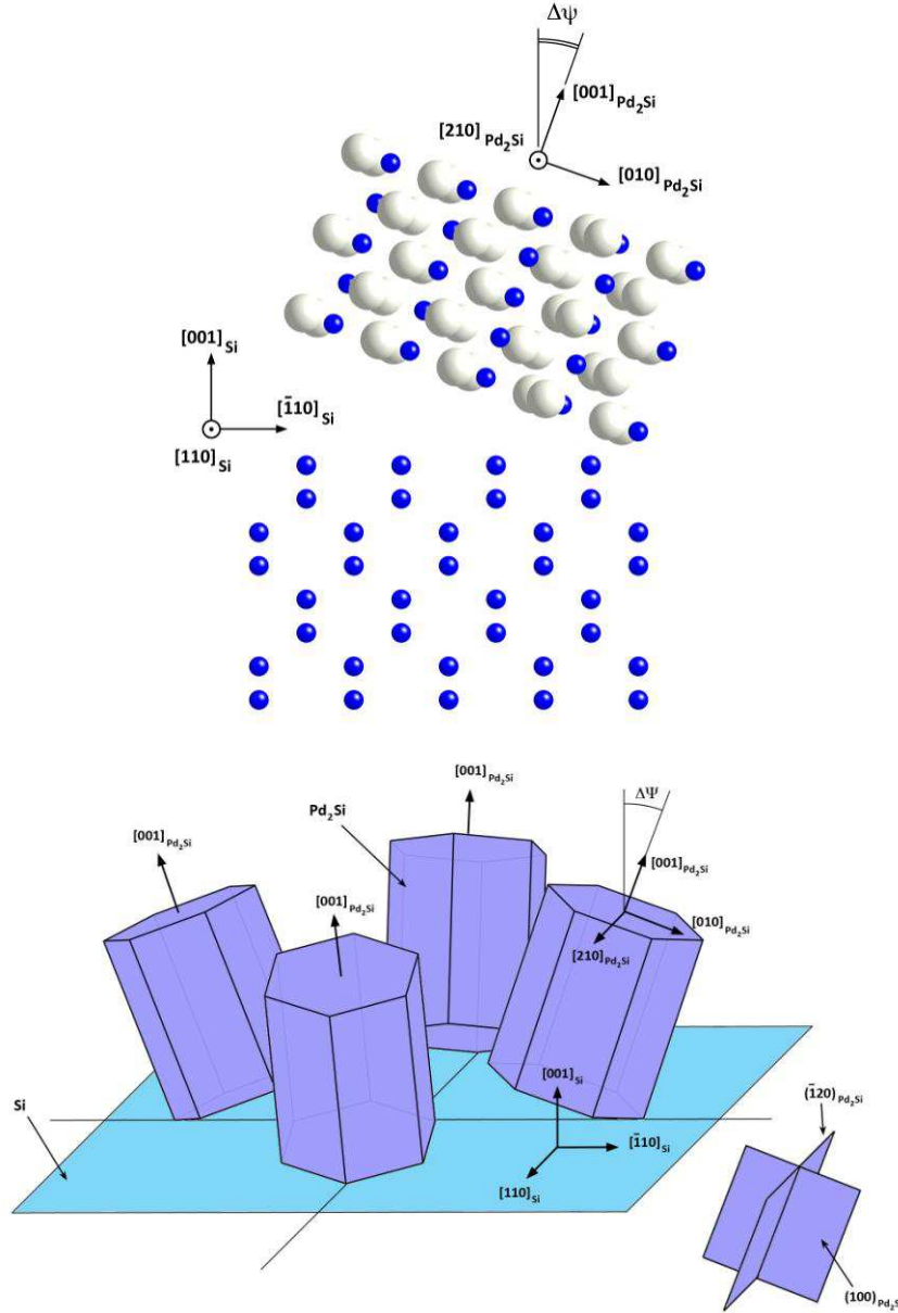
Figure 4.15. En haut: représentation schématique des structures de \text{Pd}_2\text{Si} et \text{Si} . En bas: schéma représentant les 4 variants de la maille de \text{Pd}_2\text{Si} désorientés les uns par rapport aux autres de 90^\circ dans le plan du film. La désorientation entre les plans (001)\text{Pd}_2\text{Si} et (001)\text{Si} et entre les plans (1\bar{1}0)\text{Pd}_2\text{Si} et (1\bar{1}0)\text{Si} n'est représentée que pour l'un des quatre variants (celui de droite).
