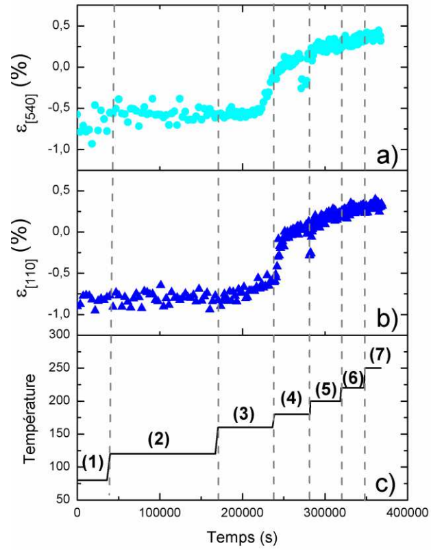
Figure 4.23. Variation des déformations suivant les directions [540] et [110] déduites des distances interréticulaires d_{210, \text{Pd}_2\text{Si}} et d_{110, \text{Pd}_2\text{Si}} mesurées au cours du traitement thermique de l'échantillon Pd(48 nm)/Si(001) défini dans la section 2c.
