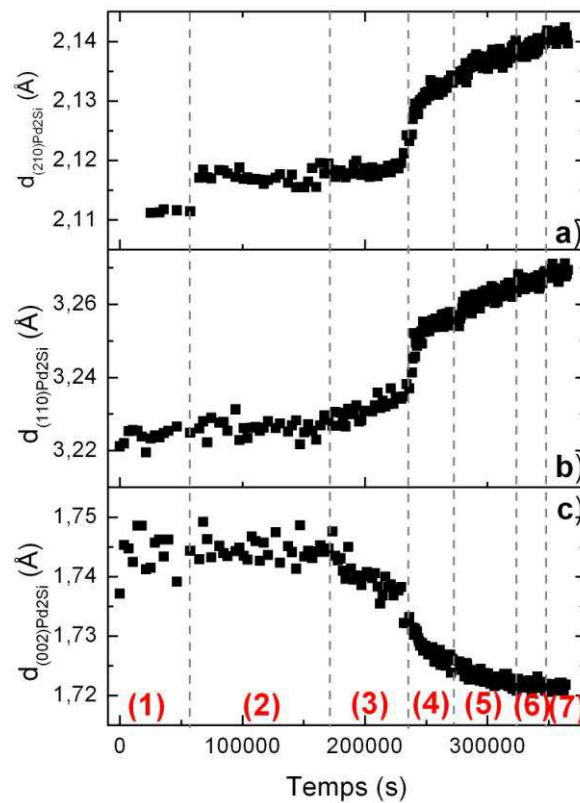
Figure 4.9. Evolution des paramètres d_{210,\text{Pd}_2\text{Si}} (a), d_{110,\text{Pd}_2\text{Si}} (b) et d_{002,\text{Pd}_2\text{Si}} (c) au cours du recuit au laboratoire d'un échantillon Pd(48 nm)/Si(001). Cet échantillon a subi plusieurs isothermes : 80 °C (étape 1), 120 °C (étape 2), 160 °C (étape 3), 180 °C (étape 4), 200 °C (étape 5), 220 °C (étape 6) et 250 °C (étape 7).
