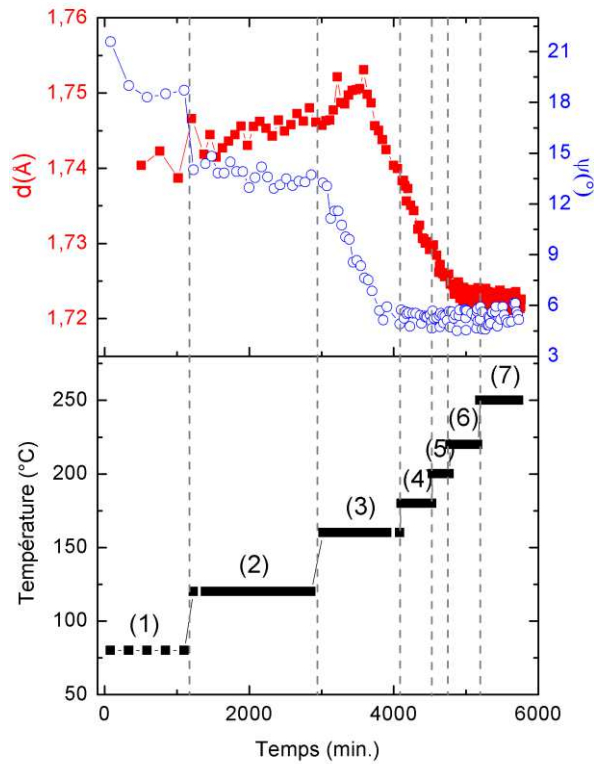
Figure 4.20. Evolution du paramètre d_{002,Pd_2Si} (carrés rouges), de l'angle \psi (cercles bleus) du pic de Bragg 002Pd_2Si et de la température au cours du traitement thermique subi par l'échantillon Pd(48 nm)/Si(001) au laboratoire. L'échantillon a été recuit à 80 °C pendant 21h (étape 1), puis à 120 °C pendant 32h (étape 2), à 160 °C pendant 17h (étape 3), à 180 °C pendant 7h (étape 4), à 200 °C pendant 14h (étape 5), à 220 °C pendant 6h (étape 6) et à 250 °C pendant 4h (étape 7).
