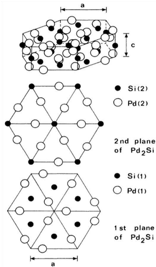
Figure 2. Schéma de la maille hexagonale du Pd 2 Si.
