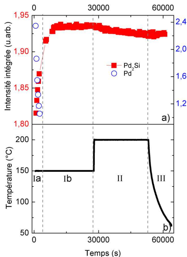
Figure 4.5. Evolution de l'intensité intégrée (a) des pics de Bragg 111 Pd (cercles bleus) et 002 Pd 2 Si (carrés rouges) et de la température (b) en fonction du temps, lors du recuit d'un échantillon de Pd(26 nm)/Si(001) sur la ligne DiffAbs.
