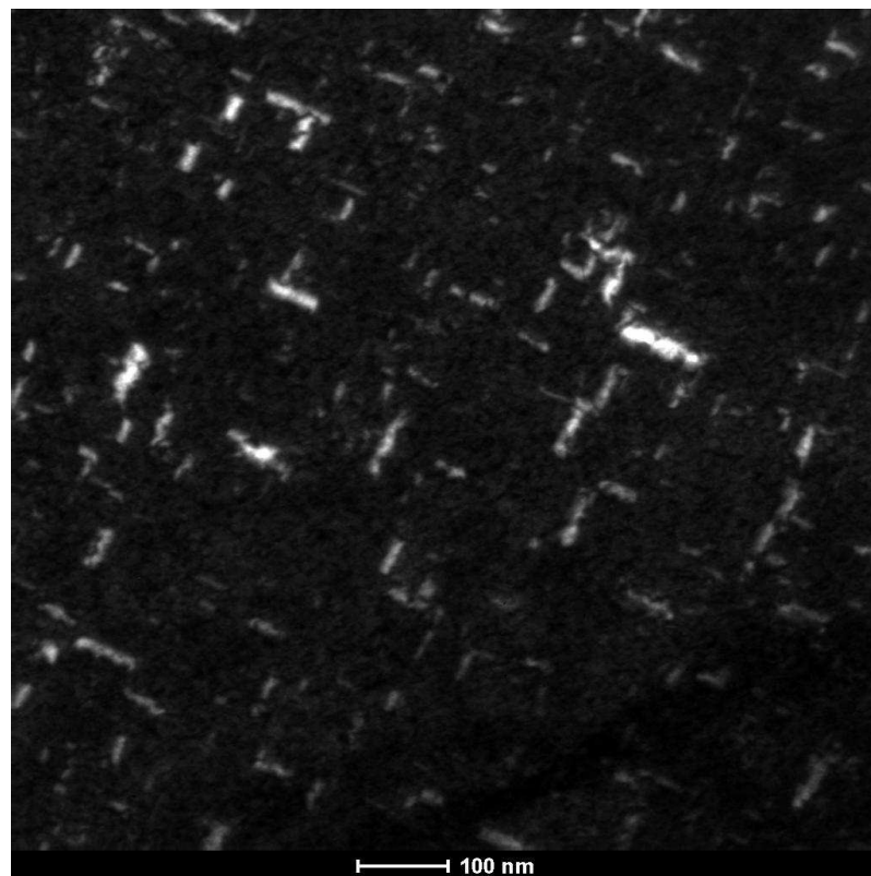
Figure 5.10. Micrographie MET en champ sombre et en vue plane d'un échantillon \text{Ni}(3\text{nm})/\text{Si}(001) recuit à 400\text{ }^\circ\text{C} . L'échantillon présente des couches cristallines formant des îlots, ainsi que de grandes surfaces dépourvues de ces îlots.
