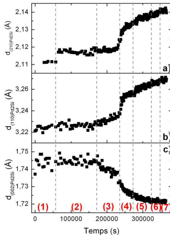
Figure 4.9. Evolution des paramètres d_{210,Pd_2Si} (a), d_{110,Pd_2Si} (b) et d_{002,Pd_2Si} (c) au cours du recuit au laboratoire d'un échantillon Pd(48 nm)/Si(001). Cet échantillon a subi plusieurs isothermes : 80 °C (étape 1), 120 °C (étape 2), 160 °C (étape 3), 180 °C (étape 4), 200 °C (étape 5), 220 °C (étape 6) et 250 °C (étape 7).
