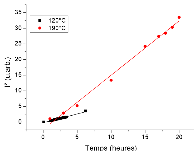
Figure 3.10. Variation du carré de l'intensité intégrée du pic de Bragg 002\text{Pd}_2\text{Si} pour l'échantillon \text{Pd}(48 \text{ nm})/\text{Si}(111) recuit à 120^\circ\text{C} pendant plus de 7 heures (carrés noirs), durant l'expérience couplée menée sur DiffAbs et pour un échantillon \text{Pd}(48 \text{ nm})/\text{Si}(111) recuit au laboratoire à 190^\circ\text{C} pendant 20 heures (cercles rouges).
