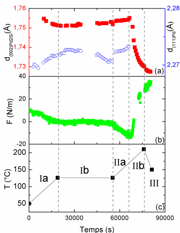
Figure 4.7. Evolution des distances interréticulaires (a) des plans (111)Pd (cercles bleus et échelle de droite) et (002) \text{Pd}_2\text{Si} (carrés rouges et échelle de gauche), de la force par unité de largeur obtenue par mesure de la courbure du substrat (b) et de la température (c) en fonction du temps, lors du recuit d'un échantillon de \text{Pd}(48 \text{ nm})/\text{Si}(001) sur la ligne DiffAbs.
