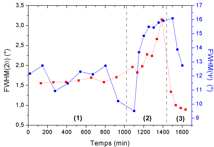
Figure 4.22. Evolution des largeurs à mi hauteur (FWHM) du pic de Bragg 002Pd 2 Si suivant 2\theta (carrés rouges) et suivant \Psi (cercles bleus) mesurées lors d'un recuit thermique réalisé au laboratoire d'un échantillon Pd(48 nm)/Si(001).
