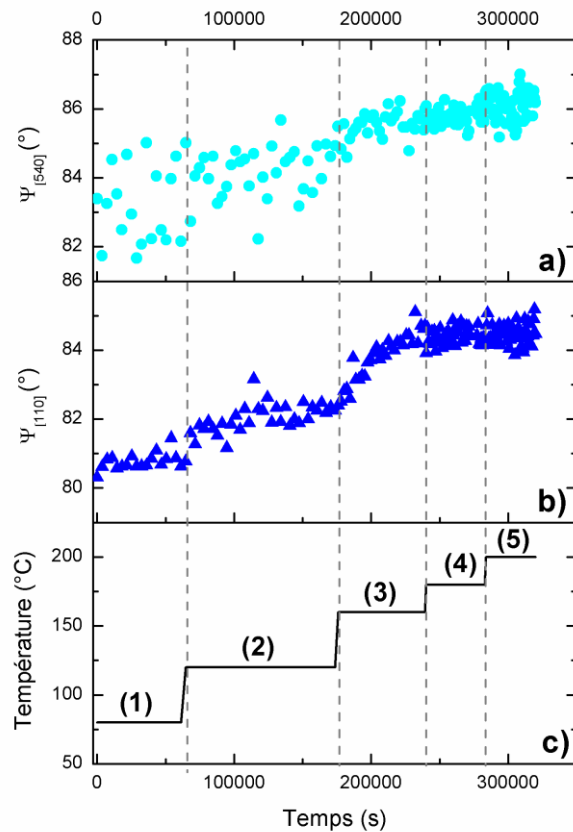
Figure 4.24. Variation des angles \Psi pour les pics de Bragg 110Pd 2 Si et 210 Pd 2 Si mesurés au cours des cinq premières étapes du traitement thermique de l'échantillon Pd(48 nm)/Si(001) défini dans la section 2c.
