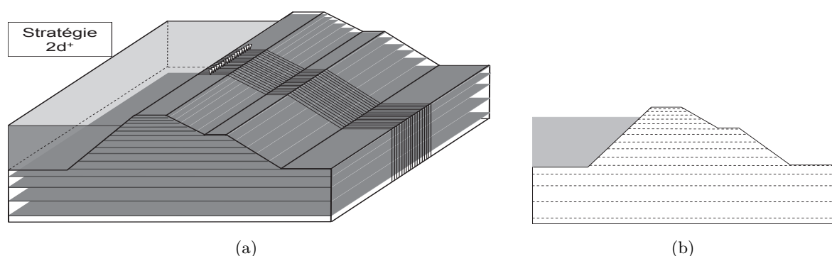
FIGURE 3.6 – Schématisation d’une discrétisation 2D^+ appliquée à un modèle de digue en charge (figure 3.6(a)). La distance finie des blocs dans le sens transversal permet une prise en compte de la topographie et du réservoir. La figure 3.6(b) présente une coupe transversale du bloc 3D illustré à la figure 3.6(a)
