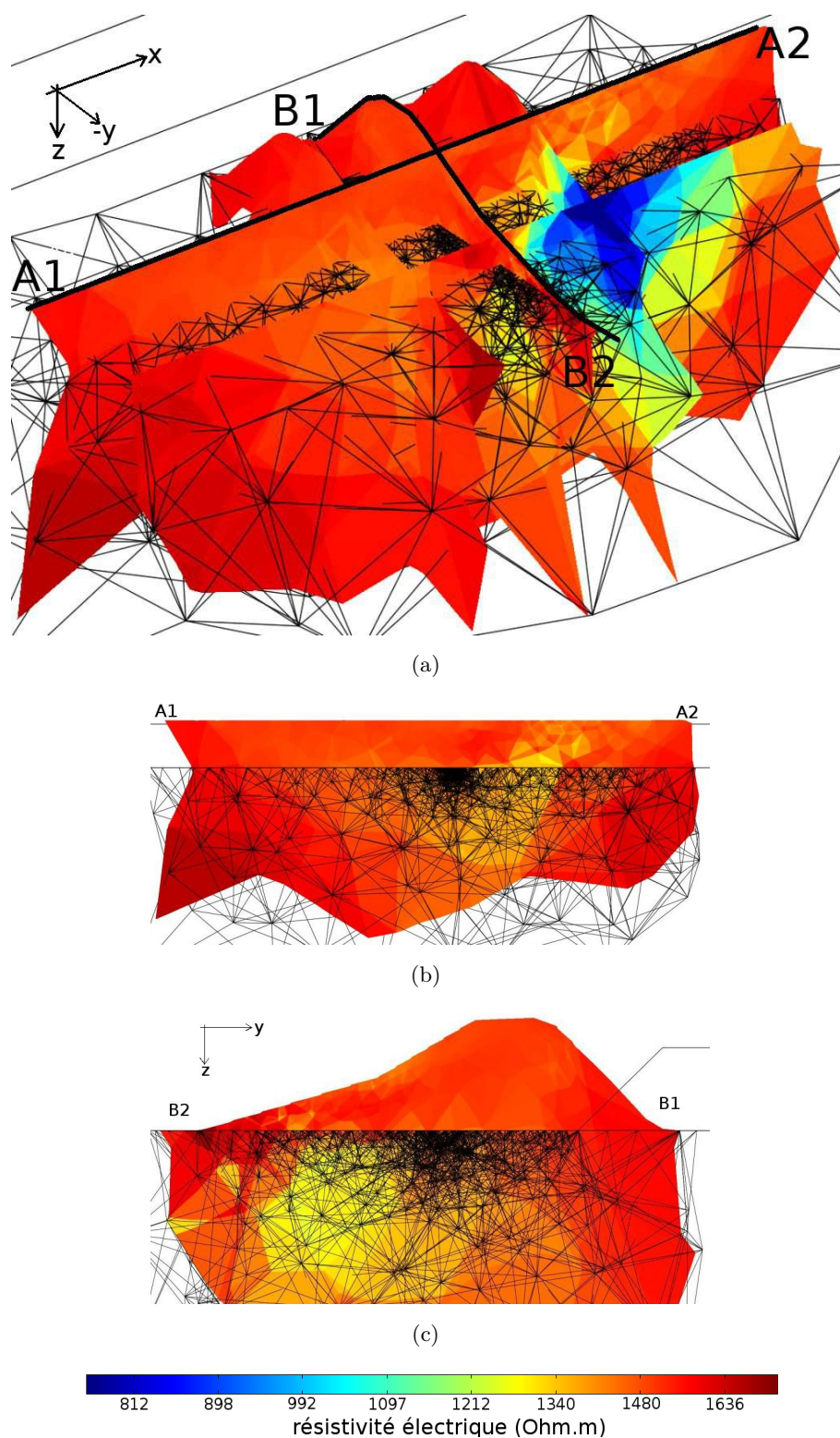
FIGURE 5.22 – Reconstruction issue de l'approche d'inversion ( InGEOHT - 3D^- ) à partir de données provenant de deux lignes d'électrodes placées transversalement et longitudinalement à la digue. La figure 5.22(a) présente une vue en perspective du résultat d'inversion à la troisième itération et les figures 5.22(b) et 5.22(c) deux coupes particulières extraites du bloc 3D. Ces deux coupes correspondent aux positions respectives des deux lignes d'électrodes (A1-A2 et B1-B2).
