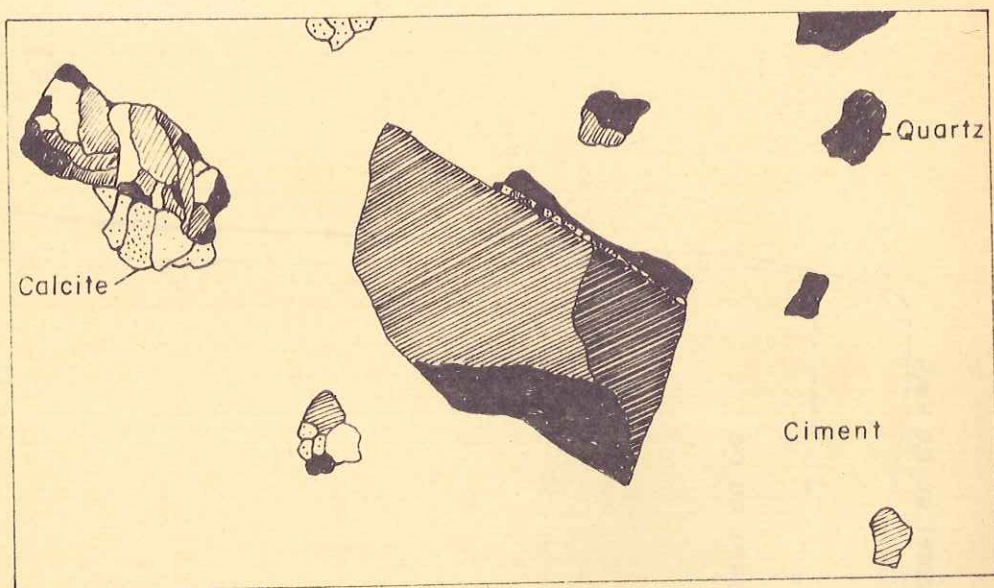
Remplacement du carbonate par le quartz = la forme losangique est conservée
