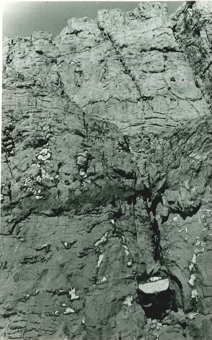
Pl. 9 - Photo A : Dalles de grès de base dégagée par l'érosion. Coupe n° 46. Gradin inférieur.
