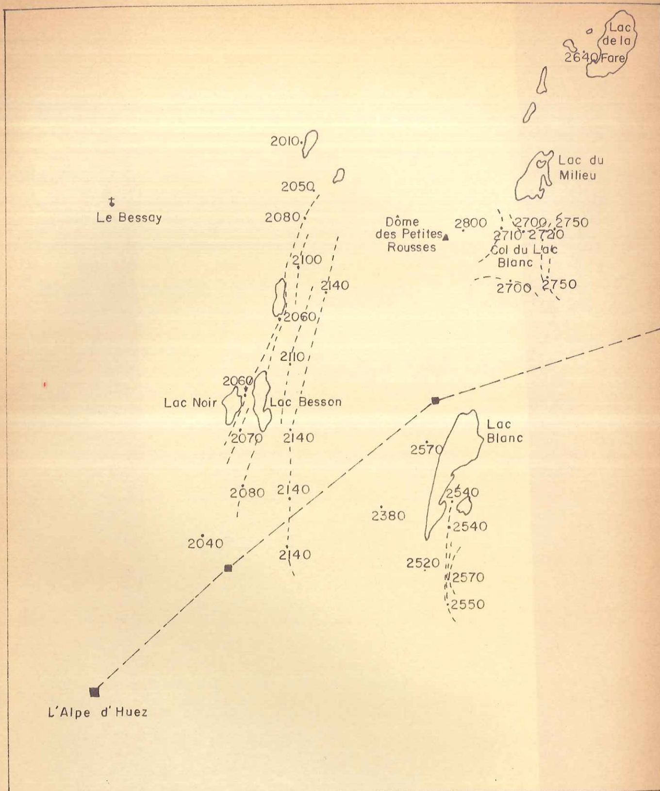
Pl. 22 - Altitude actuelle de la pénéplaine antétriasique
