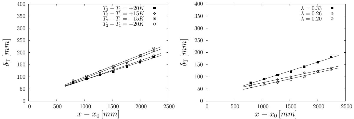
FIGURE 3.15 – Évolution longitudinale de l'épaisseur de la couche de mélange thermique \delta_T obtenue par PCTA : à gauche, pour les configurations \lambda = 0,33 , U_c = 3 m/s et différents \Delta T ; à droite, pour les configurations stable U_c = 3 m/s, \Delta T = 20 K et différents \lambda .
