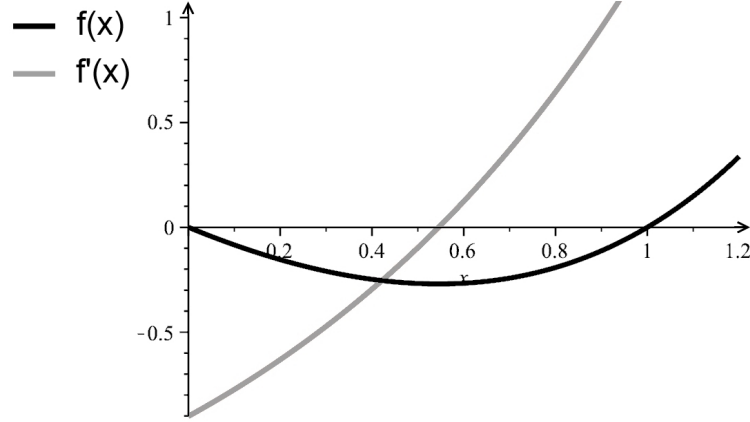
FIGURE 3.5 – Courbe représentatives de f(x) = 3^x - 2x - 1 et de sa dérivé
