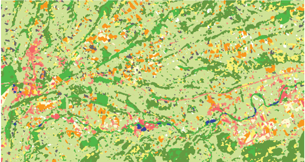
figure V.1 : Extrait de la classification des données Landsat-5 année 2011 à partir des statistiques interpolées, zone de la commune de Lannemezan
