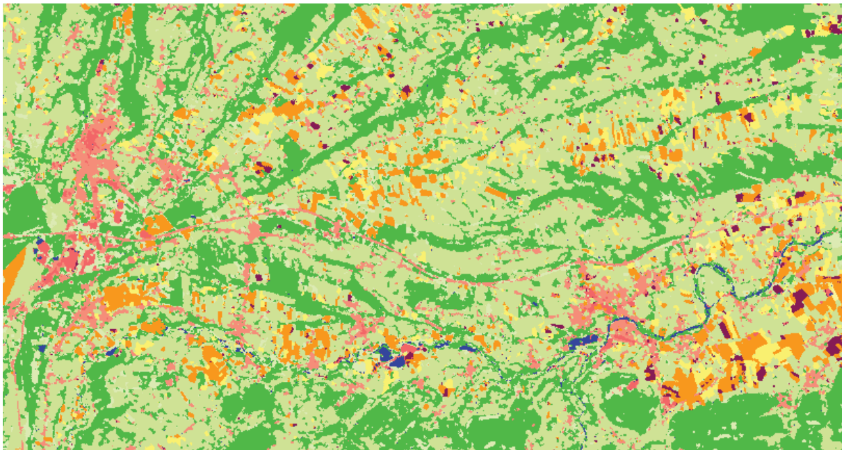
figure V.2 : Extrait de la classification des données Landsat-5 année 2011 à partir des vérités terrain, zone de la commune de Lannemezan
