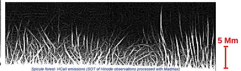
Limbe en H-Call avec le SOT de Hinode traité sous Madmax pour renforcer la visibilité Tavabi, Koutchmy 2013
