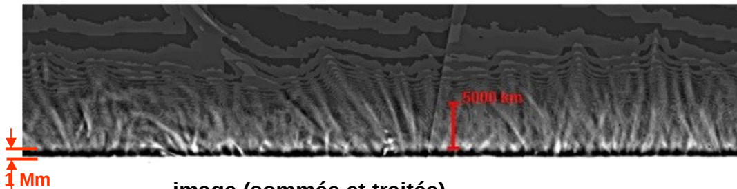
image (sommée et traitée) dans la raie H - Ca II du bord solaire SOT- Hinode (JAXA & NASA)
