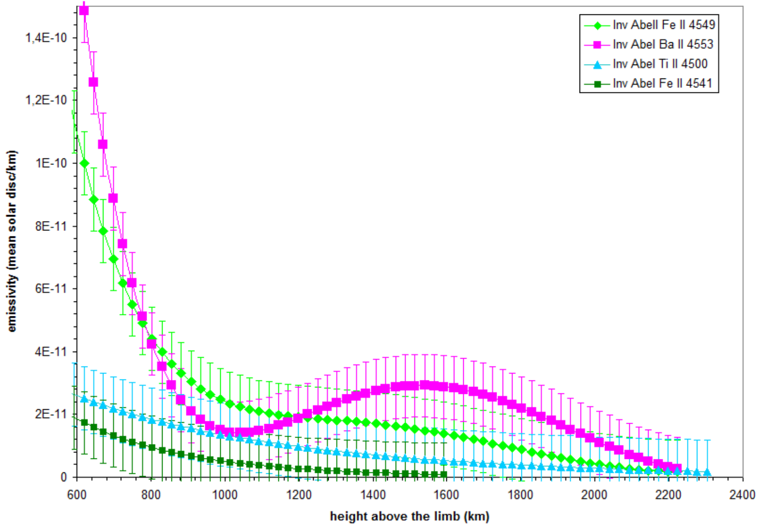
Emissivités des raies Fe II, Ti II, Ba II C2 du 22 Juillet 2009
