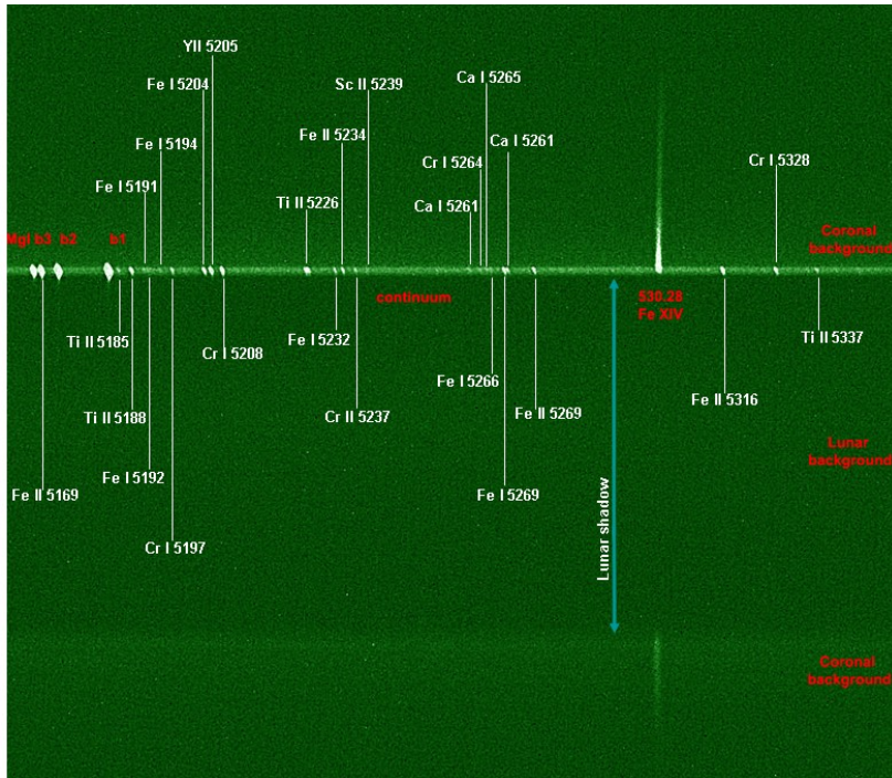
Spectrographe à fente S. Koutchmy, J. Certain éclipse du 13 Nov. 2013 Australie
