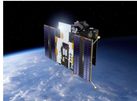
SWAP Proba2 (ESA) 174
