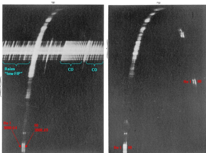
Hiei, 1963 (dans l'UV): 2 spectres sans fente/contact
