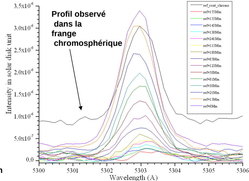
Profils transverses dans la raie du Fe XIV 5303
