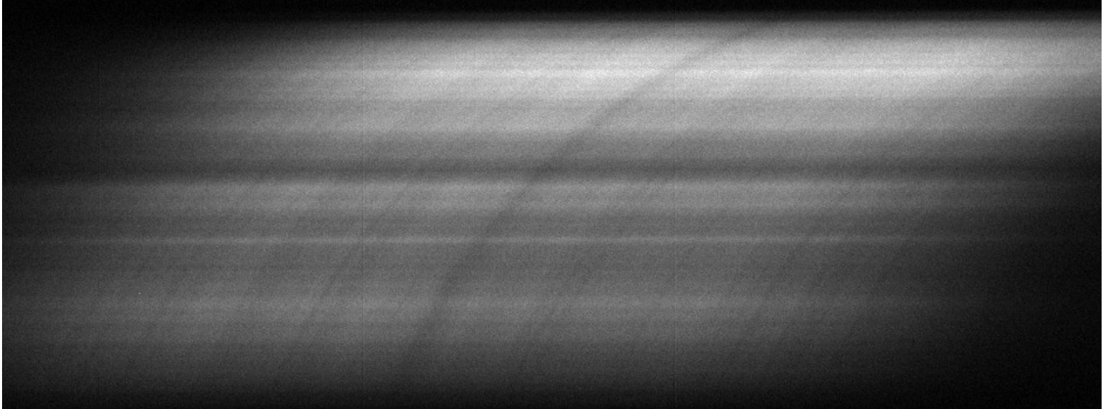
Avant éjection C2 eclipse 11 Juillet 2010 (frame 2599)
