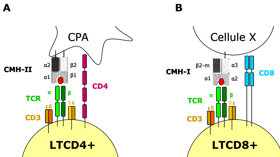
Figure 26 : Mécanisme de reconnaissance des LTCD4 + (A) et LTCD8 + (B).
