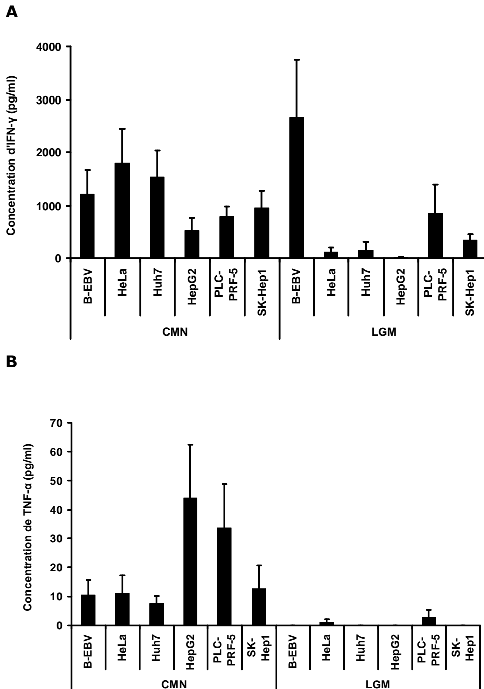
Figure 40 : Production d'IFN-γ (A) et de TNF-α (B) par les CMN et les LGM stimulés par différentes lignées cellulaires.
