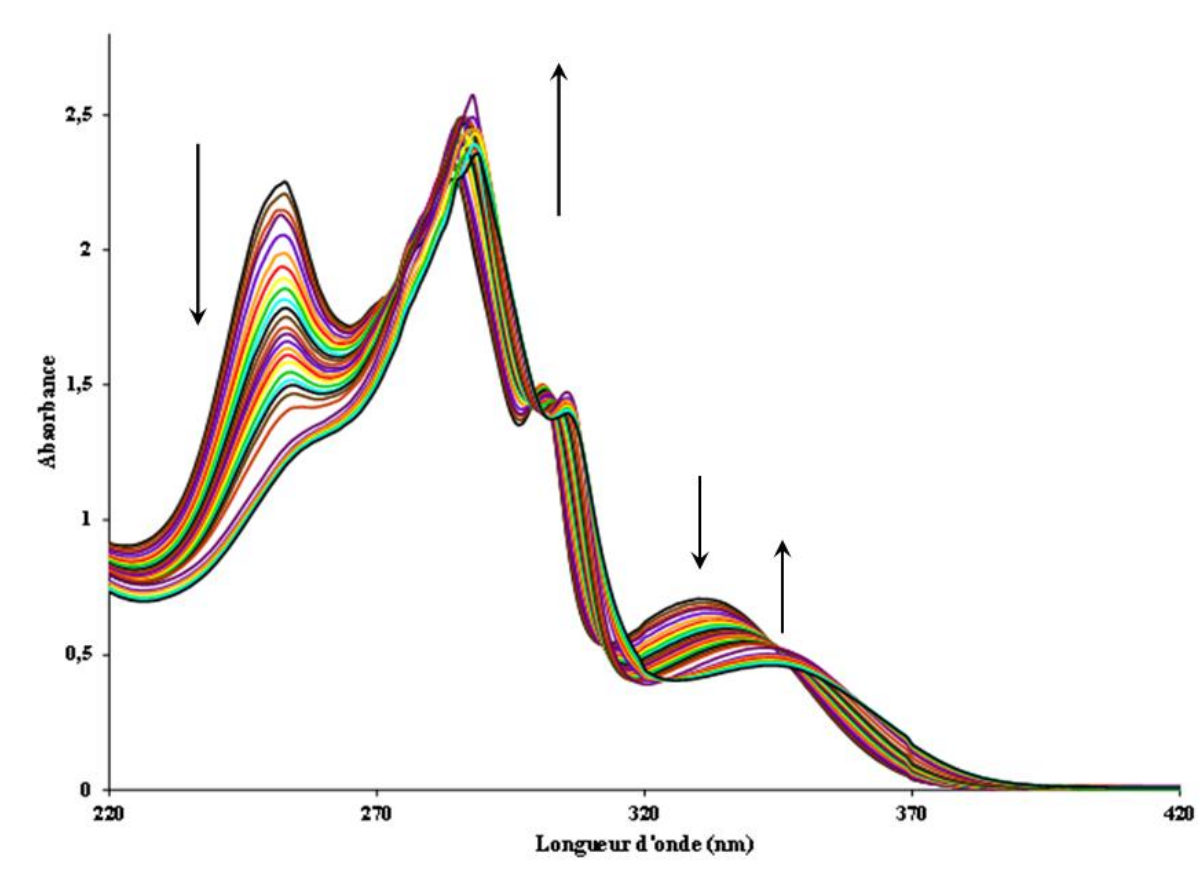
Figure 4.24 : Evolution du spectre d'absorption UV-Visible du ligand L 12 ( c = 2,49 \times 10^{-5} \text{ M} ) avec l'addition d'une solution d'EuCl 3 .6H 2 O ( c = 5 \times 10^{-4} \text{ M} ) à pH = 7,4. L'intensité d'absorption n'est pas corrigée pour la dilution.
