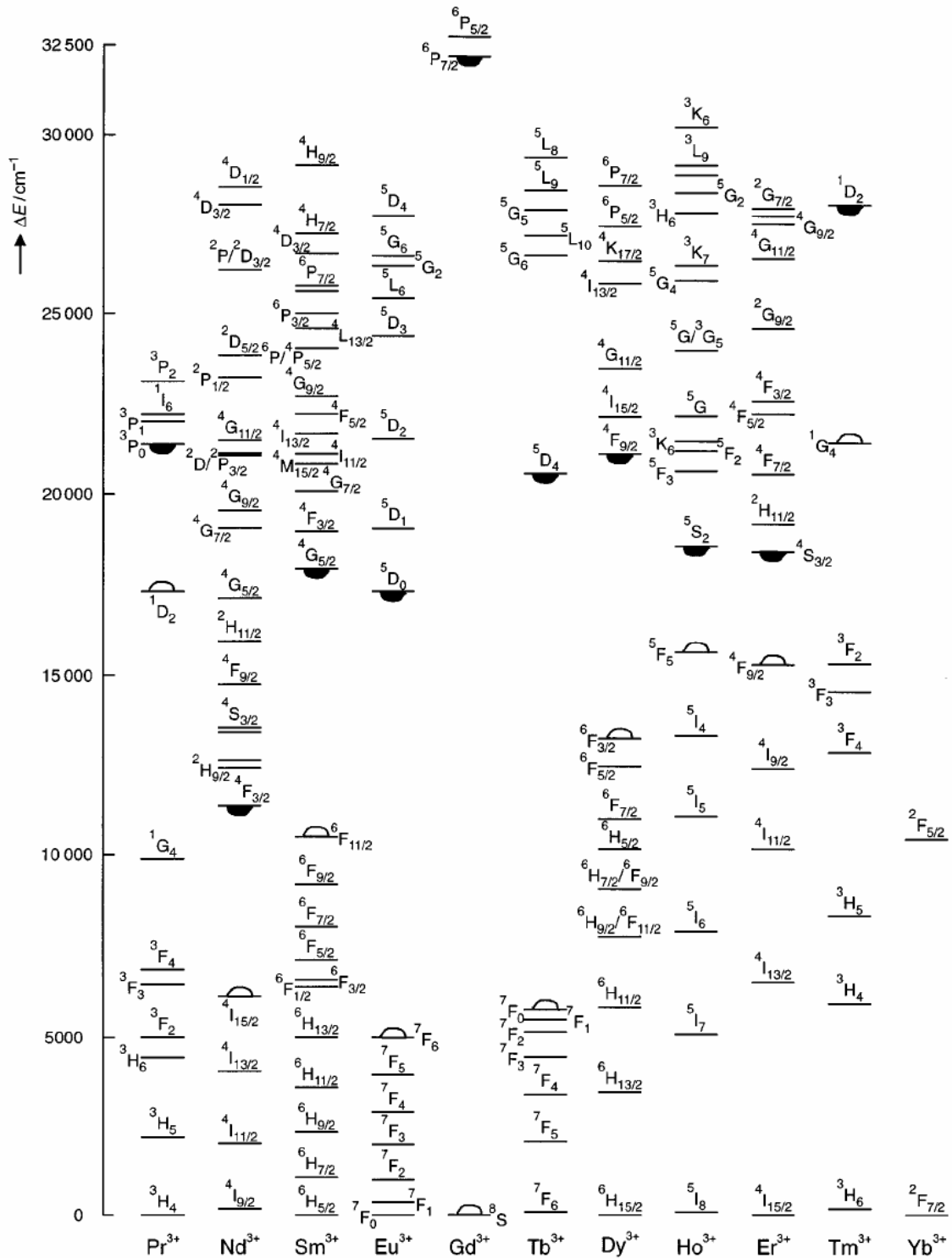
Diagramme 1.1 : Niveaux d'énergie des principaux ions lanthanides luminescents en solution aqueuse. Les niveaux luminescents les plus bas sont représentés en blanc ( \smile ) et les niveaux fondamentaux en noir ( \blacksmile ) [12] .
