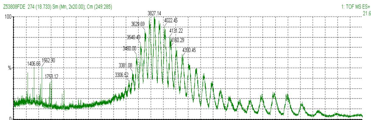
Figure 3.11 : Spectre de masse ESI + de l'anticorps Dreg55 après la réaction de marquage.
