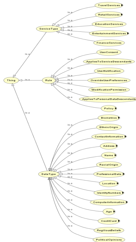
Figure 3.28 Concepts de l'ontologie de protection des données
