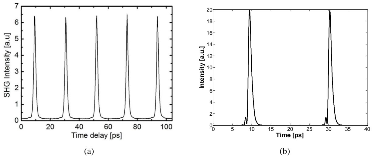
Figure 0-16. (a) Autocorrélation d'intensité pour le laser de 890 μm de long à deux sections en sortie de laser et (b) profil d'intensité de champ reconstruit correspondant pour un courant d'injection de 70 mA et une polarisation inverse de -1.5 V. [54]
