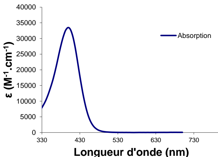
Figure 4. 11 Spectres d'absorption du salicylaldéhyde 4.1 dans l'acétone ( \mu = 2,88 D).
