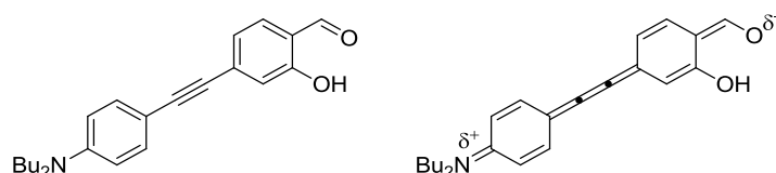
Figure 4. 8. Formes mésomères résonnantes du salicyaldéhyde 4.1 .
