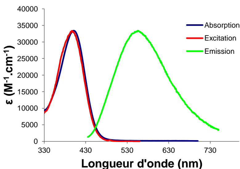
Figure 4. 10. Spectres d'absorption, d'émission ( \lambda_{\text{ex}} = 380 \text{ nm} ) et d'excitation ( \lambda_{\text{em}} = 570 \text{ nm} ) du salicyaldéhyde 4.1 dans le THF ( \mu = 1,75 \text{ D} ).
