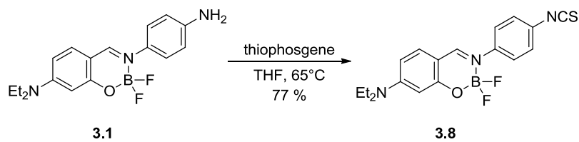
Figure 3. 56. Synthèse de l'isothiocyanate.
