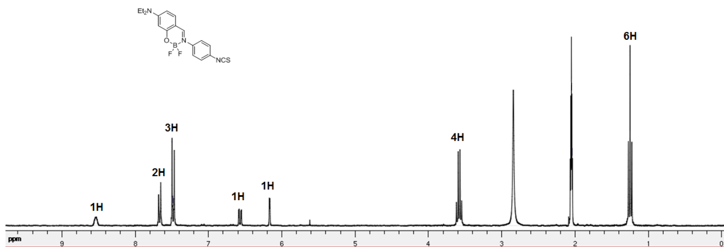
Figure 3. 57. RMN proton du Boranil 3.8 dans l'acétone- d 6 .
