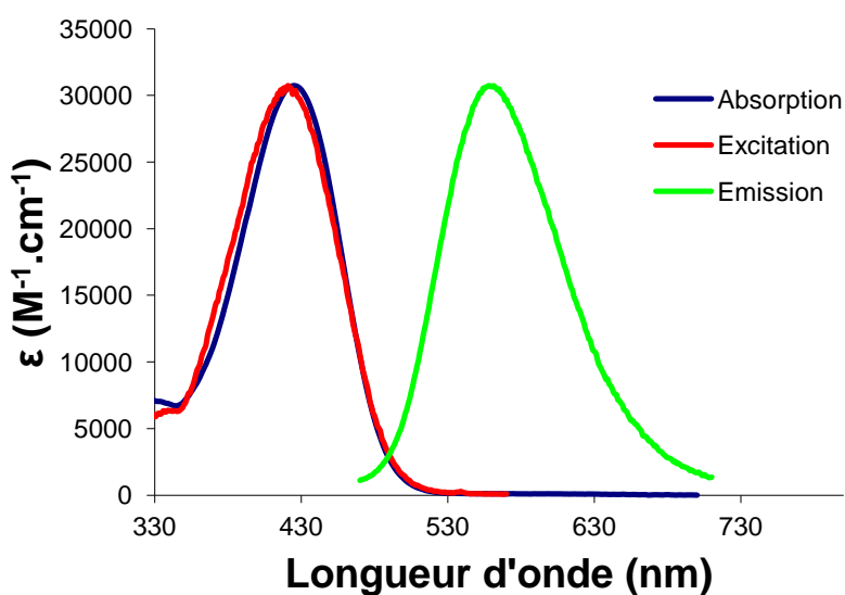
Figure 4. 17. Spectres d'absorption, d'émission ( \lambda_{\text{ex}} = 400 \text{ nm} ) et d'excitation ( \lambda_{\text{em}} = 640 \text{ nm} ) du salicyaldéhyde 4.2 dans le THF ( \mu = 1,75 \text{ D} ).
