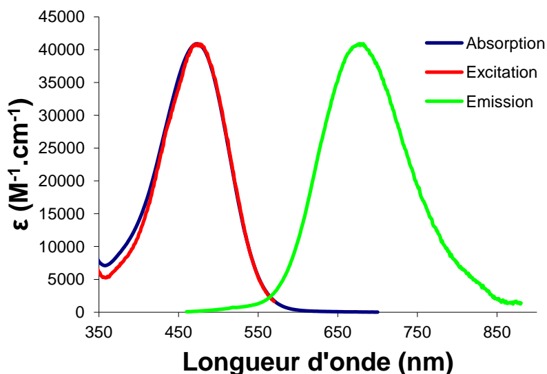
Figure 4. 46. Spectres d'absorption, d'émission ( \lambda_{\text{ex}} = 450 \text{ nm} ) et d'excitation ( \lambda_{\text{em}} = 700 \text{ nm} ) du Boranil 4.6 dans le THF ( \mu = 1,75 \text{ D} ).
