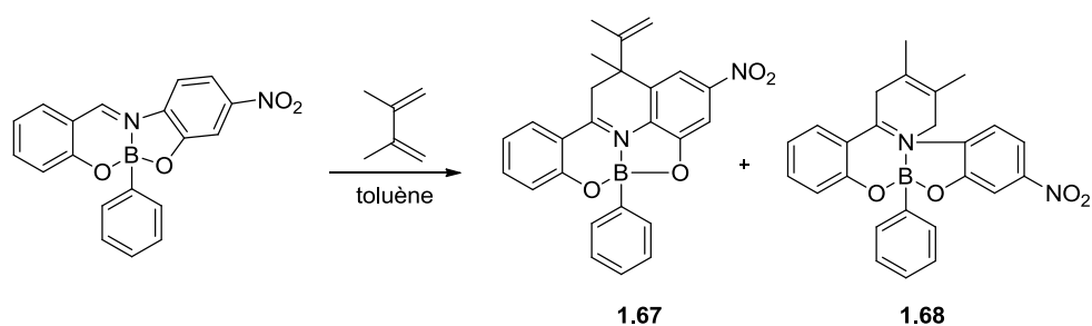
Figure 1. 36. Exemple de post-fonctionnalisation sur un dérivé de salicyldimine.
