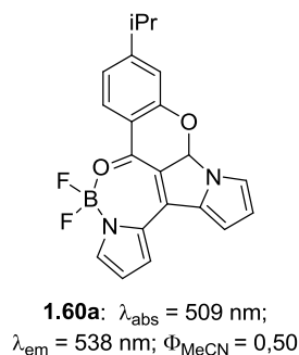
Figure 1. 47. Propriétés optiques d'un complexe borate N,B,O à 7 chaînons.
