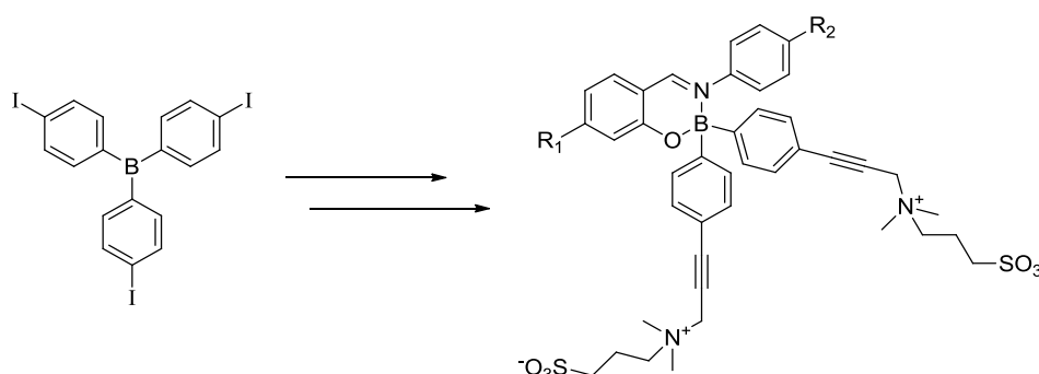
Figure 4. 54. Exemple d'utilisation de précurseurs de Bore spécifiques.
