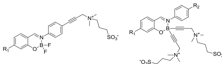
Figure 4. 53. Exemple de Boranils substitués par des sulfobétaïnes.
