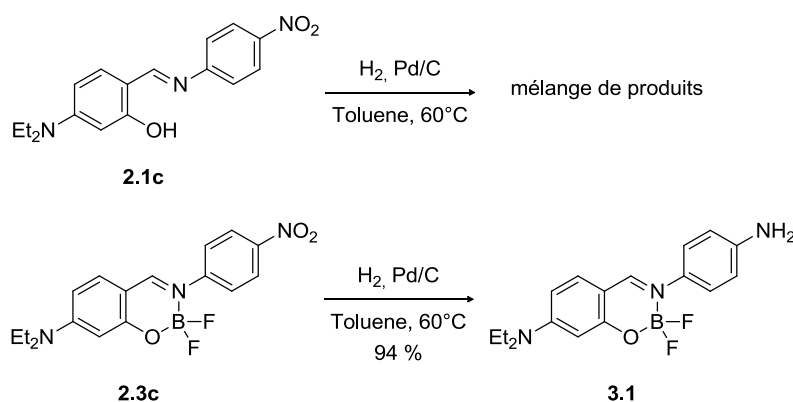
Figure 3. 22. Réduction catalysé au palladium de la fonction nitro du Boranil 2.3c .
