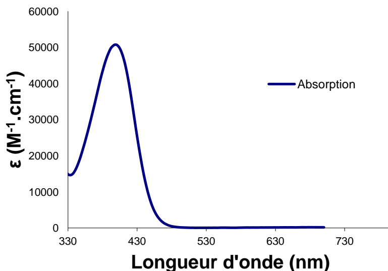
Figure 4. 25. Spectres d'absorption de l'anil 4.3 dans l'acétone ( \mu = 2,88 \text{ D} ).
