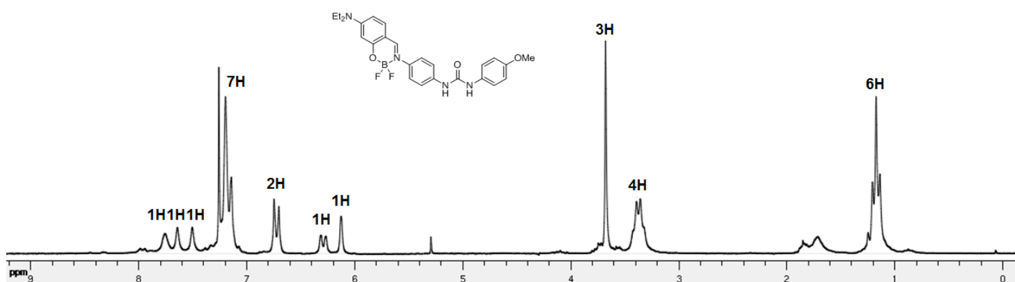
Figure 3. 42. RMN proton du Boranil 3.5 dans le CDCl_3 .
