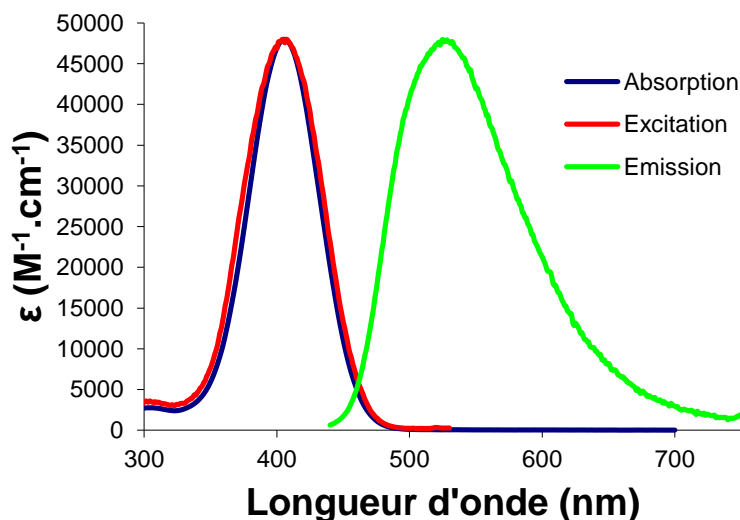
Figure 3. 25. Spectres d'absorption, d'émission ( \lambda_{ex} = 380 nm) et d'excitation ( \lambda_{em} = 540 nm) du Boranil 3.1 dans le dichlorométhane.
