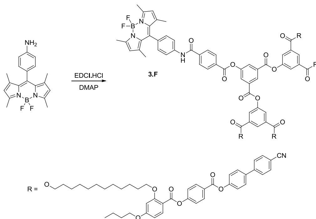
Figure 3. 19. Synthèse d'un BODIPY-arborol pour la génération de mésophase fluorescente.
