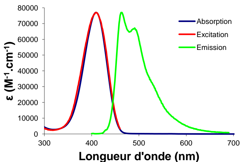
Figure 2. 46. Spectres d'absorption, d'émission ( \lambda_{\text{ex}} = 380 nm) et d'excitation ( \lambda_{\text{em}} = 490 nm) du Boranil 2.15 dans le toluène.
