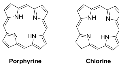
Figure 1. 18 Les porphyrines et les chlorines.
