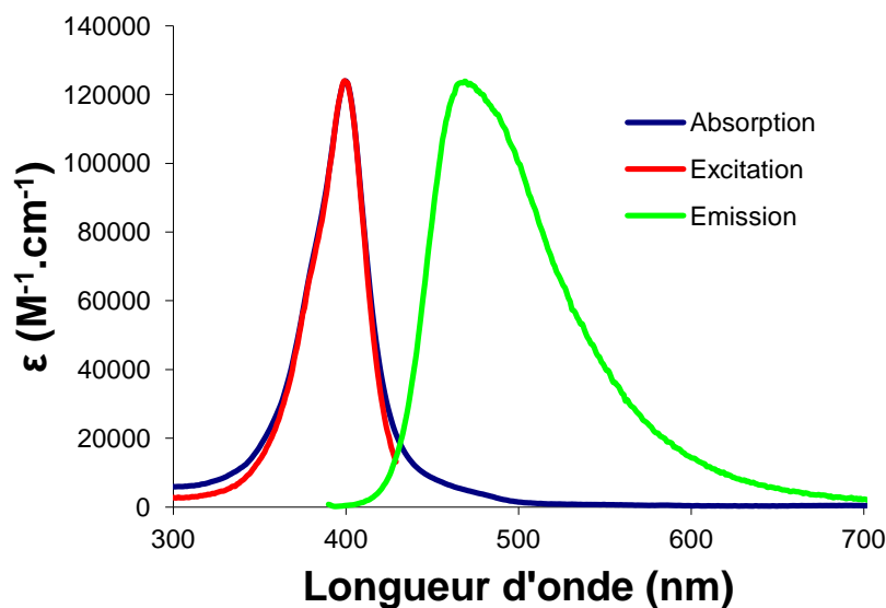
Figure 2. 30. Spectres d'absorption, d'émission ( \lambda_{\text{ex}} = 380 \text{ nm} ) et d'excitation ( \lambda_{\text{em}} = 500 \text{ nm} ) du diboranil-naphtalène 2.5 dans le dichlorométhane.
