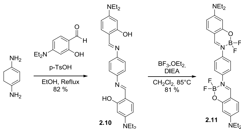
Figure 2. 36. Synthèse du para-diboranil.
