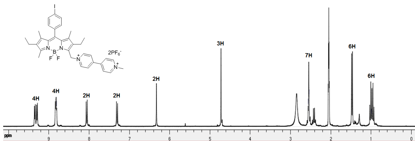
Figure 3. 5. RMN proton du BODIPY 3.A dans l'acétone- d_6 .
