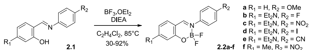
Figure 2. 4. Procédé synthétique des Boranils \text{BF}_2 2.2a-f .
