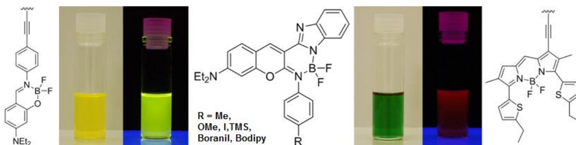
Figure 2. La famille des Boricos.
