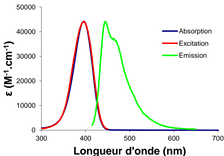
Figure 2. 13. Spectres d'absorption, d'émission ( \lambda_{ex} = 365 nm) et d'excitation ( \lambda_{em} = 470 nm) du Boranil 2.2b (Et 2 N/F/F) dans le toluène.
