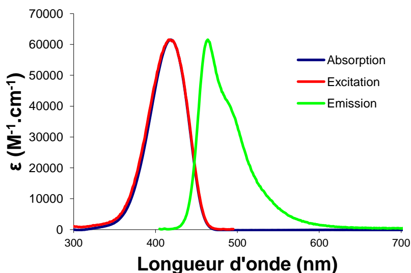
Figure 2. 23 Spectres d'absorption, d'émission ( \lambda_{ex} = 400 nm) et d'excitation ( \lambda_{em} = 500 nm) du Boranil 2.2e (Et 2 N/CN/F) dans le dichlorométhane ( \mu = 1,60 D).
