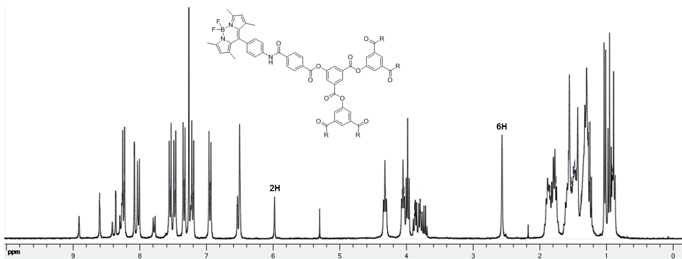
Figure 3. 20. RMN proton du composé 3.F dans CDCl 3 .
