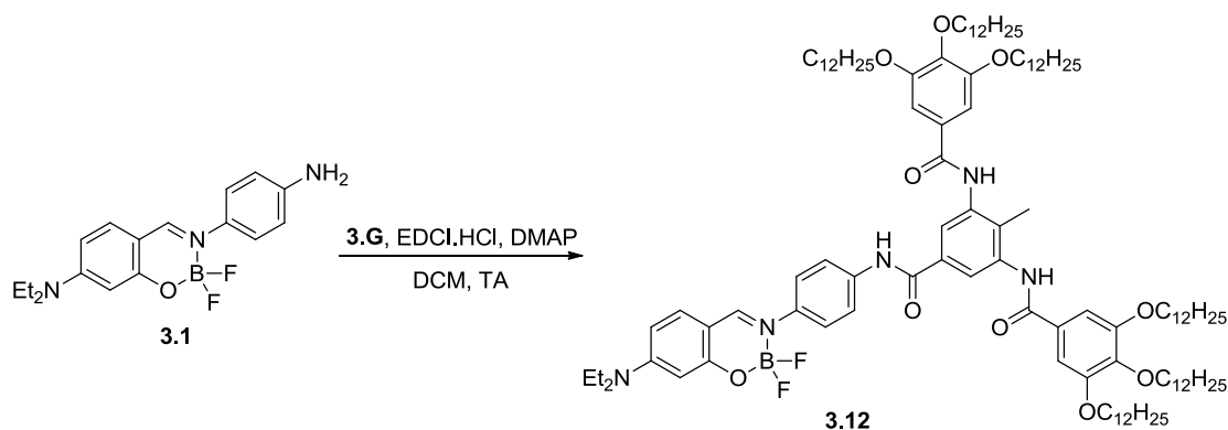
Figure 3.72. Boranil lié à la plateforme par couplage peptidique.
