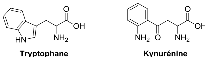
Figure 5. 3. L'acide aminé tryptophane et son métabolite, la kynurénine.
