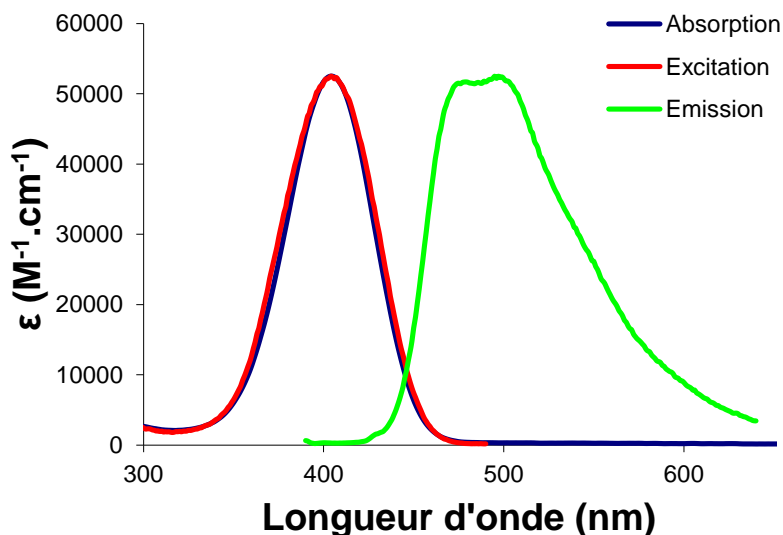
Figure 3. 49. Spectres d'absorption, d'émission ( \lambda_{ex} = 380 nm) et d'excitation ( \lambda_{em} = 520 nm) du Boranil 3.6 dans le dichlorométhane.
