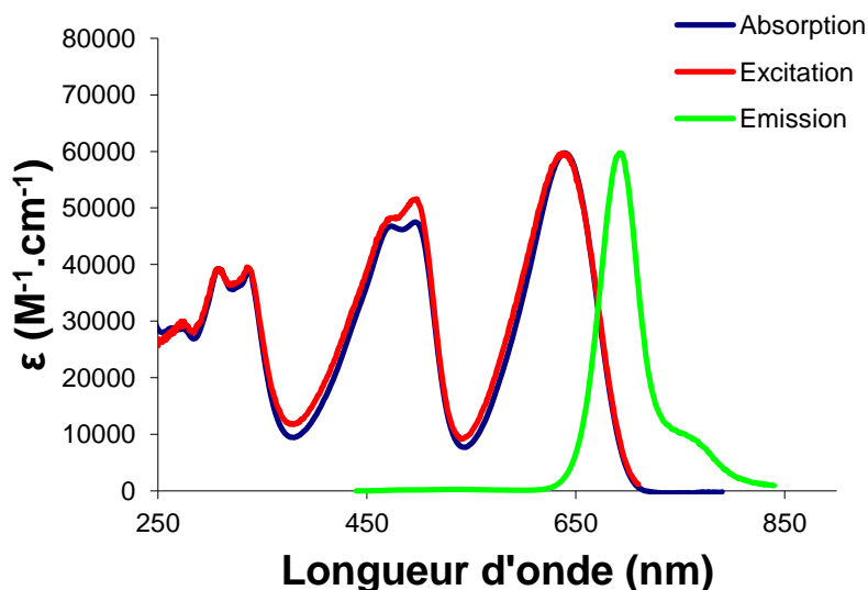
Figure 5. 24. Spectres d'absorption, d'émission ( \lambda_{\text{ex}} = 485 \text{ nm} ) et d'excitation ( \lambda_{\text{em}} = 750 \text{ nm} ) de la dyade Borico-BODIPY dans le dichlorométhane.
