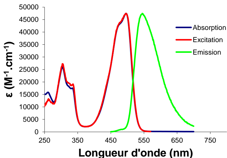
Figure 5. 13. Spectres d'absorption, d'émission ( \lambda_{ex} = 420 nm) et d'excitation ( \lambda_{em} = 600 nm) du Borico 5.2c dans le DCM.
