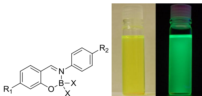
Figure 1. La famille des Boranils.
