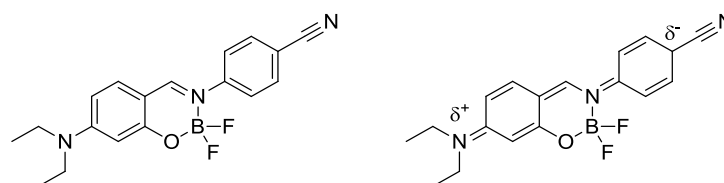
Figure 2. 22. Formes mésomères résonantes du Boranil 2.2e .
