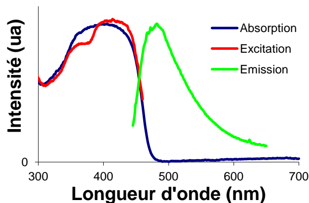
Figure 2. 27. Spectres d'absorption, d'émission ( \lambda_{\text{ex}} = 380 \text{ nm} ) et d'excitation ( \lambda_{\text{em}} = 510 \text{ nm} ) du Boranil 2.2d ( \text{Et}_2\text{N}/\text{I}/\text{F} ) à l'état solide.
