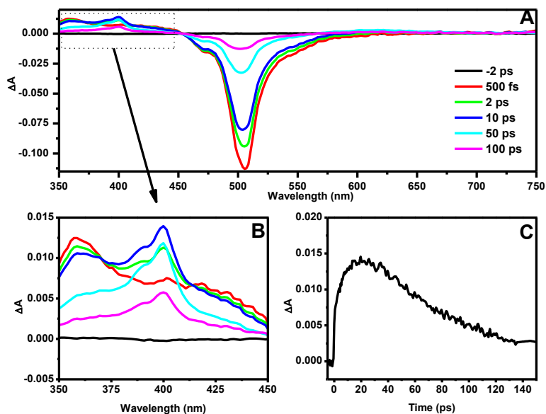
Figure 3. 10. Absorption transitoire du BODIPY 3B (excitation à 505 nm).
