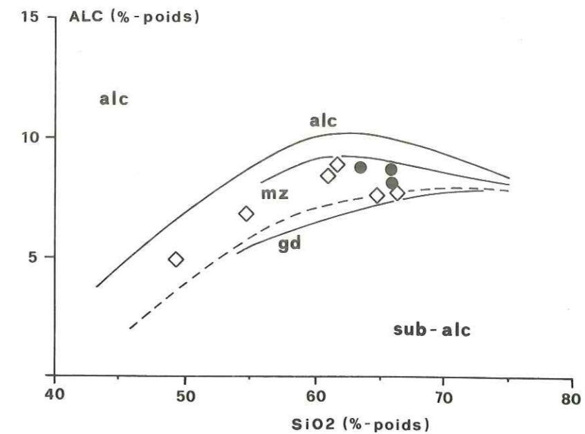
Fig. A3. Distribution des porphyres quartzifères de Plex-Aboyeu ● et des roches du volcanisme carbonifère supérieur du massif des Grandes Rousses ◇ (BANZET et al., 1985) dans le diagramme T(otal)-A(lkali)-S(ilica) de LAMEYRE (1987). ALC = \text{Na}_2\text{O} + \text{K}_2\text{O} ; alc - série alcaline; mz - série monzonitique; gd - série granodioritique; la ligne traitillée sépare les séries alcalines et subalcalines (sub-alc).
