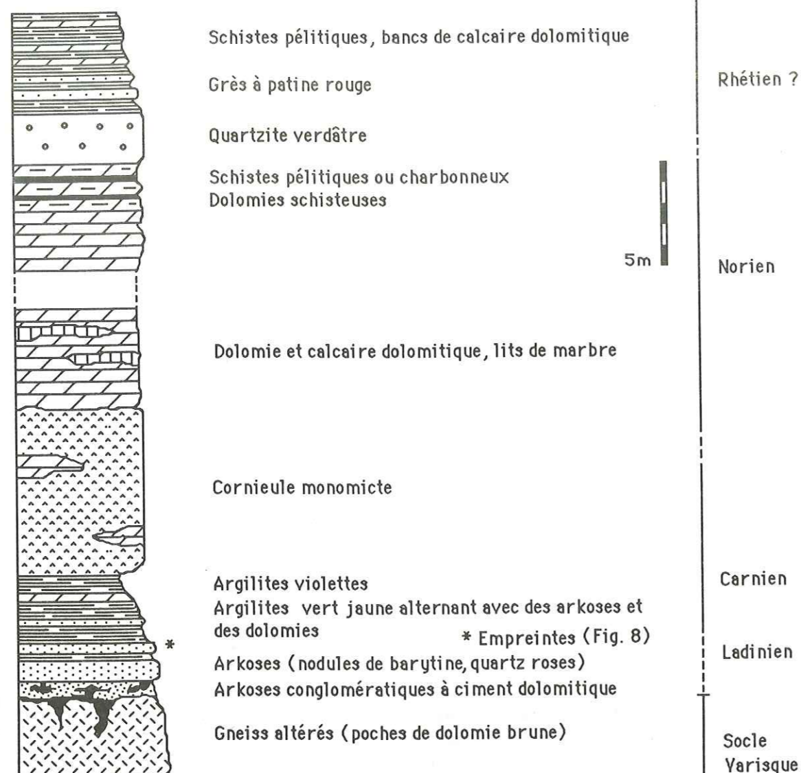
Fig. 7. Coupe stratigraphique schématique du Trias (les épaisseurs sont approximatives; elles correspondent à des niveaux déformés)
