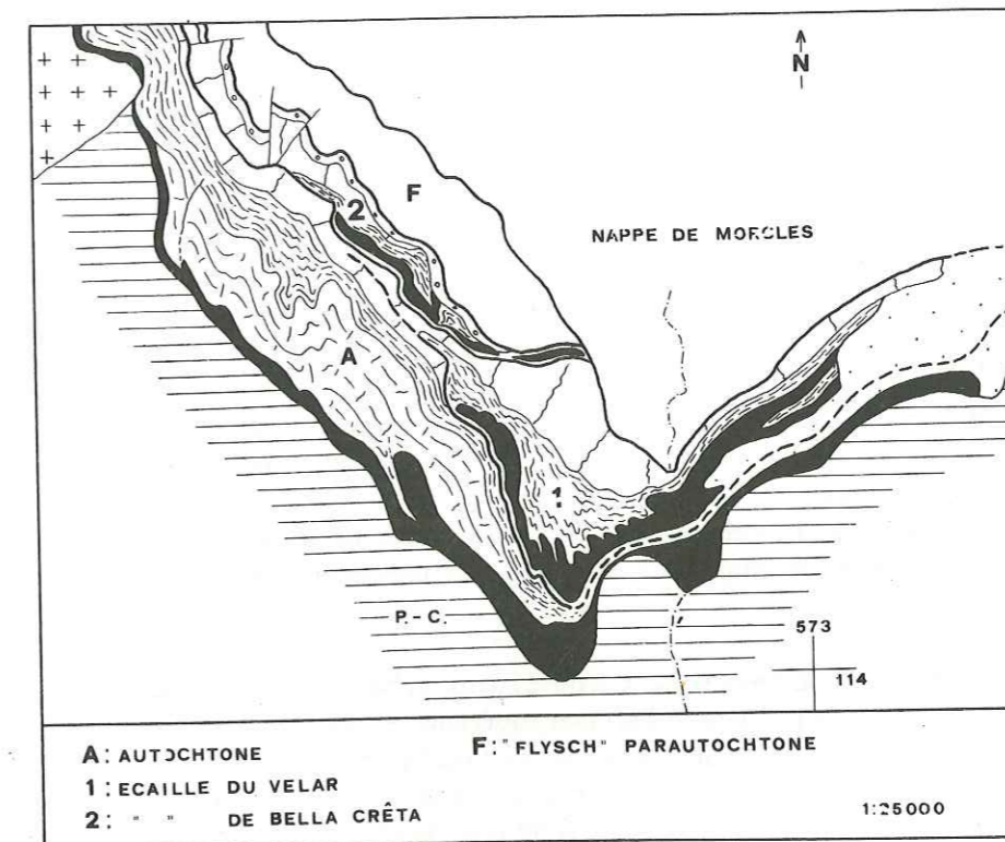
Fig. 13. Carte structurale des écaïlles parautochtones.
