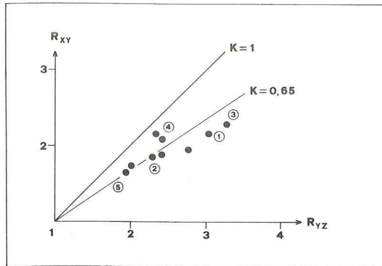
Fig. 27. Valeurs de l'ellipsoïde de la déformation mesurées sur des taches de réduction et reportées sur un diagramme de Flinn.
