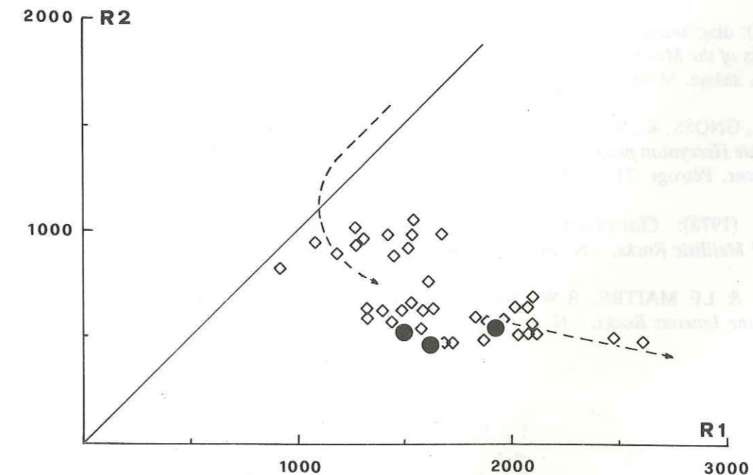
Fig. A4. Distribution des porphyres quartzifères de Plex-Aboyeu ● et des roches du volcanisme carbonifère supérieur du massif des Grandes Rousses ◇ (BANZET et al., 1985) dans le diagramme R_1(=4\text{Si}-11(\text{Na}+\text{K})-2(\text{Fe}+\text{Ti})) - R_2(=6\text{Ca}+2\text{Mg}+\text{Al}) de DE LA ROCHE & LETERRIER (1973).
