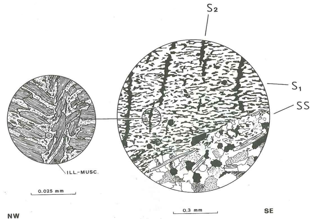
Fig. 44. Relations à l'échelle de la lame mince entre SS, S1 et S2 dans les grès du Trias. (Coordonnées: 573.600/112.400; voir fig. 43)
