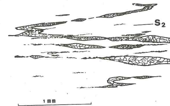
Fig. 18. Déformation D2 dans le calcaire permo-carbonifère du Sécheret.
