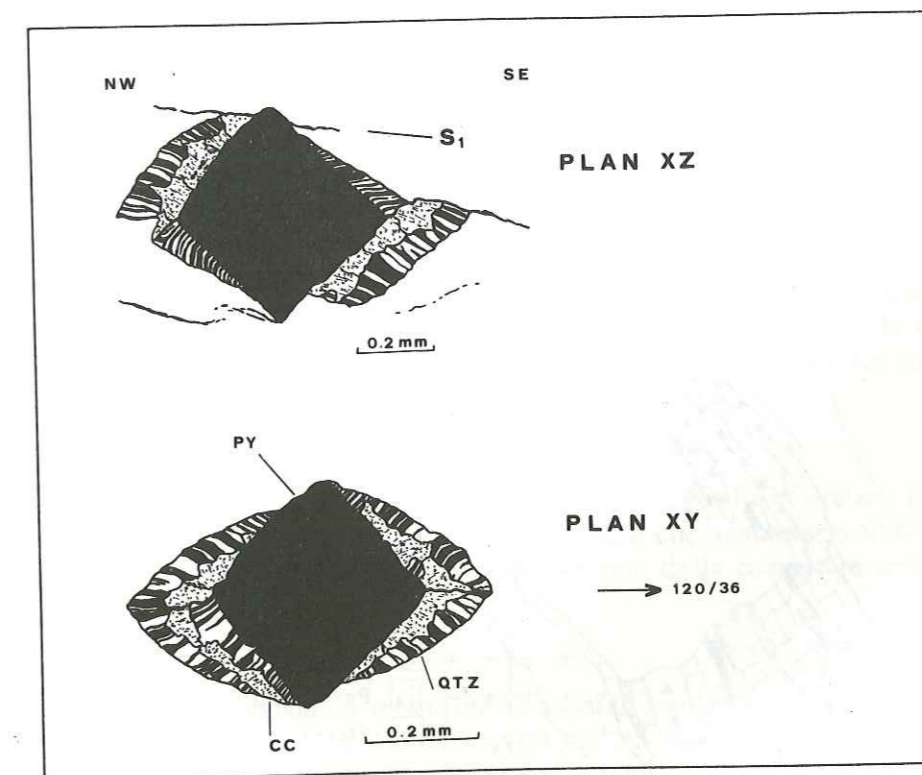
Fig. 41. Ombres de pression autour des cristaux de pyrite dans les dolomies du Trias. (Nant des Pesottes, 1640 m)
