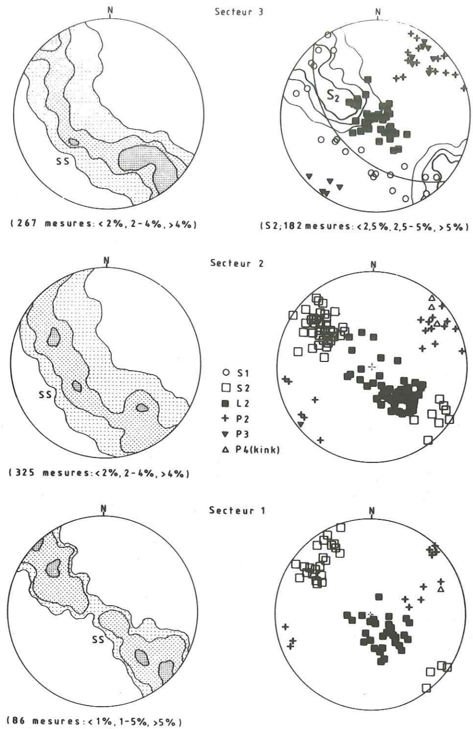
Fig. 15. Structures du Permo-Carbonifère. (Canevas de Lambert, hémisphère inférieur) (Secteurs voir page 24)
