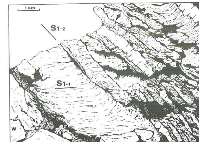
Fig. 40. Schistosité S1-1 , parallèle à SS , visible dans des microlithons de la schistosité S1-2 ; flanc normal d'un pli. (Nant de Luymène; coord: 571.450/114.950, 1720 m)
