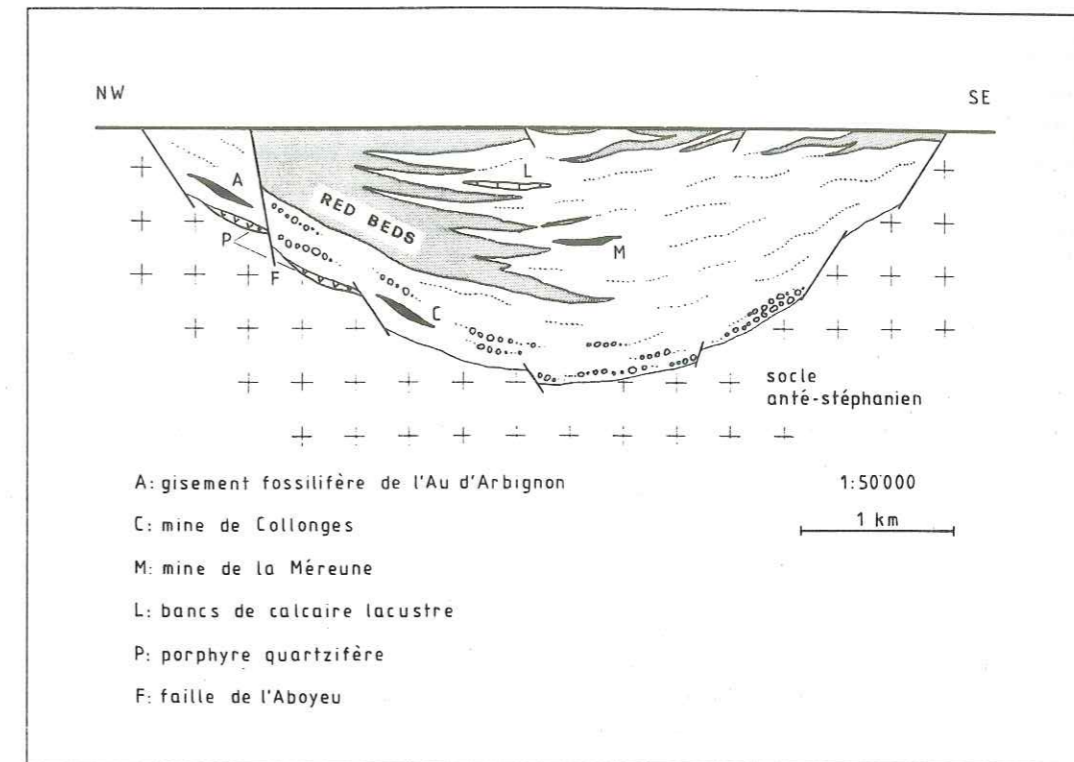
Fig. 2. Coupe schématique du bassin sédimentaire permo-carbonifère; reconstitution au Trias. (construction du bassin, voir page 28)
