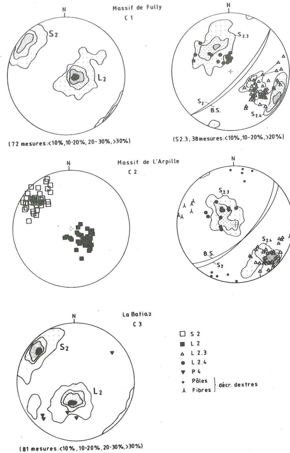
Fig. 35. Structures de la déformation alpine dans le socle. Localisation: voir fig. 39. (Canevas de Lambert, hémisphère inférieur)
