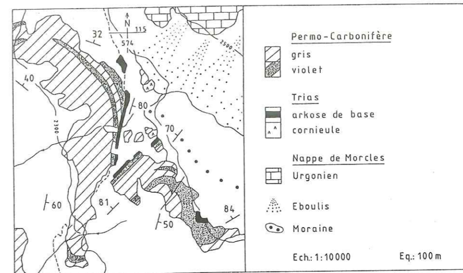
Fig. 12. Carte géologique du synclinal de Fenestral
