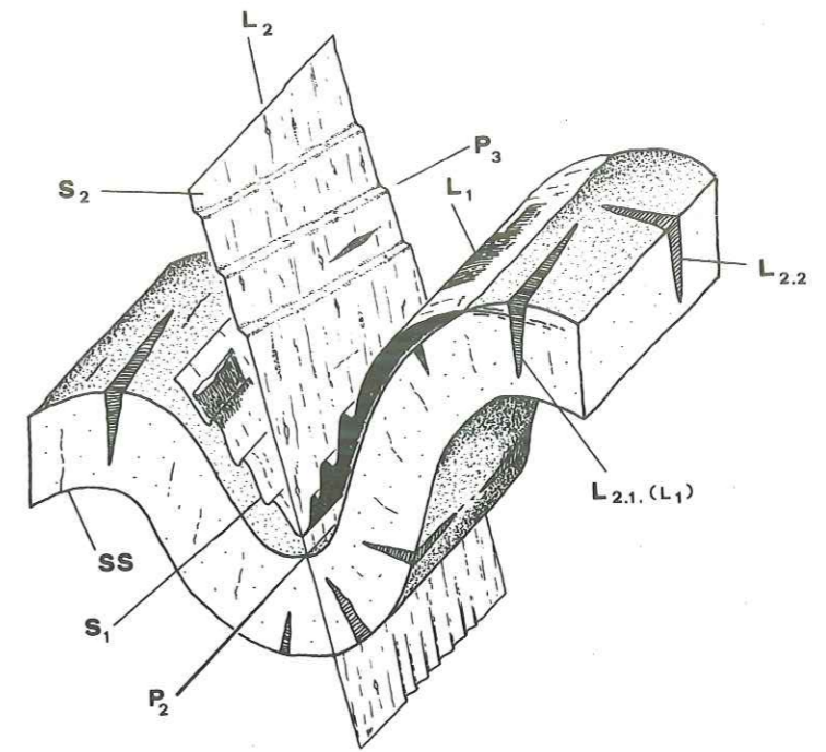
Fig. 16. Structures du Permo-Carbonifère (explications dans le texte) La Maraiche (coord. 573.500/113.650).
