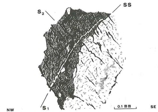
Fig. 17. Relations entre SS, S1 et S2; anticlinal de Lui Crève.
