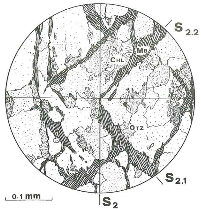
Fig. 19. Clivages conjugués S2.1 et S2.2 dans les microgrès. L2 est vertical. (Mb= séricite, Chl= chlorite, Qtz= quartz)
