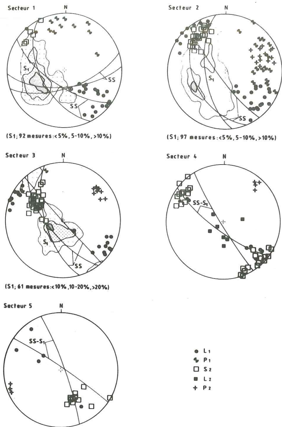
Fig. 45. Structures de la déformation dans la couverture autochtone et l'échelle du Vélard. (Canevas de Lambert, hémisphère inf.) Explications dans le texte Secteur 1: L'Au d'Arbignon-coord. 571.800 Secteur 2: Coord. 571.800-arête S du Six Tremble Secteur 3: Arête S du Six Tremble-coord. 573.400 Secteur 4: Flanc W du Grand Chavalard Secteur 5: Région de la Tête du Portail
