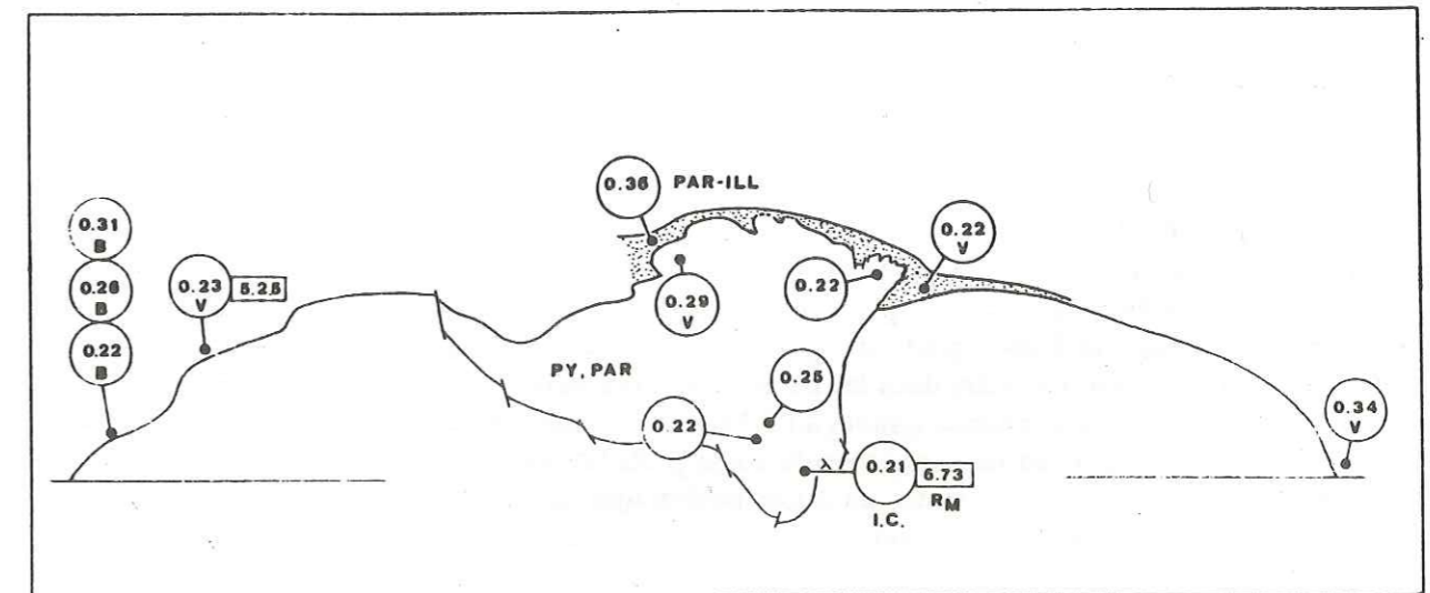
Fig. 51. Valeurs de la réflectance de la vitrinite R_{\max} (d'après KUBLER et al., 1979) et de la cristallinité de l'illite I.C., dans le synclinal de Dorénaz et la couverture mésozoïque autochtone (v=pélites vertes; B= d'après BURKHARD, 1988).
