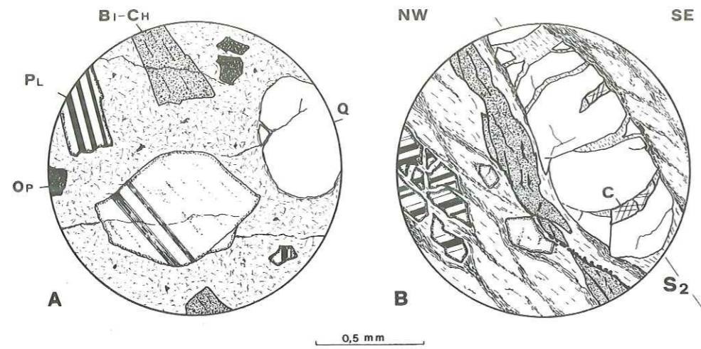
Fig. 37. Aspects de la déformation dans les niveaux de porphyre quartzifère. A) Sud de Plex B) Torrent de l'Aboyeu (Bi-Ch= biotite chloritisée, Q= quartz, Pl= plagioclase, Op= opaques, C= calcite; matrice indéterminable). (voir description page précédente)
