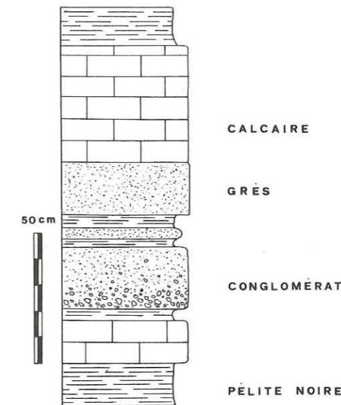
Fig. 3. Coupe stratigraphique des bancs de calcaire lacustre. Grand Couloir (coord: 571.250/113.275, 2050 m)
