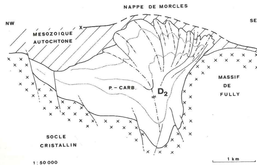
Fig. 11. Schéma structural du synclinal de Permo-Carbonifère de Dorénaz.
