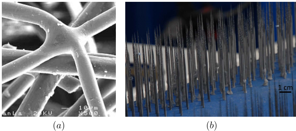
Figure I.9 – Contact entre fibres fusibles observé au MEB sur une laine de chanvre [Collet 2004] (a), et aiguilles utilisées dans les chaînes de fabrication par aiguietage (b)
