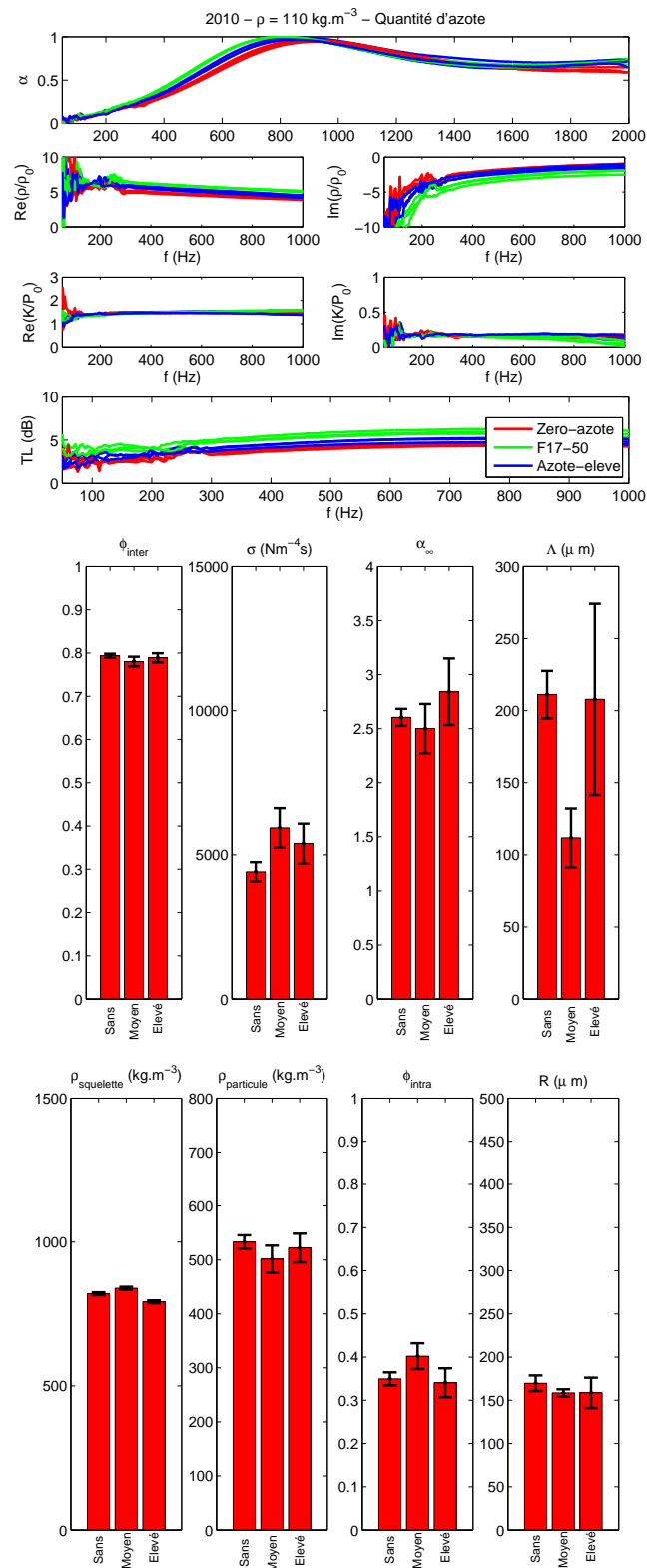
Figure E.21 – Propriétés acoustiques des chênevottes en fonction de la quantité d'azote
