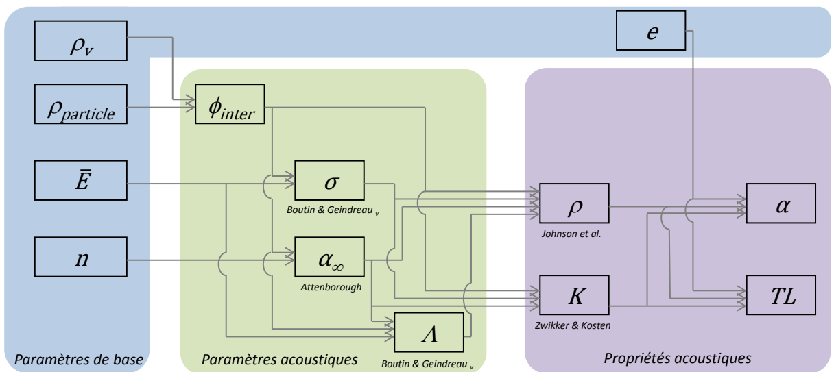
Figure IV.16 – Diagramme pr sentant le processus de mod lisation des ch nevottes
