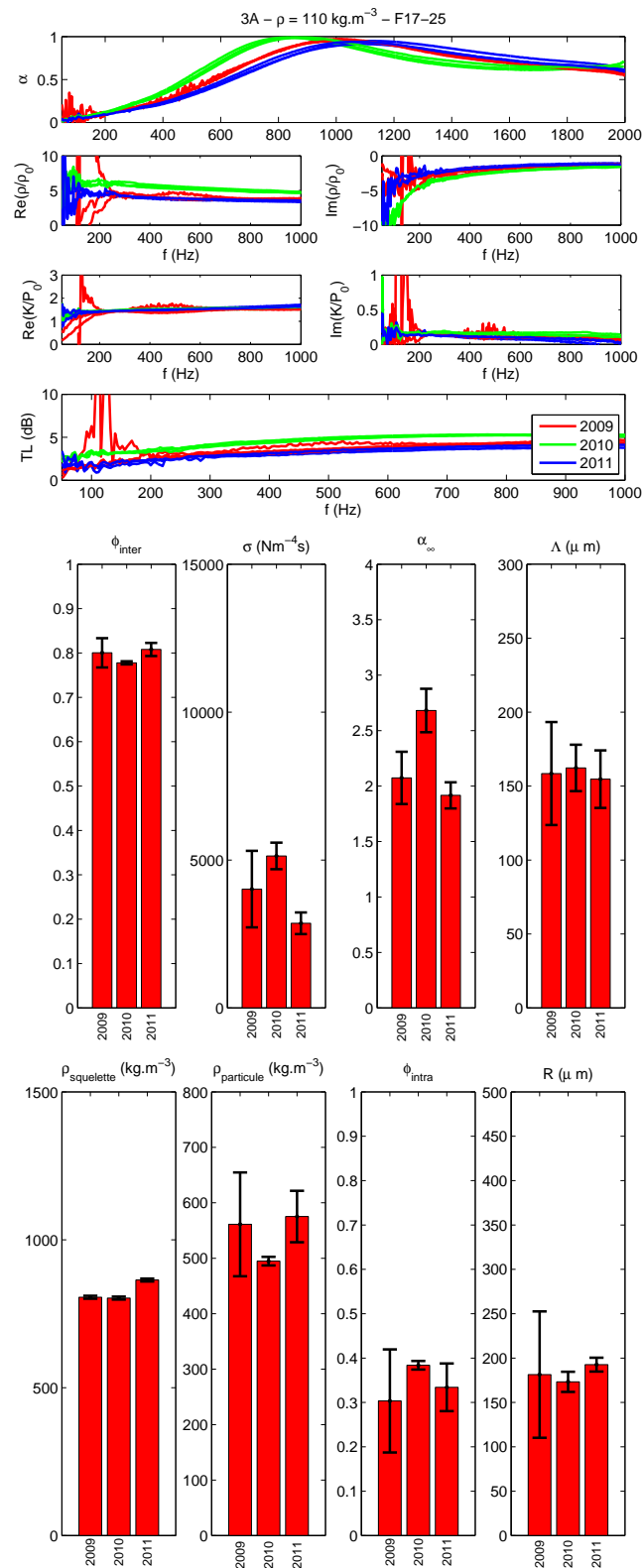
Figure E.27 – Propriétés acoustiques des chènecottes en fonction de l'année - F17-25
