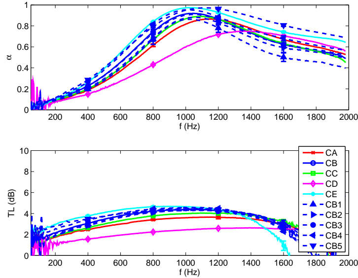
Figure II.13 – Propriétés acoustiques des chènevottes pour \rho_v = 120kg.m^{-3}
