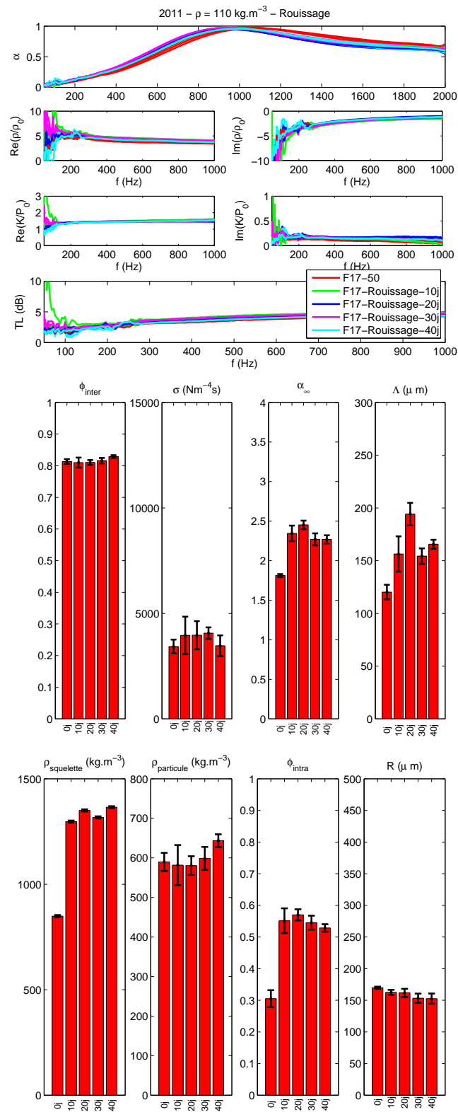
Figure E.26 – Propriétés acoustiques des chènervottes en fonction du rouissage
