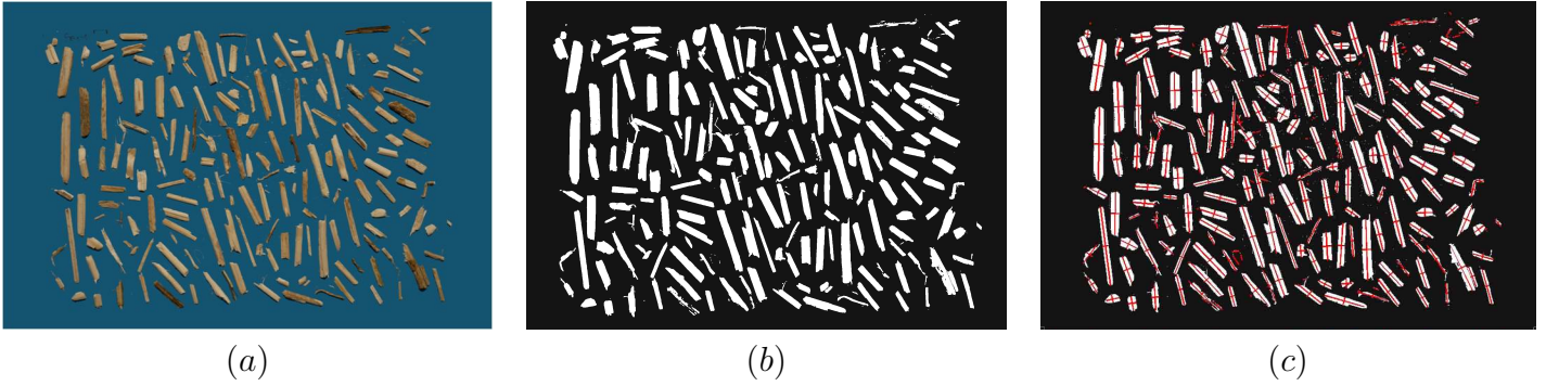
Figure II.4 – Caractérisation de la granulométrie des chènevottes avec image initiale (a), image convertie en noir et blanc (b) et détermination des longueur et largeur de chaque particule (c)
