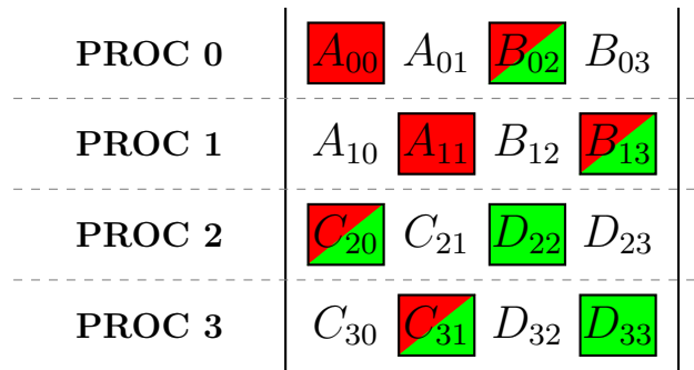
FIGURE 7.9 – Structure de la matrice éléments finis standards pour un espace de fonction produit (II).
