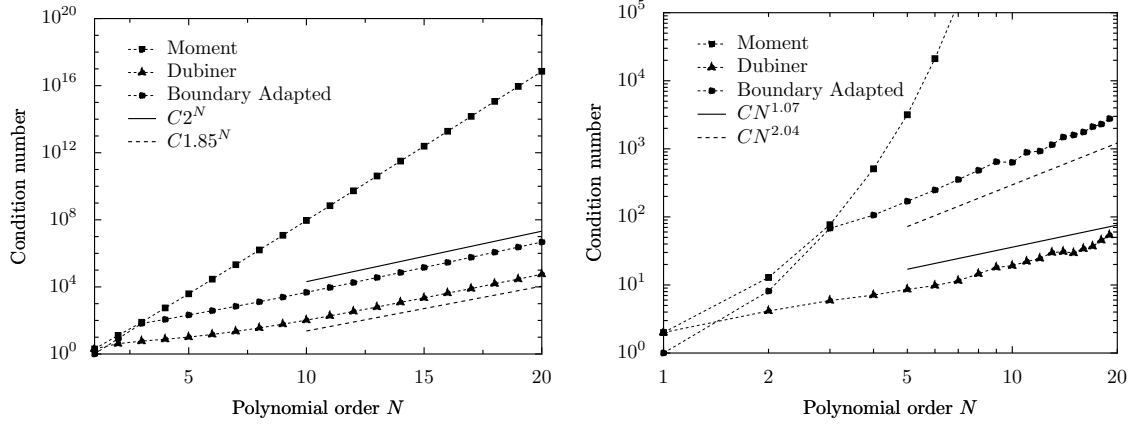
(a) Conditionnement de V(\mathcal{B}, X) pour les points équirépartis (b) Conditionnement de V(\mathcal{B}, X) pour les points de Fekete
