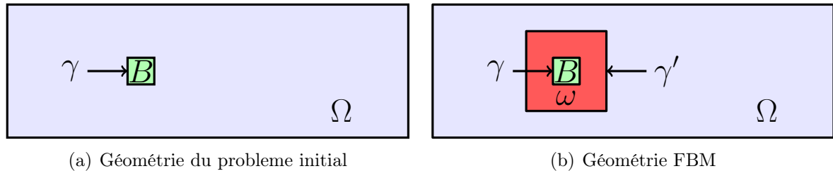
FIGURE 3.18 – Géométries utilisées dans l'application 2
