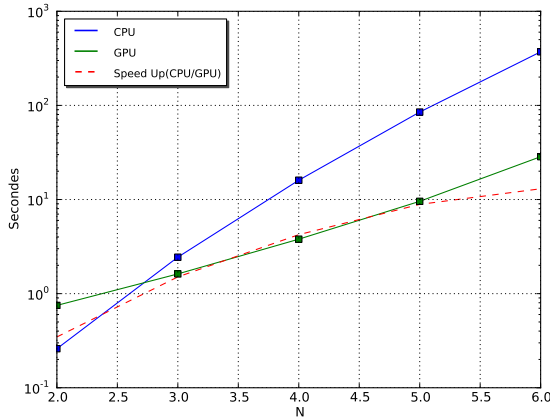
FIGURE 7.23 – Temps d'assemblage en 3D (masse+raideur) en fonction de l'ordre polynomial N avec N_{elt} = 10000 et \mathbf{dimBloc} = 6 .
