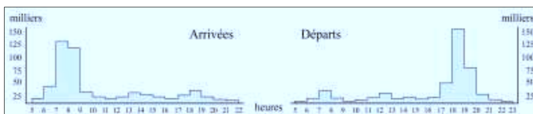
figure 6 : Trafic quotidien des gares parisiennes au début des années 80
