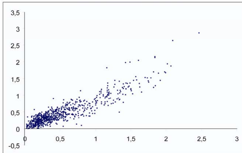
Figure 37 : Validation du modèle A_{visi} par le croisement des flux prédicts avec les flux observés
