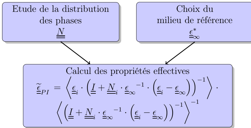
FIGURE 2.7 – Démarche des méthodes d'homogénéisation basées sur des problèmes d'inclusion.
