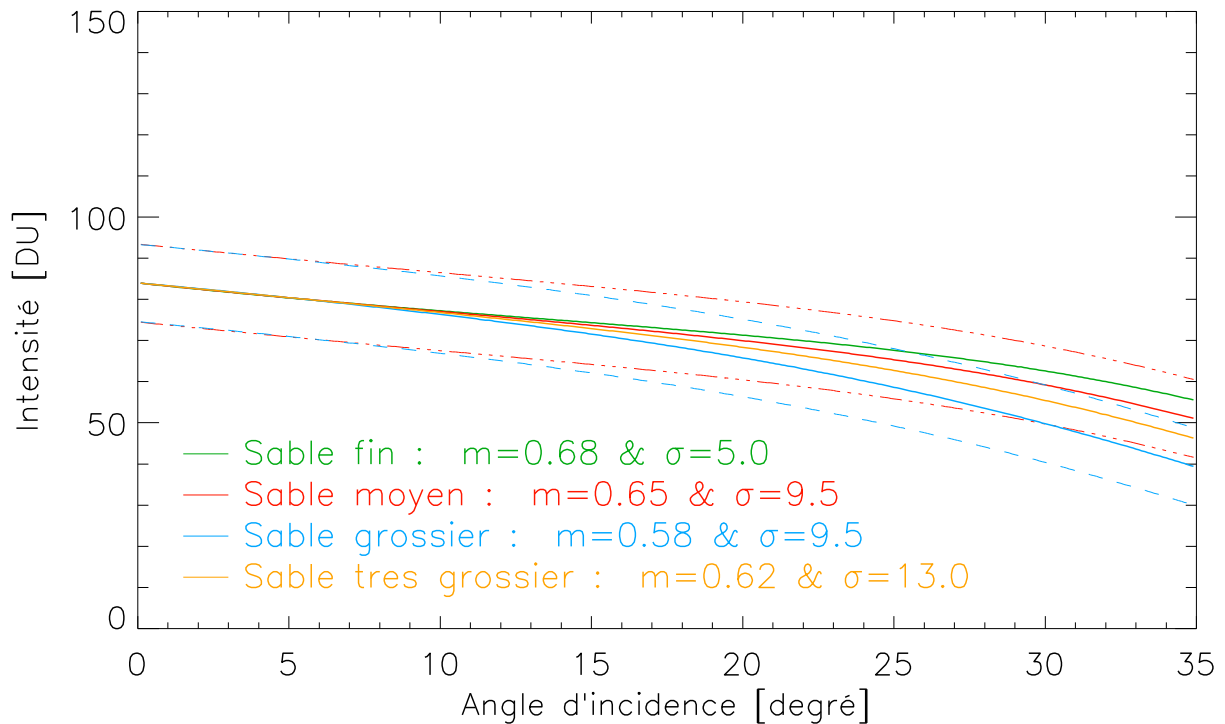
Figure IV.17 : Régression numérique des données à partir du modèle de distribution de microfacettes. Pour plus de visibilité, comme les échantillonnages statistiques des sables fins et très grossiers sont très faibles, seuls les écart-types des sables moyens et grossiers sont représentés (en pointillé)
