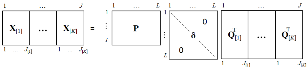
FIGURE 2.1 – SVD sur une matrice \mathbf{X} structurée par blocs.
