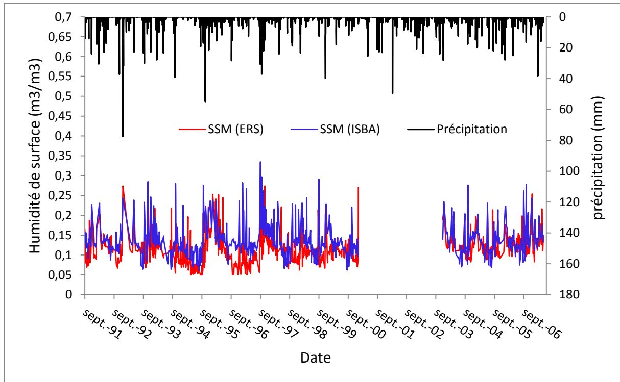
Figure V.8 : Inter-comparaison entre les sorties d'humidité de surface ISBA-A-gs et ERS
