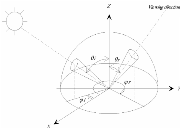
Figure I.4: Géométrie de mesure de la réflectance (GDTA 1991).
