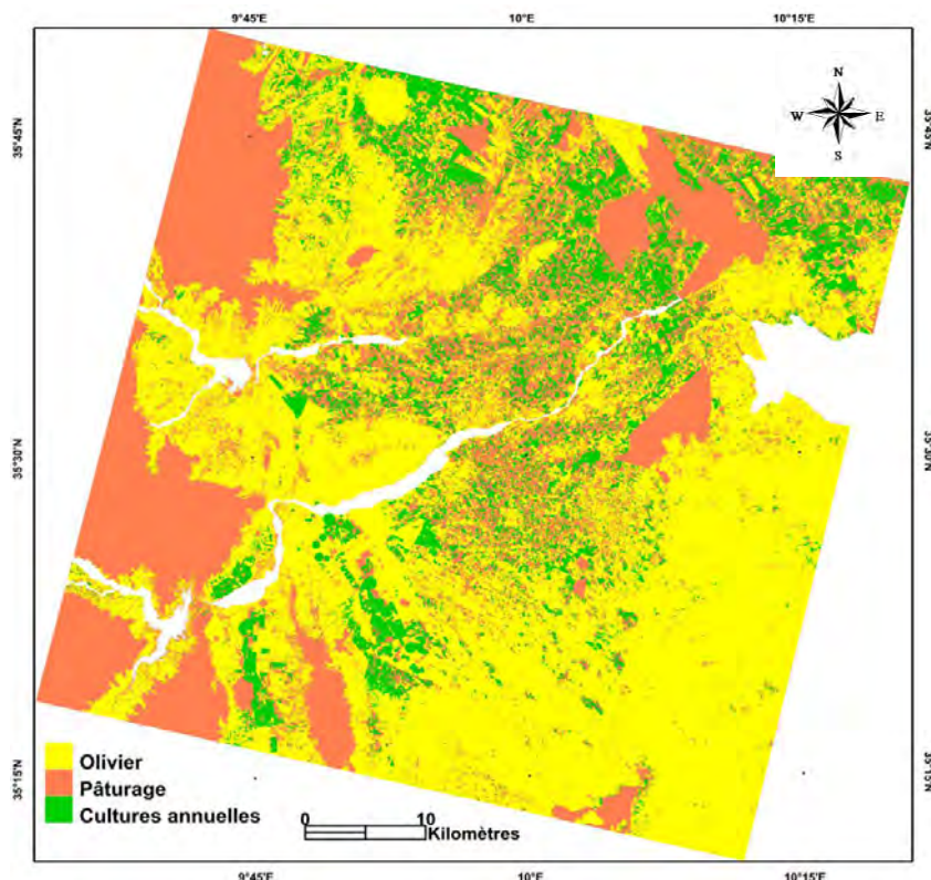
Figure II.17 : Occupation du sol établie à partir des données SPOT HR (saison agricole 2008-2009) Pour les deux autres classes Oliviers et pâturages, les restitutions sont moins bonnes, le RMSE peut atteindre 40%. On signale que les performances de la méthode de désagrégation varient sensiblement d'une classe à l'autre. En particulier, les pourcentages de la classe « pâturages » restitués à haute et basse résolution spatiale apparaissent nettement moins corrélés que ceux de la culture annuelle. L'explication tient pour partie à la forte hétérogénéité de cette classe (taille et densité de la végétation qui change d'une saison à une autre).
