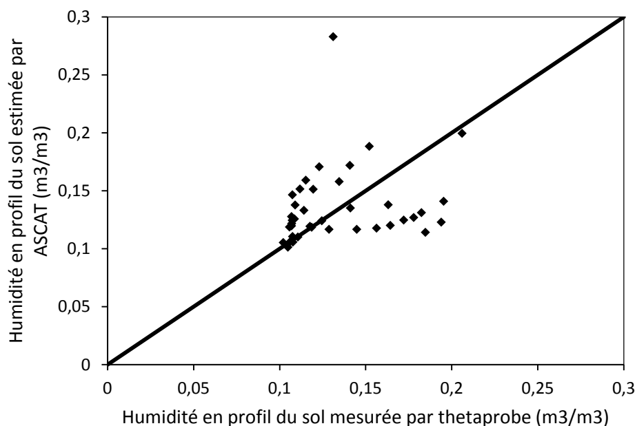
Figure IV.5.b : inter-comparaison entre les humidités du sol de la zone racinaire estimées par ASCAT et ceux de mesures in situ
