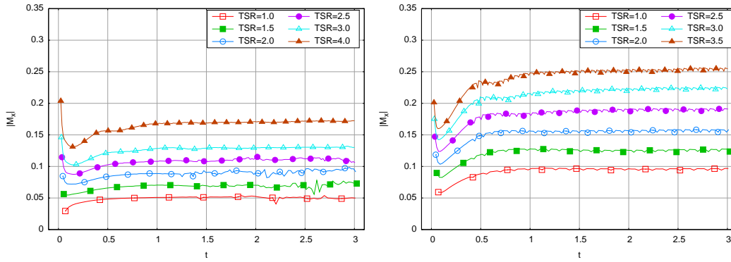
(a) Configuration BBMC avec un angle de calage de 5^\circ
