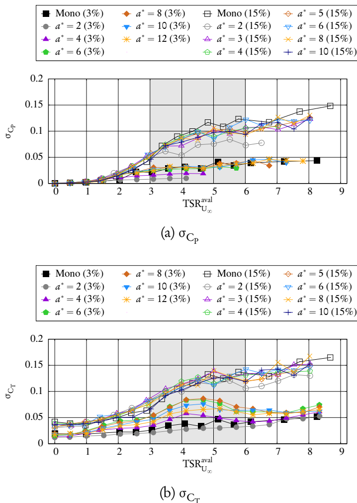
FIGURE 1.17 – Écart-types de C_{P,U_\infty}^{\text{aval}} et de C_{T,U_\infty}^{\text{aval}} , en fonction du \text{TSR}_{U_\infty}^{\text{aval}} de l'hydrolienne aval, avec \text{TSR}^{\text{amont}} = 4 , U_\infty = 0,8 \text{ m} \cdot \text{s}^{-1} pour I_\infty = 3\% et U_\infty = 0,83 \text{ m} \cdot \text{s}^{-1} pour I_\infty = 15\% . Ces écart-types sont comparés à ceux d'une seule hydrolienne, à I_\infty = 3\% et I_\infty = 15\% respectivement.
