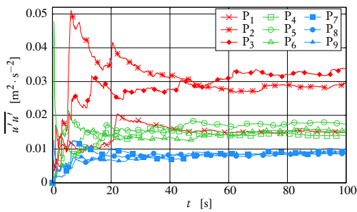
(c) Première contrainte normale de Reynolds \overline{u'u'} = \sigma_u^2
