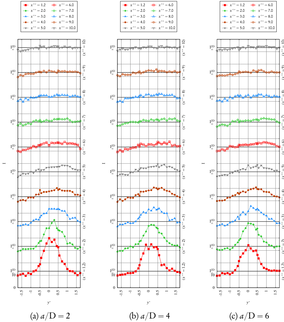
FIGURE A.13 – Profils de taux de turbulence aval \text{TSR}^{\text{amont}} = \text{TSR}^{\text{aval}} = 3,67 , U_\infty = 0,83 \text{ m} \cdot \text{s}^{-1} , I_\infty = 15\% et avec différentes distances inter-hydroliennes, à savoir a^* = 2 , a^* = 4 et a^* = 6 .
