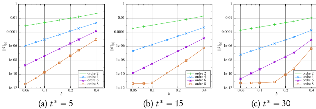
FIGURE 5.9 – Erreur L_2 sur la concentration \|\mathcal{E}\|_{[c]} à t^* = 5 (à gauche), t^* = 15 (au centre) and t^* = 30 (à droite) en fonction de la discrétisation spatiale h pour différents ordres r d'approximation (voir le tableau 5.1), avec \kappa = 2 et les paramètres du tableau 5.3.
