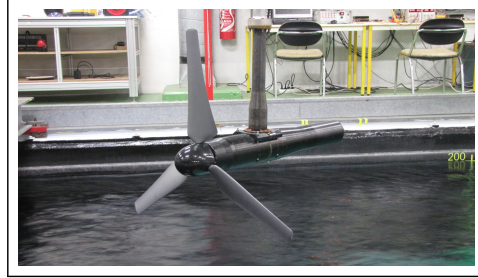
(b) Photographie du prototype
