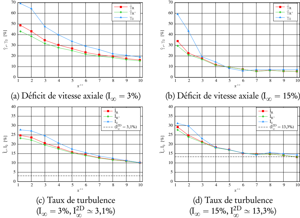
FIGURE 1.21 – Évolution du déficit de vitesse axiale et taux de turbulence dans le sillage de l’hydrolienne aval avec a^* = 4 , \text{TSR}^{\text{amont}} = \text{TSR}_{U_\infty}^{\text{aval}} = 3,67 et avec I_\infty = 3\% (à gauche) et 15\% (à droite).
