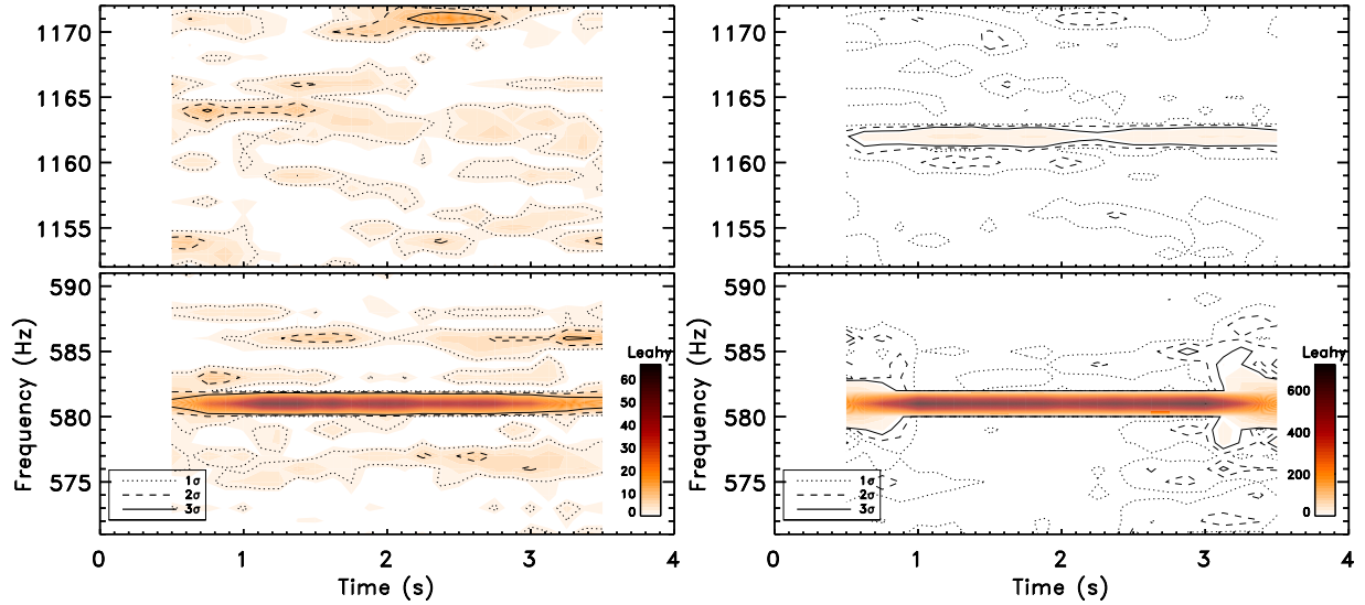
FIGURE 5.4 – Spectres de puissance dynamique et recherche de la fréquences fondamentale et de la première harmonique pour les instruments PCA (gauche) et LOFT (droite). Les contours de détection du signal à 1, 2 et 3 \sigma sont représentés. La valeur de la puissance de Leahy augmente avec la couleur foncée.
