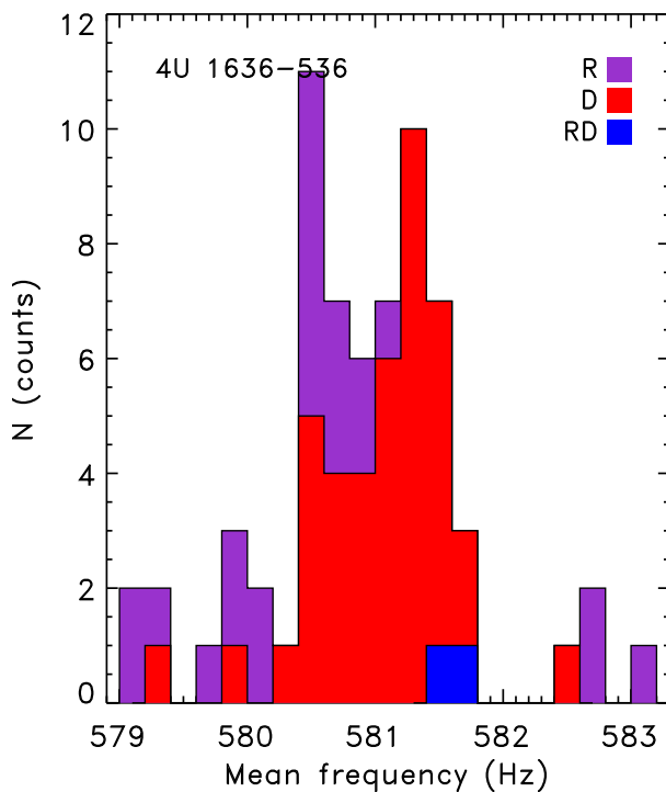
FIGURE 2.9 – Histogramme de répartition des fréquences. On distingue sur ces histogrammes les signaux localisés dans la phase de croissance ( R ) du sursaut, ceux de la phase de décroissance ( D ) et ceux qui s'étalent sur les deux phases ( RD ). Le test de Kolmogorov-Smirnov entre les distributions des fréquences de la phase de croissance ( R ) et de décroissance ( D ) donne une statistique égale à 0.47, soit une probabilité qu'elles soient distinctes égale à 99.8%.
