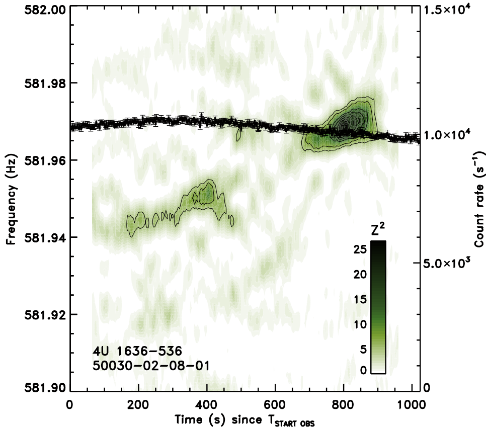
FIGURE 2.12 – Représentation des iso-contours du test de signification statistique ( Z_1^2 ) pour l'étude de la courbe de lumière du super-sursaut de 4U 1636–536. J'ai utilisé une fenêtre glissante d'une durée de 128 s et un pas de 4 s. On observe deux trains d'oscillations disjoints significatifs et une dérive fréquentielle totale de \sim 0.025 Hz ( < 0.005\% ) autour de 591.96 Hz.
