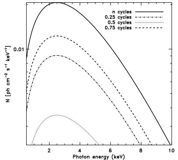
FIGURE 3.6 – Spectre observé de densité d'énergie de l'émission sous l'effet d'une atmosphère diffusante à différents états du cycle de rotation (1/4, 1/2, 3/4 de cycle, ou un cycle entier). La température de la tache est fixée à 2 keV
