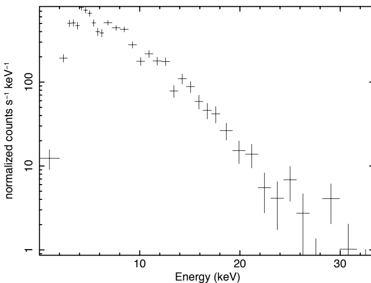
FIGURE 2.3 – Spectre en énergie calculé pendant la présence des oscillations du sursaut X de 4U 1702-429. Il montre que le signal est concentré dans la bande d'énergie 2-22 keV.
