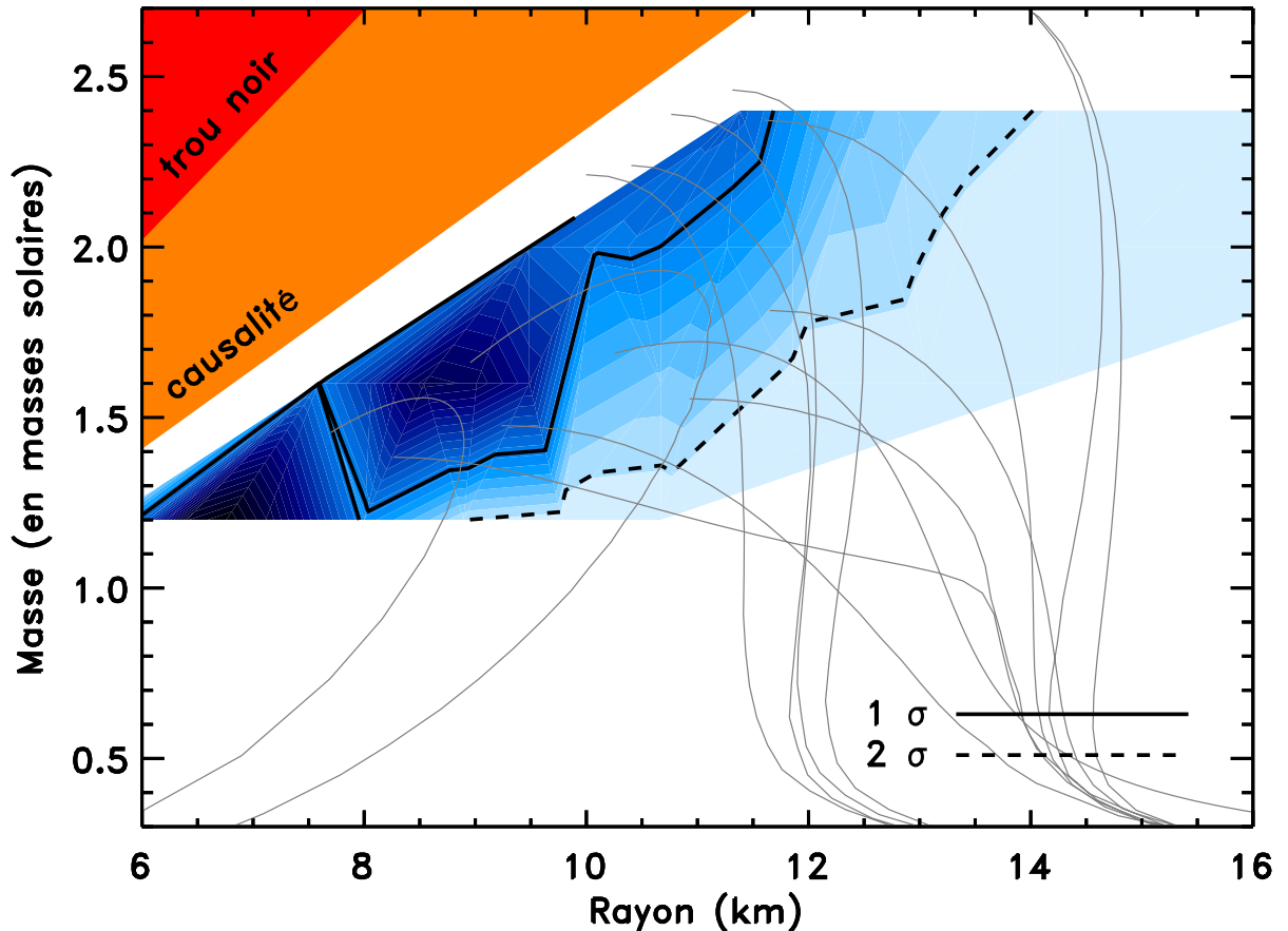
FIGURE 4.8 – Contraintes permises par l'ajustement conjoint des 5 trains d'oscillations de l'échantillon de 4U 1636–536 dans le diagramme M-R. Les contours de confiance à 1 \sigma (68.3%) et 2 \sigma (95.45%) sont dessinés et les couleurs définissent la valeur du test de Cash (probabilité croissante vers le teint foncé).
