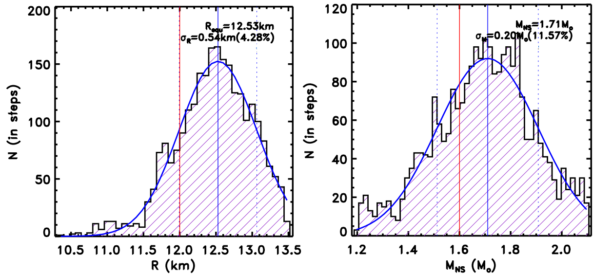
FIGURE 5.6 – Fonctions de densité de probabilité de la masse et du rayon issues de l'ajustement avec la statistique permise par LOFT . Les distributions sont ajustées par une gaussienne afin d'obtenir la valeur moyenne et une incertitude à 1\sigma .
