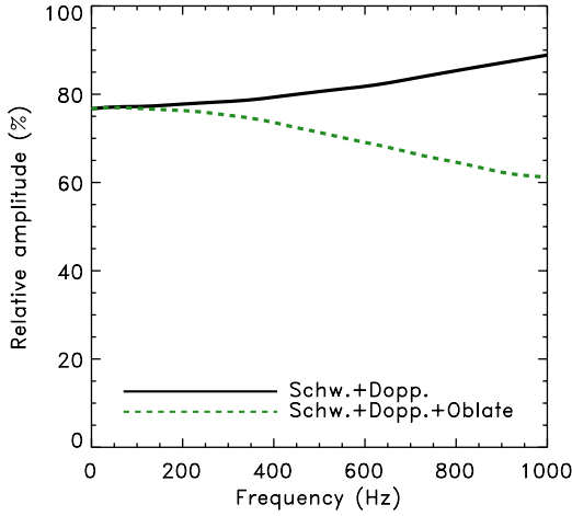
FIGURE 3.8 – Evolution de l'amplitude relative des oscillations en fonction de la fréquence de rotation d'une étoile sphérique ou ellipsoïdale.
