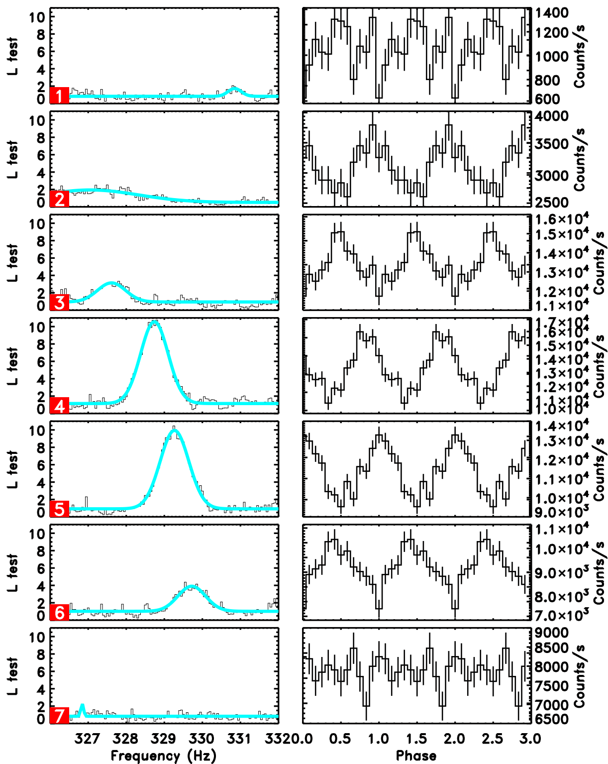
FIGURE 2.8 – Evolution dynamique de la signification statistique. A gauche sont présentées les valeurs de la statistique L associées aux fréquences testées dans le voisinage de 329 Hz, pour chaque intervalle considéré. Pour affiner les résultats, j'ajuste en plus ces valeurs par une distribution gaussienne et je considère que son centroïde est la fréquence la plus probable. A droite, on présente les profils moyens d'oscillations (sur 12 bins) correspondant à ces segments.
