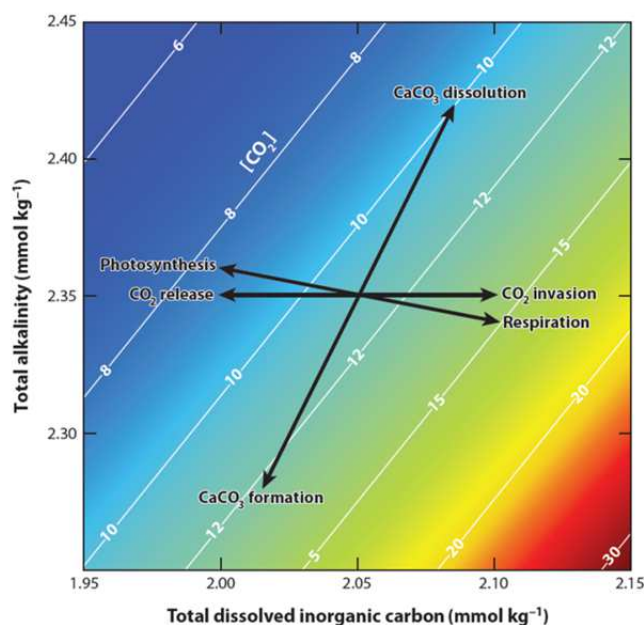
Figure 0-3: Effets de différents processus sur les paramètres CID (total dissolved inorganic carbon) , A_T (total alkalinity), et [\text{CO}_2] de la chimie des carbonates. Sous conditions fixes, température: 15^\circ\text{C} ; salinité : 35 et pression : 1 atm. Issu de Zeebe 2011.
