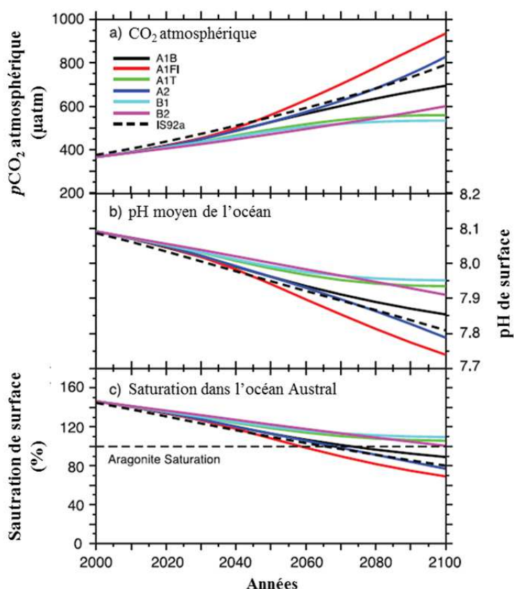
Figure 0-5: Changements de la pCO 2 atmosphérique, du pH moyen à la surface des océans et de l'état de saturation de l'aragonite de l'océan Austral, en fonction des 6 scénarios définis par le SRES (de A1B à B2). Séries temporelles pour a) la pCO 2 atmosphérique ; b) le pH moyen de l'océan de surface ; c) l'état de saturation en aragonite moyen dans l'océan Austral (Plattner et al. 2001). IS92a : scénario antérieur au SRES. D'après Solomon et al. 2007.
