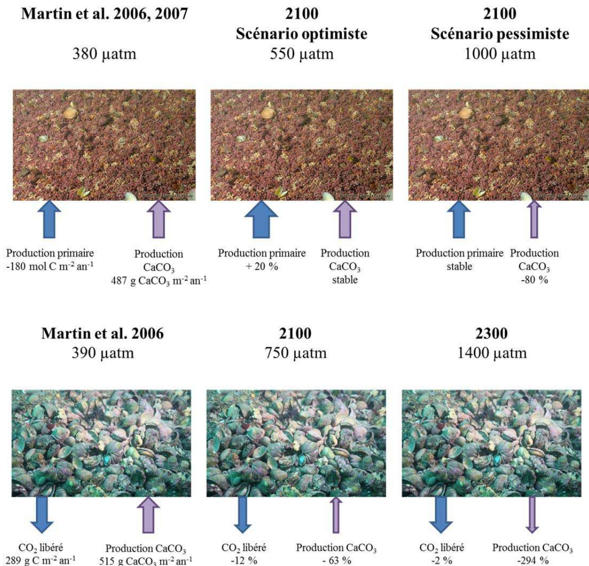
Figure D-11: Flux de carbone (C) et carbonate (CaCO 3 ) des populations de maërl et crépidules mesurés in situ sous des conditions actuelles de pCO 2 (Martin et al. 2006a; Martin et al. 2006b; Martin et al. 2007a) et extrapolées à partir des mesures faites durant cette thèse pour des conditions de pCO 2 prévues pour la fin du siècle. Les flèches bleues représentent les flux de CO 2 assimilé ou libéré par les processus de photosynthèse et de respiration alors que les flèches violette traduisent les flux de CaCO 3 induits par les processus de précipitation et de dissolution. La largeur des flèches est proportionnelle à l'intensité des flux.
