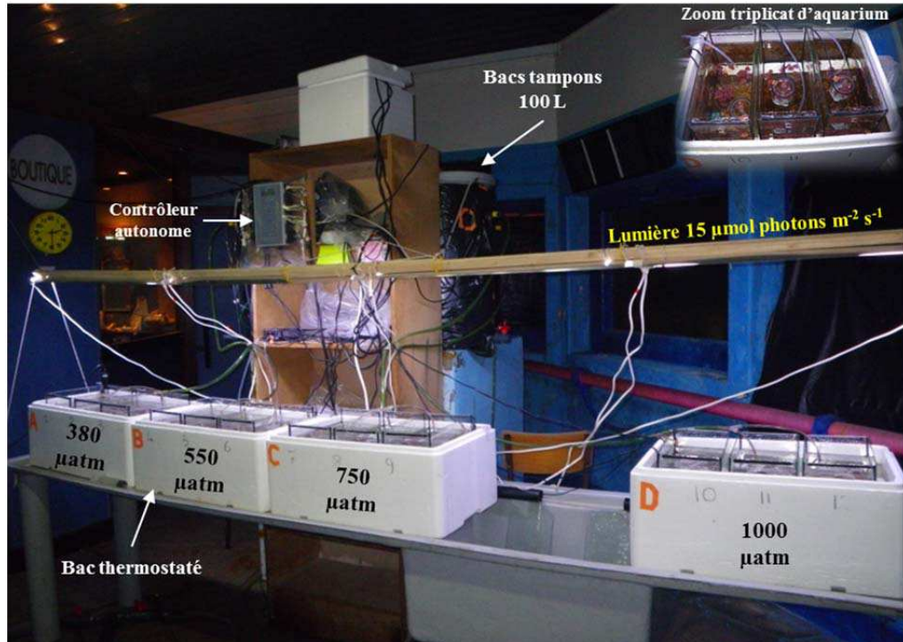
Figure I2-7: Montage expérimental de l'expérience sur le maërl. L'eau régulée au pH requis dans des bacs tampons de 100 L alimentait par gravité un triplicat d'aquariums maintenus dans des bacs thermostatés. La température et l'ajout de CO 2 étaient gérés par un contrôleur autonome IKS (Aquastar, Karlsbad, Allemagne).
