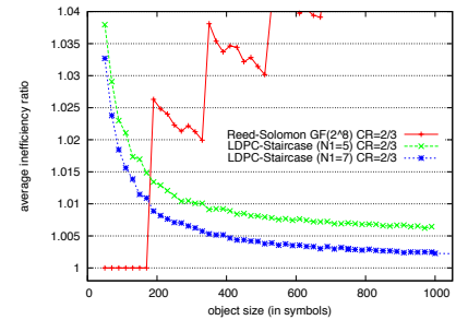
Figure 5.3: Capacités de correction des codes LDPC-Staircase ( ML ) et Reed-Solomon, avec ( k = 1024 , CR = 2/3 , G = 1 ).
