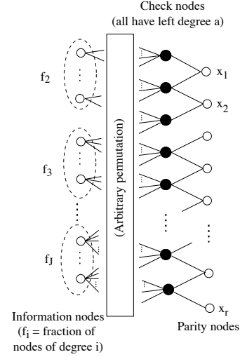
Figure 4.8: Graphe de Tanner d'un code IRA, extraite de [36].
