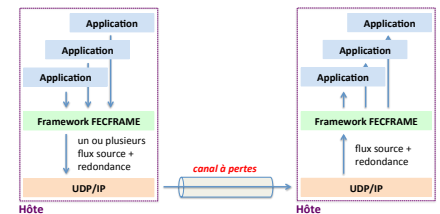
Figure 11.2: Déploiement de FECFRAME dans l'hôte.
