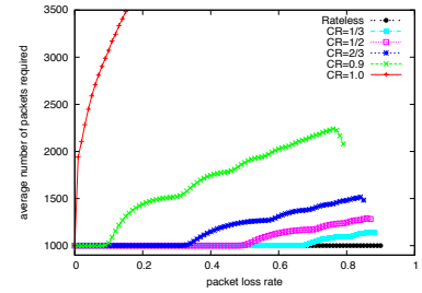
Figure 3.2: Impacts du code rate sur le nombre moyen de paquets nécessaires au décodage en mode carrousel.
