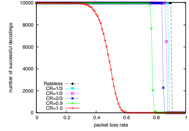
Figure 3.1: Impacts du code rate sur les performances des transmissions en mode carrousel.
