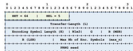
Figure 8.2: Format binaire du FEC OTI du RFC 5170. Le champ Header Extension Type (HET) indique une extension d'en-tête ALC/LCT de type EXT_FTI, tandis que le champ Length (HEL) donne sa longueur, ici 5 mots de 32-bits.
