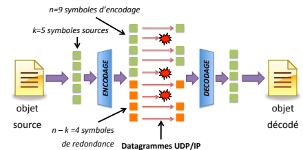
Figure 2.3: Principes de fonctionnement d'un code AL-FEC lors d'une transmission de datagramme UDP/IP sur Internet.
