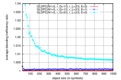
Figure 7.7: Capacités de correction moyennes des codes GLDPC-Staircase (cas où E = 0 , N_1 = 5 et non 7, bleu clair) et GLDPC-Staircase avec E = 1 ( r_G = 1/2 ) et E = 3 ( r_G = 1/3 ).
