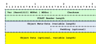
Figure 10.7: Objet composite et en-tête FCAST .
