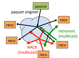
Figure 10.1: Mécanisme de retransmission avec SRM.
