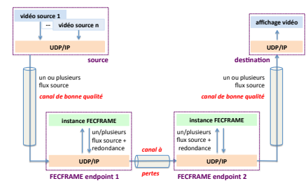
Figure 11.3: Déploiement de FECFRAME dans un équipement intermédiaire.
