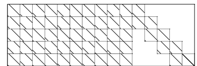
Figure 7.1: Matrice de parité d'un code QC-LDPC-Staircase (le bloc en bas à droite est une matrice escalière).
