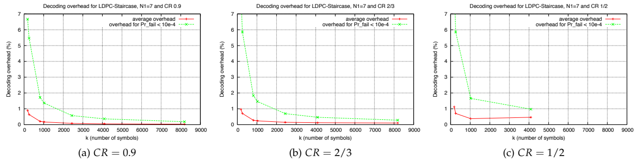
Figure 5.2: Capacités de correction des codes LDPC-Staircase en décodage ML, en fonction de CR, avec N_1 = 7 et G = 1 .
