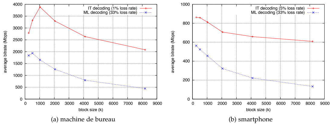
Figure 6.4: Vitesse du codec LDPC-Staircase, en décodage IT (bon canal) et ML (mauvais canal) ( CR = 2/3 , N_1 = 7 , symboles de 1024 octets, et G = 1 ).
