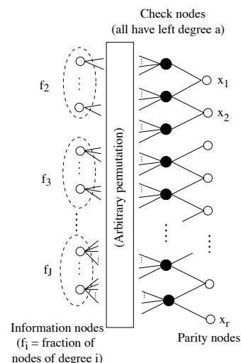
Figure 4.8: Graphe de Tanner d'un code IRA, extraite de [36].
