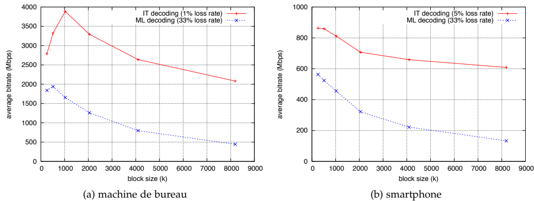
Figure 6.4: Vitesse du codec LDPC-Staircase, en décodage IT (bon canal) et ML (mauvais canal) ( CR = 2/3 , N_1 = 7 , symboles de 1024 octets, et G = 1 ).
