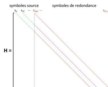
Figure 4.9: Matrice de parité (512, 100) des codes à triple diagonale de Zivkoic.
