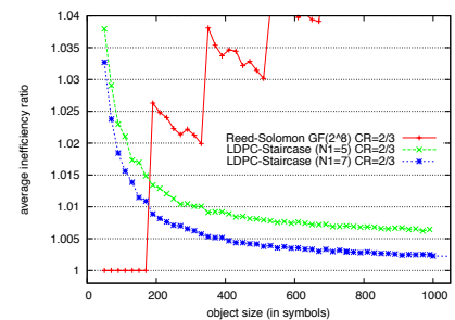
Figure 5.3: Capacités de correction des codes LDPC-Staircase ( ML ) et Reed-Solomon, avec ( k = 1024 , CR = 2/3 , G = 1 ).
