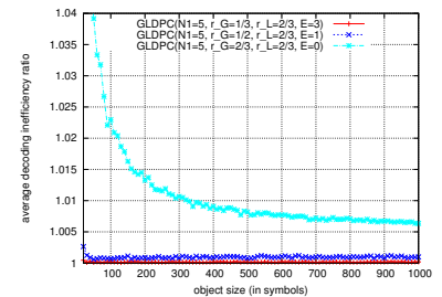
Figure 7.7: Capacités de correction moyennes des codes GLDPC-Staircase (cas où E = 0 , N_1 = 5 et non 7, bleu clair) et LDPC-Staircase avec E = 1 ( r_G = 1/2 ) et E = 3 ( r_G = 1/3 ).
