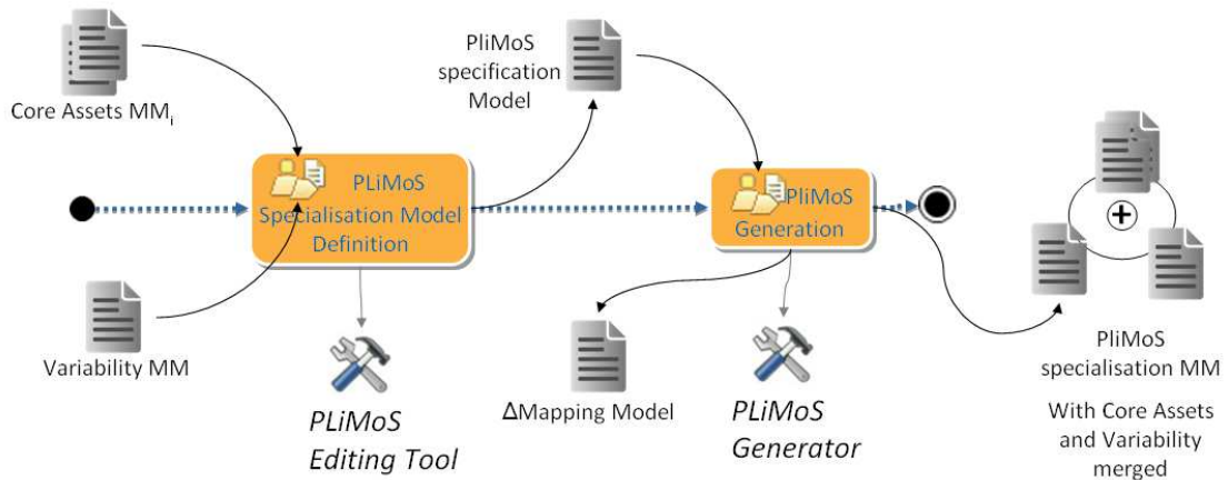
FIGURE 9.1: Processus de génération des modèles PLiMoS_{specialisation}
