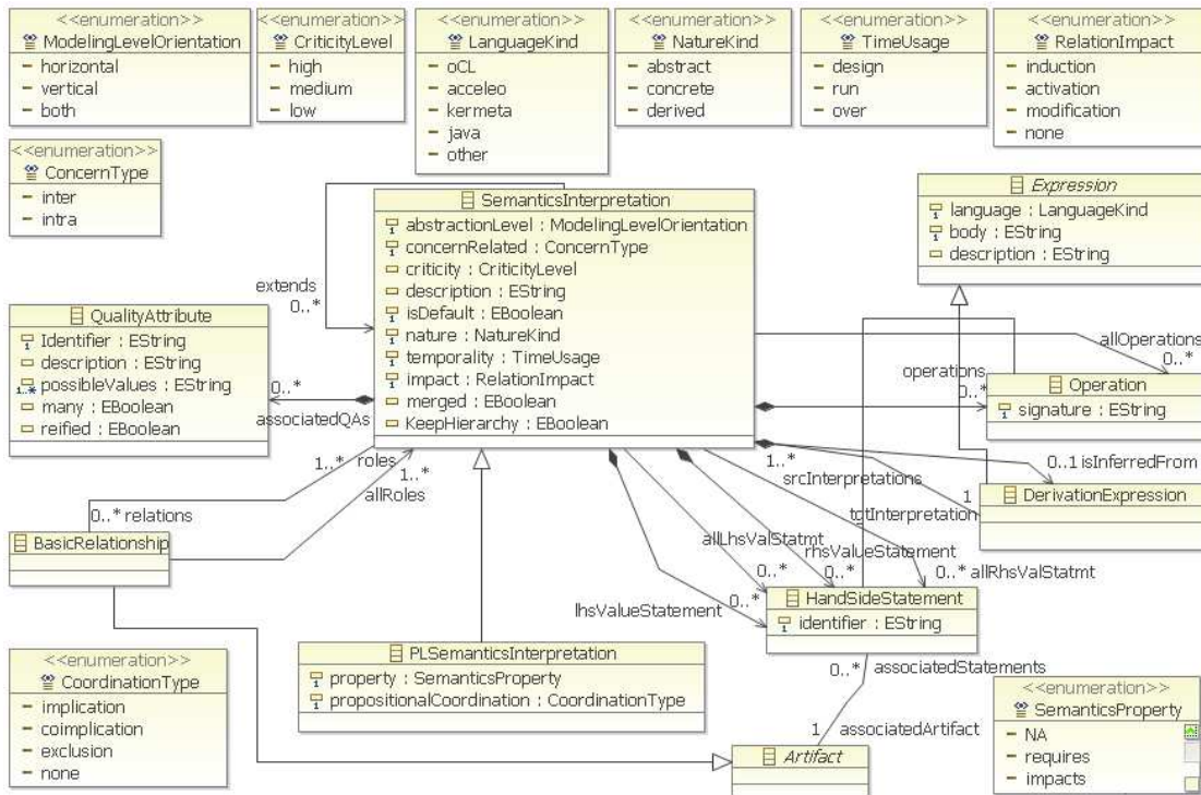
FIGURE 8.2: PLiMo definition : interprétations sémantiques
