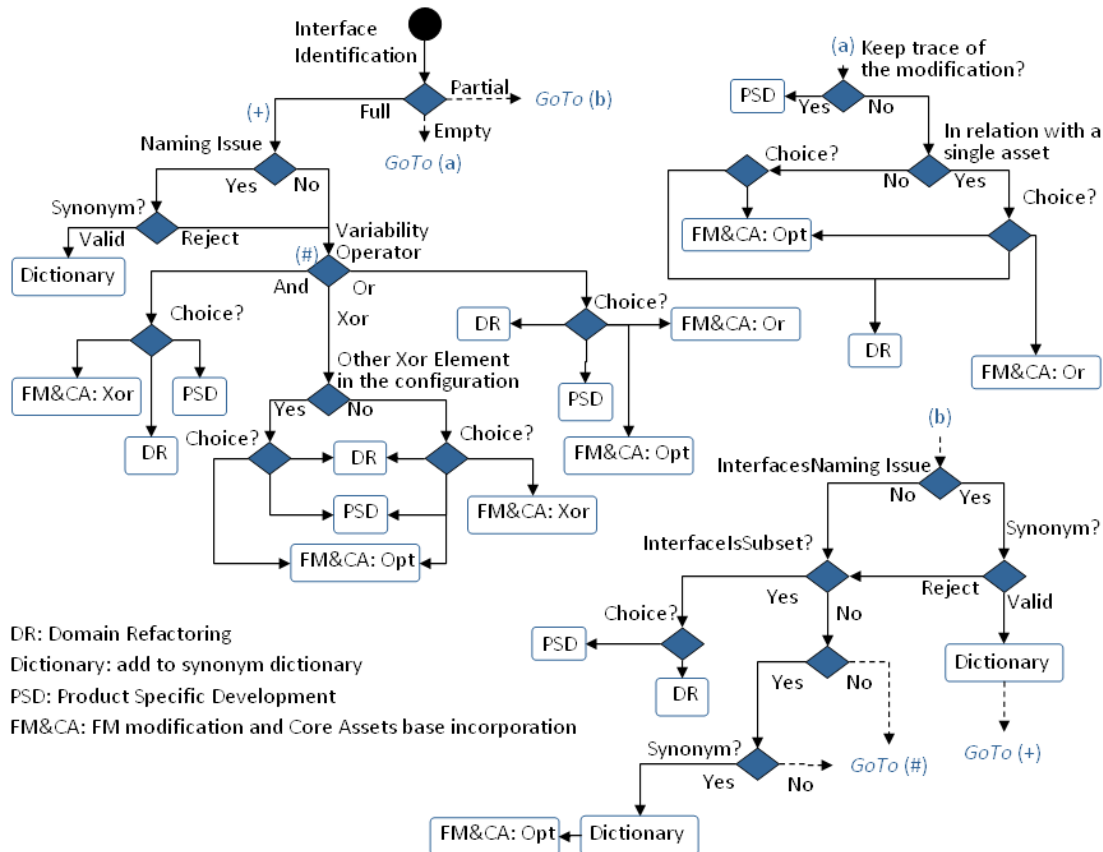
FIGURE 11.10: Logique de l'algorithme de retour
