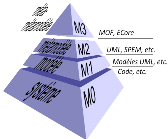
FIGURE 2.3: Pyramide de modélisation de l'OMG [OMG11a].
