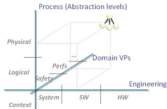
FIGURE 6.3: Cadre conceptuel de variabilité à quatre dimensions
