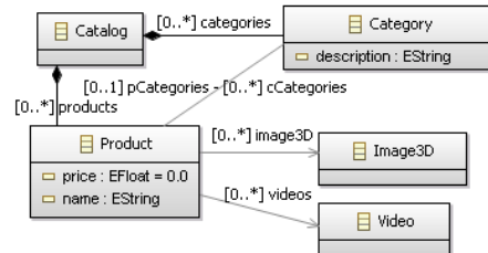
FIGURE 11.7: L'exemple du ItemCatalog SPL - produit étendu avec des capacités de stockage vidéo
