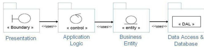
FIGURE B.2: Vue d'ensemble du patron BCED.
