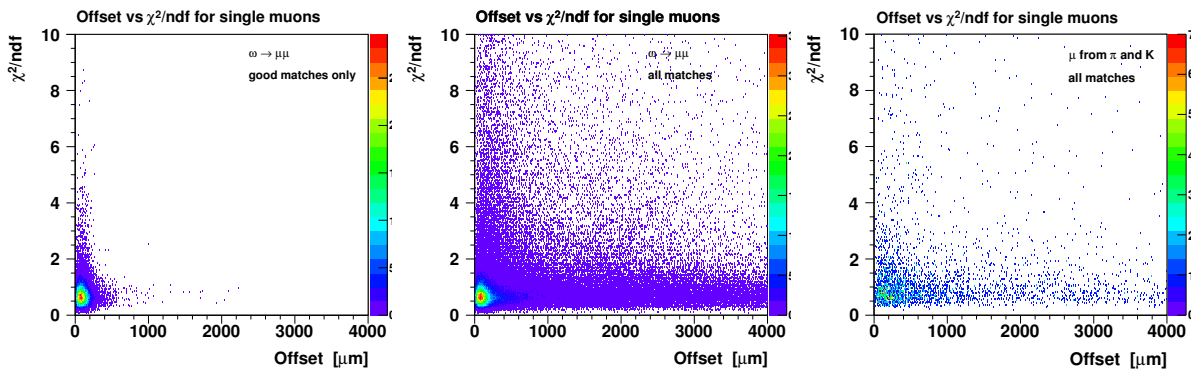
FIGURE 5.35 — Distributions dans le plan \chi^2 – Offset, des muons issus de décroissance \omega \rightarrow \mu\mu en imposant une concordance parfaite entre le MFT et le MUON (gauche), sans sélection sur la concordance (centre) comparée à la distribution pour des muons issus de décroissance semi-leptonique de pions et kaons (droite).
