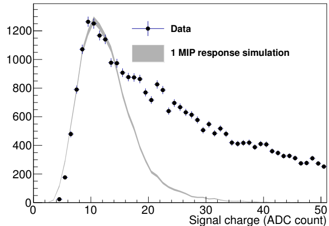
FIGURE 2.10 — Comparaison de la réponse d'une voie de détection, entre les données prises en collisions pp à \sqrt{s} = 7 TeV (points) et la simulation complète du détecteur (courbe grisée).
