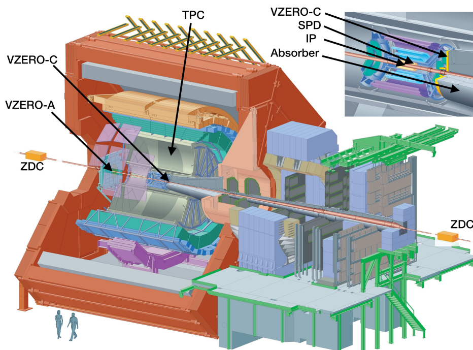
FIGURE 2.1 – Vue schématique de l'expérience ALICE.
