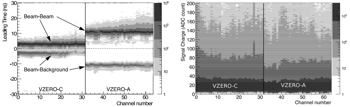
FIGURE 2.11 – Temps de l’impulsion issue du PMT en nanoseconde en fonction du numéro de la voie (gauche), charge intégrée en nombre de coups ADC en fonction du numéro de la voie (droite) pour des collisions pp à \sqrt{s} = 7 TeV. Les numéros de voie de 0 à 31 correspondent au VZERO-C et les numéros de 32 à 63 au VZERO-A.
