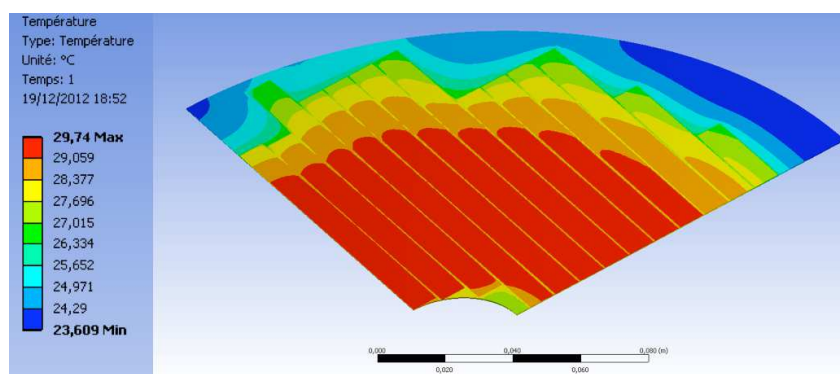
FIGURE 5.19 – Simulation thermique d'un quart de plan.
