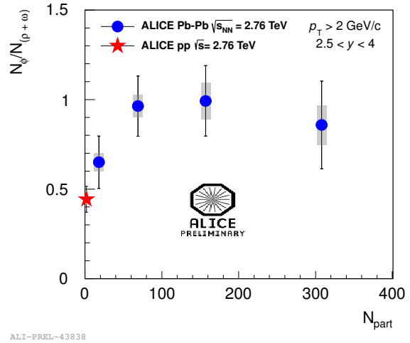
FIGURE 4.12 – Rapport N_\varphi/N_{\rho+\omega} corrigé des effets d'acceptance et d'efficacité en fonction du nombre de participants à la collision. Les résultats en collisions Pb–Pb à \sqrt{s_{NN}} = 2.76 TeV (ronds bleus) sont comparés au résultat en collisions pp à \sqrt{s} = 2.76 TeV (étoile rouge). Les barres grisées représentent l'incertitude systématique.
