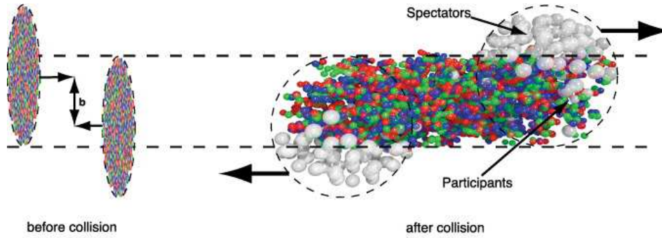
FIGURE 2.18 – Vue schématique de la collision entre deux noyaux de plomb illustrant les principes de paramètre d'impact et de nucléons participant et spectateurs.
