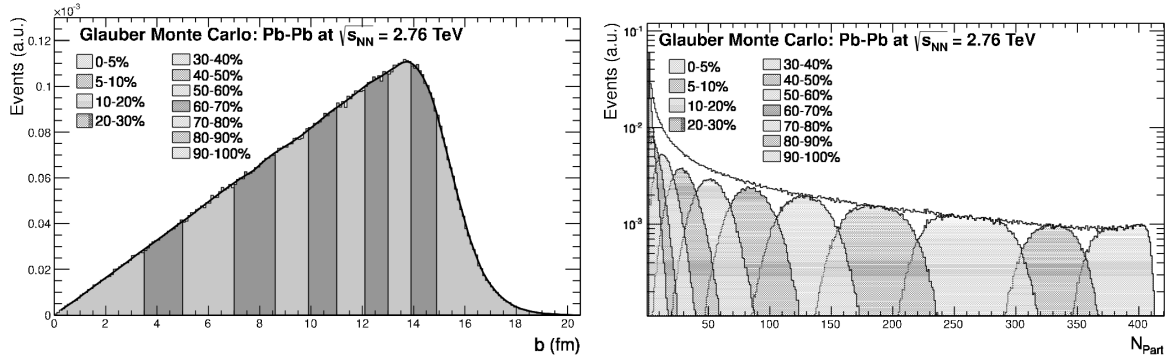
FIGURE 2.19 – Propriétés géométriques des collisions Pb–Pb à \sqrt{s_{NN}} = 2.76 TeV obtenues par un calcul Monte Carlo basé sur le modèle de Glauber. Distribution du paramètre d’impact b (gauche) et distribution du nombre de nucléons participant N_{part} (droite). Les tranches en centralité effectuées sur la distribution de b sont reportées sur la distribution de N_{part} . Figures extraites de [44].
