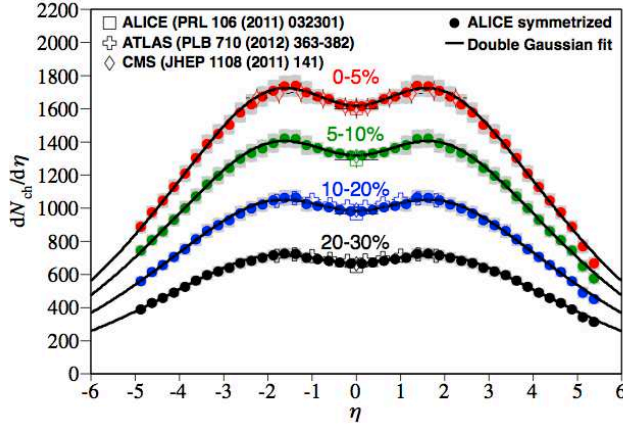
FIGURE 2.26 — Densité de particules chargées en fonction de la pseudo-rapacité mesurée pour quatre classes en centralité. Les points expérimentaux sont ajustés par une fonction du type
