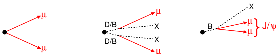
FIGURE 5.6 – Vues schématiques de trois événements dimuons différents; dimuon prompt (gauche); dimuon issu de désintégrations de hadrons charmés ou beaux (centre); dimuon provenant de la désintégration d'un hadron beau en J/\psi (droite).
