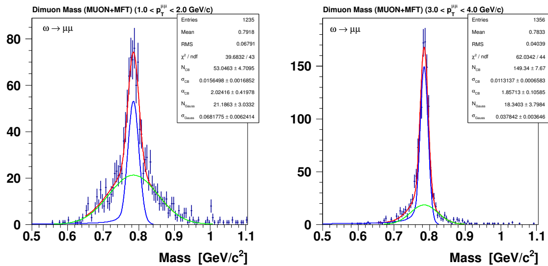
FIGURE 5.38 — Résolution en masse pour le signal \omega \rightarrow \mu\mu pour deux intervalles en p_T^{\mu\mu} : 1 < p_T^{\mu\mu} < 2 \text{ GeV}/c (gauche) et 3 < p_T^{\mu\mu} < 4 \text{ GeV}/c (droite). Les contributions au spectre en masse totale (courbe rouge) où les deux muons ont une concordance parfaite (courbe bleue) et où l'un des muons a une mauvaise concordance (courbe verte) sont représentées.
