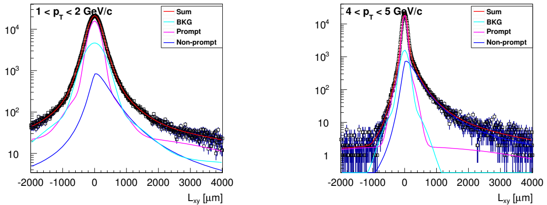
FIGURE 5.33 — Minimisation du spectre de pseudo-proper decay length par superposition des formes attendues pour les J/\psi prompts et secondaires et pour le bruit de fond. Présentation de la minimisation pour deux tranches en impulsion transverse : 1 < p_T < 2 \text{ GeV}/c (gauche) et 4 < p_T < 5 \text{ GeV}/c (droite).
