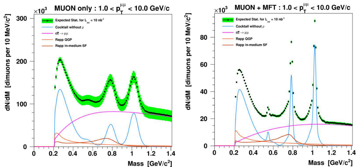
FIGURE 5.39 — Spectre en masse invariante pour p_T > 1 \text{ GeV}/c après soustraction du bruit de fond combinatoire pour les scénarios sans (gauche) et avec MFT (droite). La distribution totale est décrite par la superposition des différents signaux. La bande verte représente l'incertitude induite par la soustraction du bruit de fond, supposant une erreur sur sa normalisation au niveau de 0.25 % par intervalle de masse invariante.
