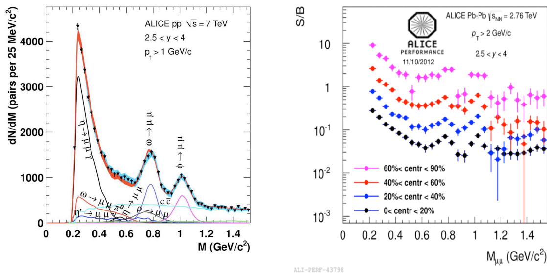
FIGURE 5.4 – Spectre en masse invariante obtenu en collisions pp à \sqrt{s} = 7 TeV dans la région des basses masses ( M < 1.5 \text{GeV}/c^2 ), les données (triangles noirs) sont ajustées par une superposition de sources hadroniques [66] (gauche). Rapport signal sur bruit (S/B) dans la région des basses masses pour quatre tranches en centralité en collisions Pb–Pb à \sqrt{s_{NN}} = 2.76 TeV (droite).
