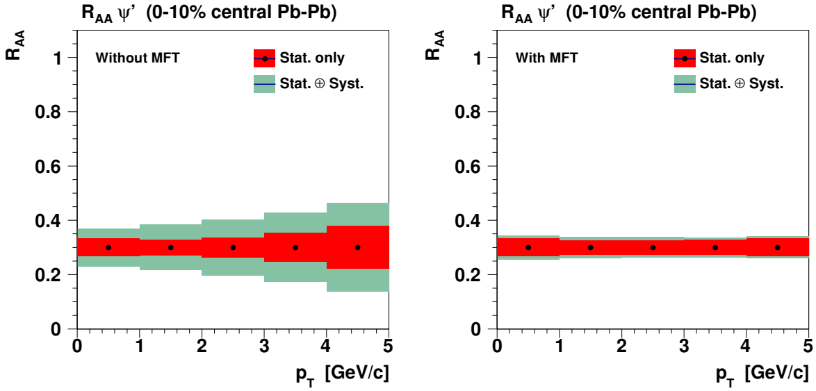
FIGURE 5.31 – Incertitudes statistiques et systématiques attendues pour la mesure du rapport de modification nucléaire du \psi' pour une centralité de 0–10% en collisions Pb–Pb à \sqrt{s_{NN}} = 5.5 TeV en fonction du p_T pour les scénarios sans (gauche) et avec (droite) MFT. Une luminosité intégrée de 10 \text{ nb}^{-1} est supposée.
