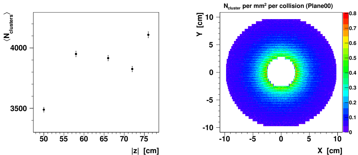
FIGURE 5.20 – Multiplicité moyenne de clusters par plan pour une collision centrale Pb–Pb (gauche) ; densité de clusters par mm 2 dans le plan 1 (droite).
