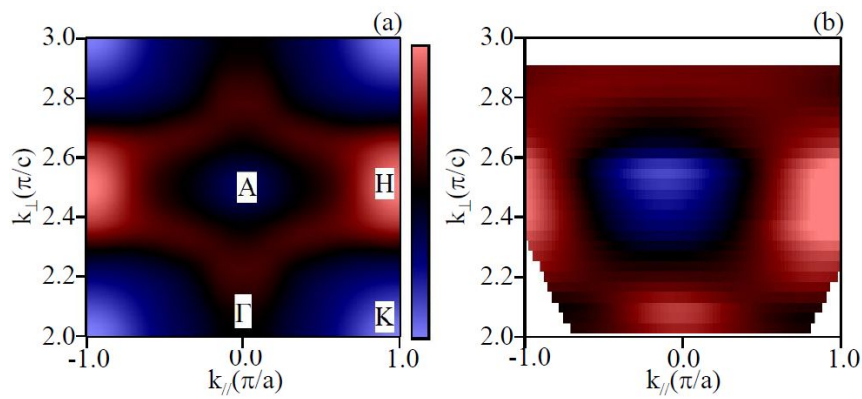
Fig. V-11 : surface iso-énergie à l'énergie de liaison du pic B simulée (a) et mesurée (b) dans le plan \Gamma\text{AHK}
