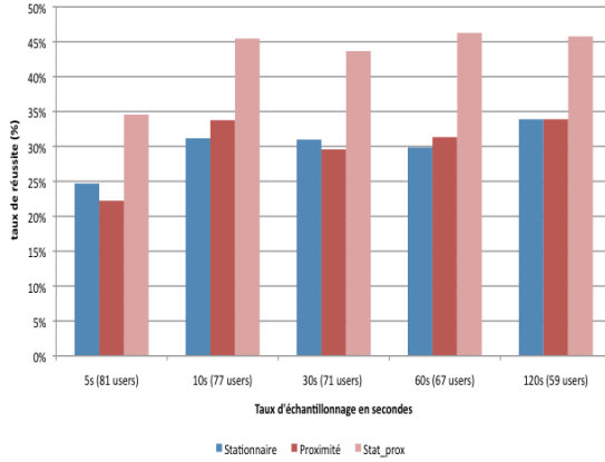
Figure 7: Taux de réussite des désanonymizers sur l'ensemble des données Geolife.
