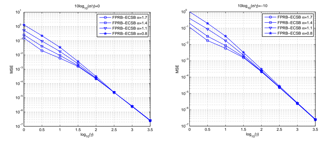
FIGURE 3.7 Erreur quadratique moyenne de l'estimation du paramètre de dispersion en fonction de \gamma pour différentes valeurs de \alpha avec 10\log_{10}(\sigma/\gamma) = 0 (gauche) et 10\log_{10}(\sigma/\gamma) = -10 (droite)
