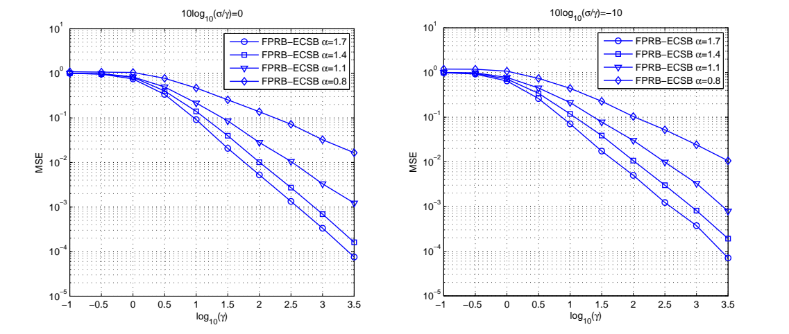
FIGURE 3.6 MSE de l'estimation du signal OFDM en fonction de 10\log_{10}(\gamma) pour différentes valeurs de \alpha avec 10\log_{10}(\sigma/\gamma) = 0 (gauche) et 10\log_{10}(\sigma/\gamma) = -10 (droite)
