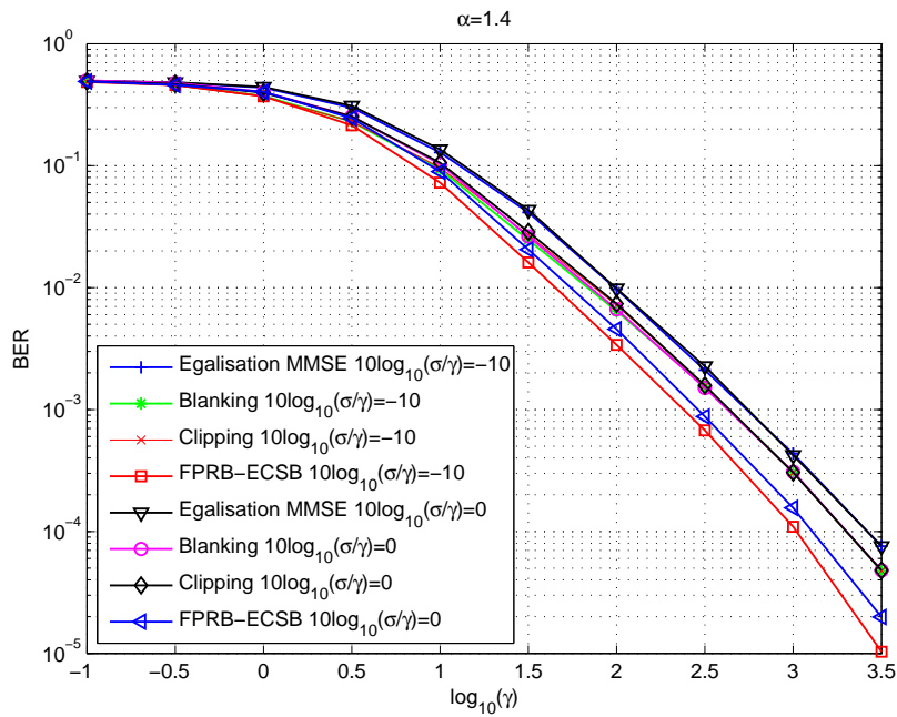
FIGURE 3.16 Performance en terme de taux d'erreur binaire de la méthode proposée FPRB-ECSB pour différentes valeurs du rapport 10 \log_{10}(\sigma/\gamma) avec \alpha = 1.4 .
