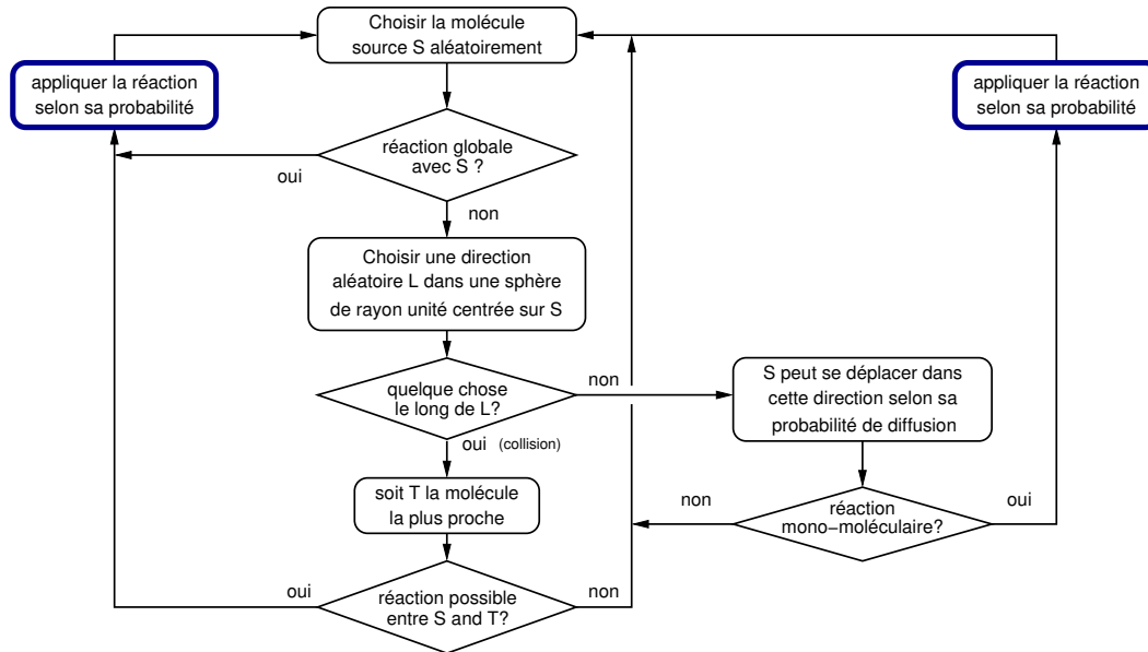
FIG. 3.3: Algorithme de calcul de l'évolution de l'état du système à chaque pas de temps.
