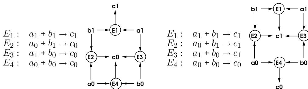
FIG. 6.3: Porte ET (à gauche) et porte OU (à droite) implémentées en mode dual .
