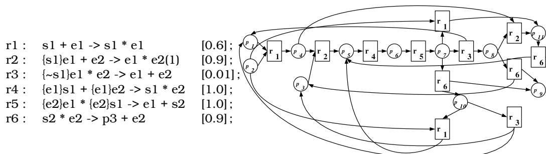
FIG. 4.2: Réseau métabolique montrant la catalyse par deux enzymes successives d'un substrat s_1 en produit p_3 , la réaction intermédiaire étant canalisée. Dans le réseau de Petri à droite, les places P_1 à P_{11} représentent respectivement les espèces : e_1 , s_1 , e_2 , e_1s_1 , e_1s_1e_2 , e_1s_1e_2s_1 , e_1e_2s_2 , e_2s_2 , p_3 , e_1e_2 , et e_1s_1e_2s_2 .
