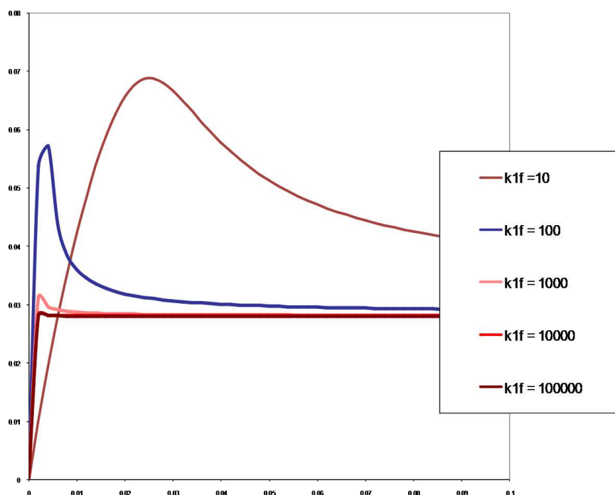
FIG. 5.2: Comportements non-linéaires d'une FDS à deux enzymes selon les paramètres cinétiques.
