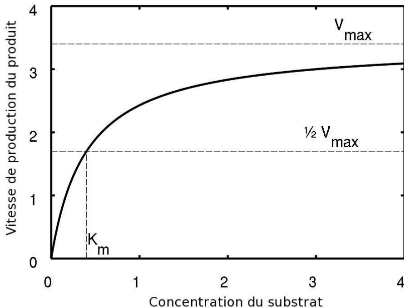
FIG. 2.2: Vitesse de production de P en fonction de [S]
