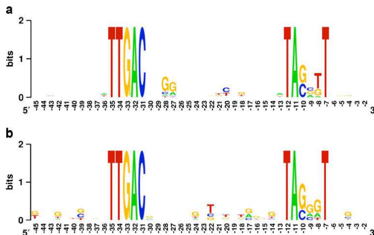
FIG. 7.1: Séquences des 14 plus faibles (a) et des 14 plus forts (b) promoteurs affichées avec WebLogo.
