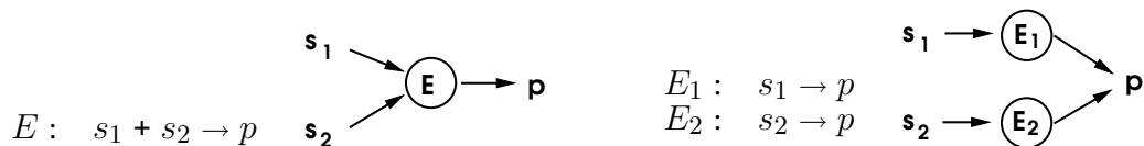
FIG. 6.2: Porte ET (à gauche) et porte OU (à droite) implémentées en mode mono .
