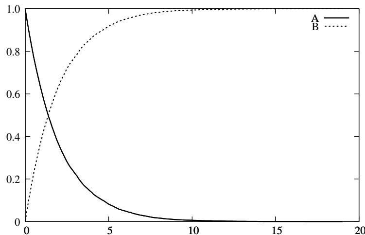
FIG. 2.1: Réaction mono-moléculaire
