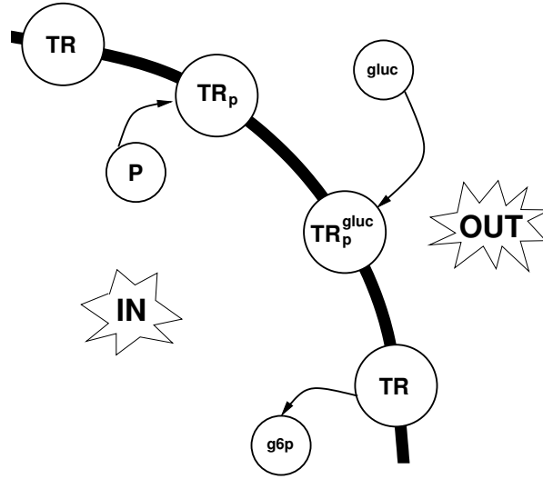
FIG. 3.5: Transporteur membranaire actif EII^{BC} chez E. coli .
