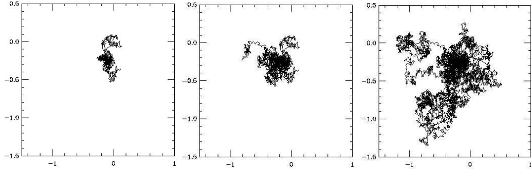
FIG. 3.1: Trajectoire simulée d'une particule suivant un mouvement brownien projeté sur un plan. Avec D = 0.16\mu^2/sec , les axes gradués en microns, la position à t = 0 est (0, 0) . Les figures sont prises après 1 seconde, 3 secondes et 10 secondes.
