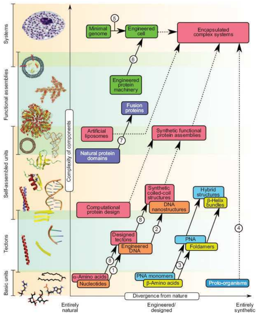
FIG. 6.1: Représentation des différentes approches de la biologie de synthèse selon Bromley et. al [40].
