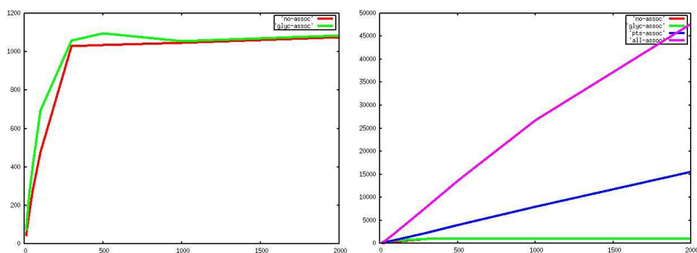
FIG. 5.4: Courbes de production de pyruvate en fonction de la concentration initiale de PEP.
