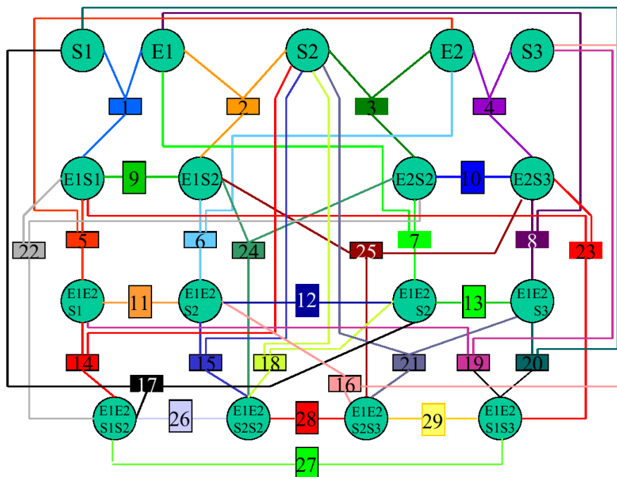
FIG. 5.1: Toutes les réactions possibles avec deux enzymes successives pouvant former une FDS. Le système comprend 17 espèces chimiques (enzymes libres, métabolites et complexes) représentées dans des cercles. Ces espèces sont reliées entre elles par 29 réactions représentées dans des rectangles.
