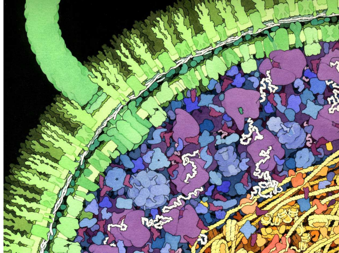
FIG. 3.2: Représentation de l'encombrement moléculaire du cytosol d'une bactérie, E. coli . (origine : The Machinery of Life , David S. Goodsell)
