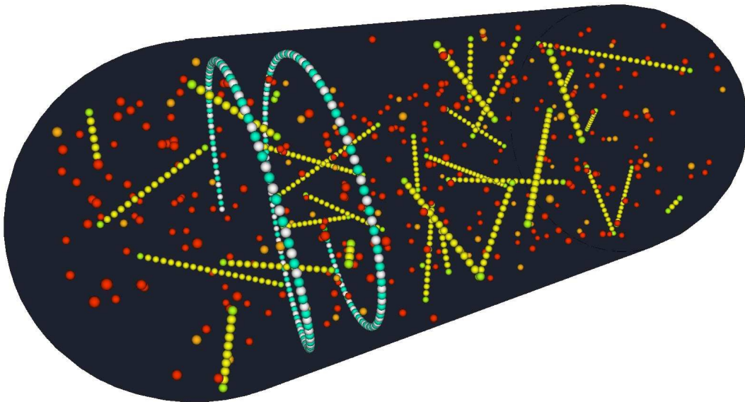
FIG. 3.4: Assemblage de filaments linéaires et hélicoïdaux.
