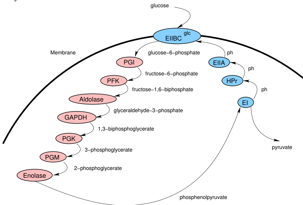
FIG. 5.3: Couplage entre la voie de la glycolyse (enzymes en rose) et la voie de la PTS (enzymes en bleu).
