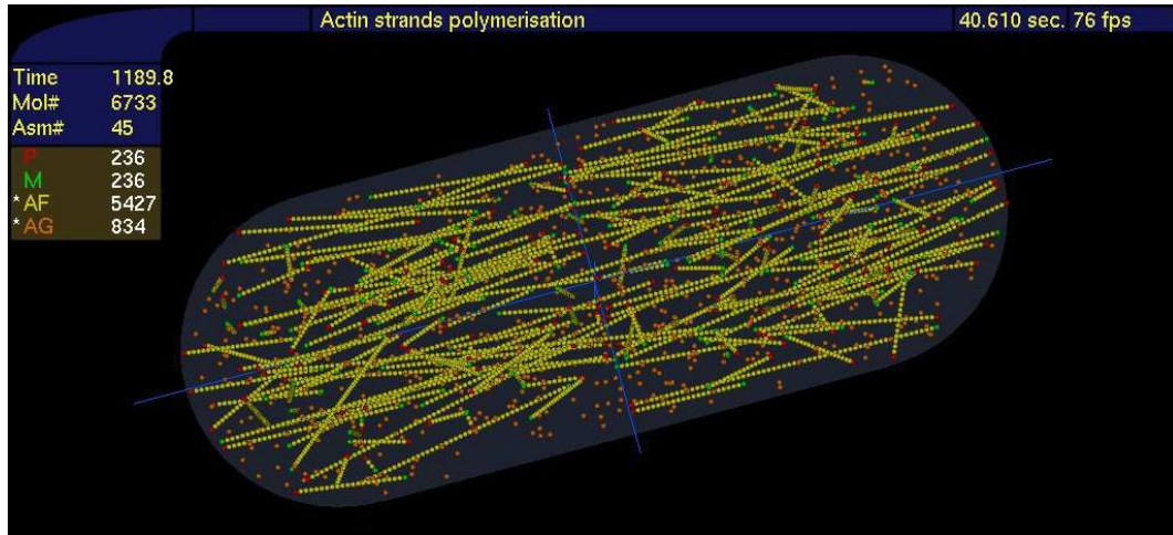
FIG. 4.1: Auto alignement de filaments d'actine le long de l'axe principal du compartiment.
