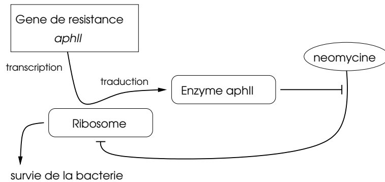
FIG. 7.4: Réseau d'interactions entre le gène aphII et la neomycine.
