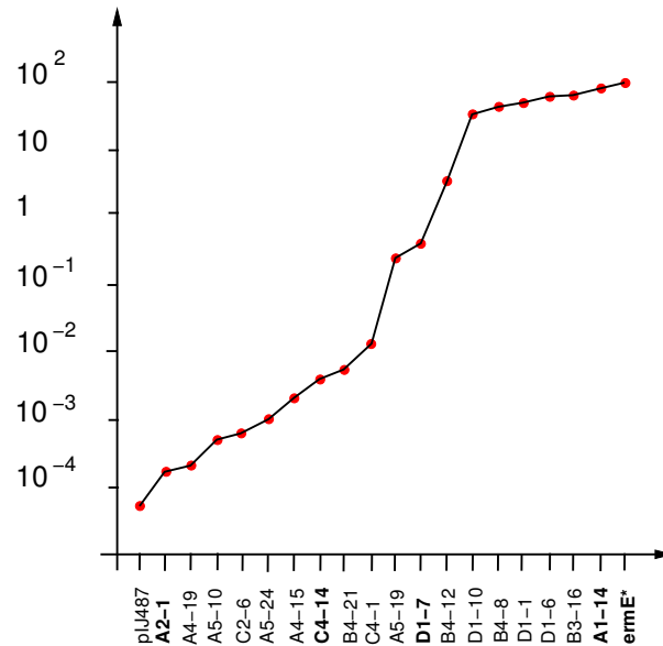
FIG. 7.2: Courbe de survie en fonction de la force des promoteurs dans une culture contenant 100 \mu\text{g/ml} de neomycine. Le taux d'expression des promoteurs dont les noms sont en gras à aussi été mesuré par RT-PCR.
