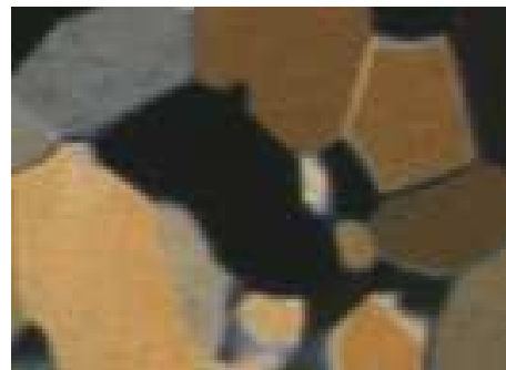
Figure 1.13 : Zoom d'une image de cristaux de glace (Dôme C, profondeur : 229 mètres).
