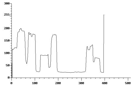
Filtre médian.
