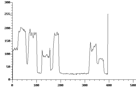
Image initiale.
