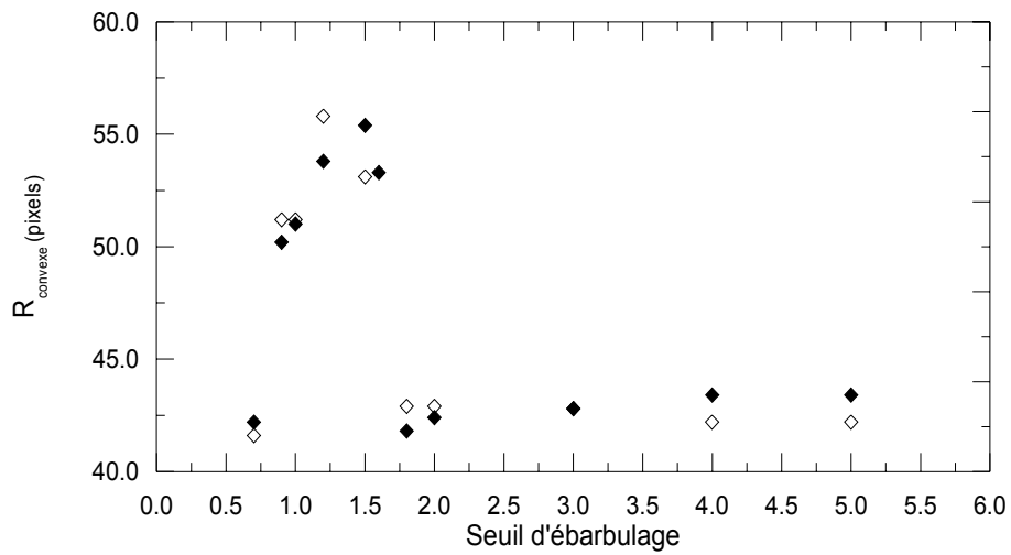
Figure 4.19 : Evolution du rayon convexe moyen pour deux amas de cercles, le critère d'ébarbulage est : \text{Pts perdus} / \text{Total des pts} \leq T .
