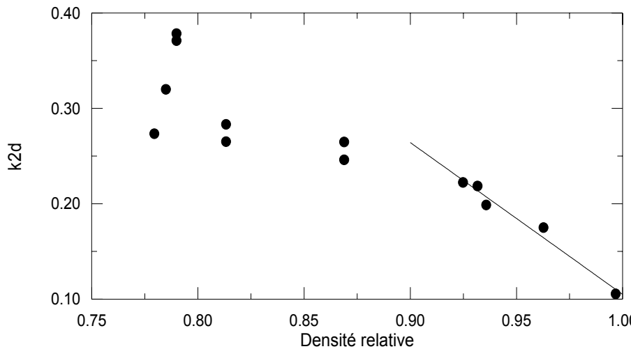
Figure 5.10 : k_{2d} en fonction de la densité relative à Vostok (Bh7).
