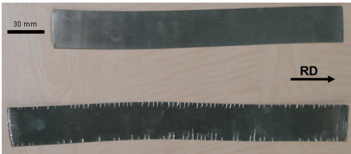
Figure IV-9 : échantillons laminés de manière symétrique (haut) et asymétrique (bas) en 5 passes
