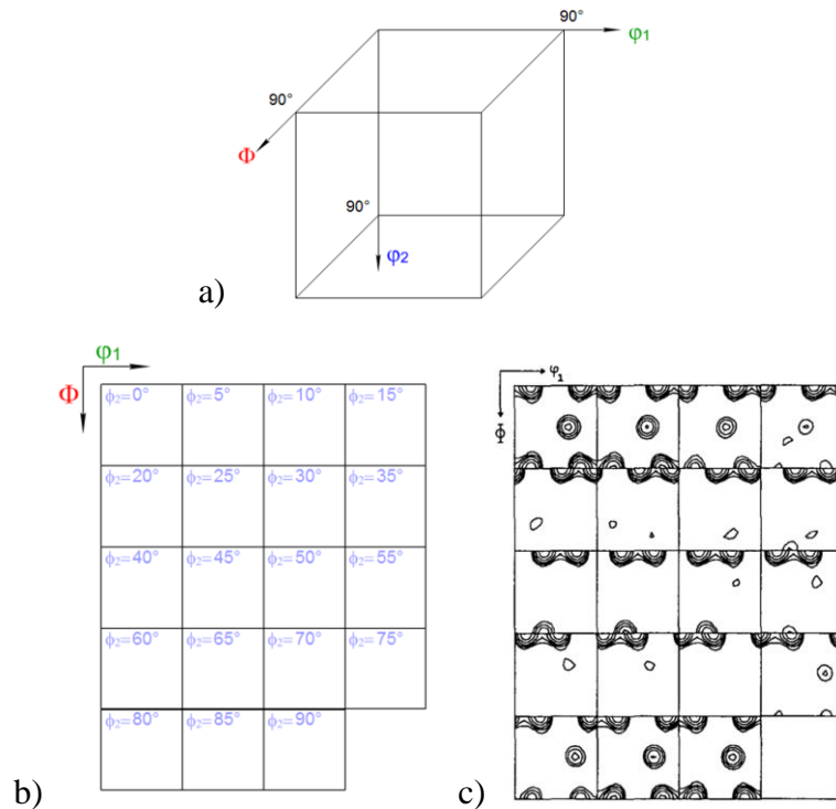
Figure II-5 : espace d'Euler avec les angles \varphi_1 , \Phi , \varphi_2 (a) et ODF en 2 dimensions (b) [AluMatter], ODF d'un alliage Al - 1% Mn - 0,5% Mg chauffé à 573 K (c) [Daaland 96]
