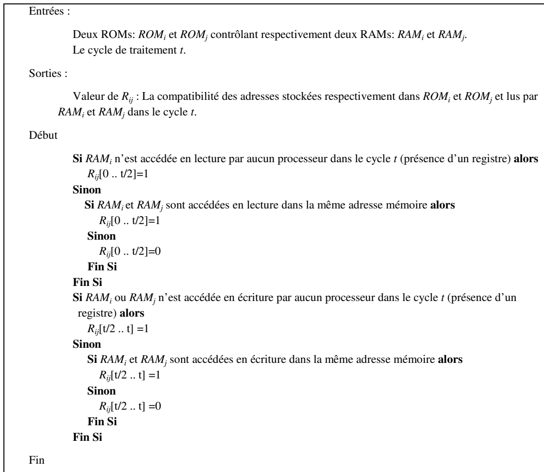
Figure4. 27 Compatibilité des adresses mémoires envoyées par deux ROMs dans un cycle de traitement particulier
