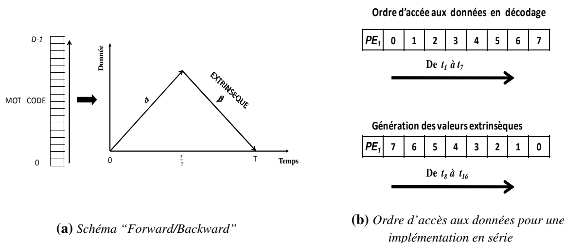
Figure 1.8 Implémentation en série d'un Turbo décodeur
