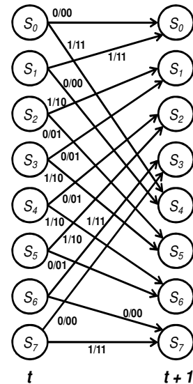
Figure 1.4 Diagramme de treillis
