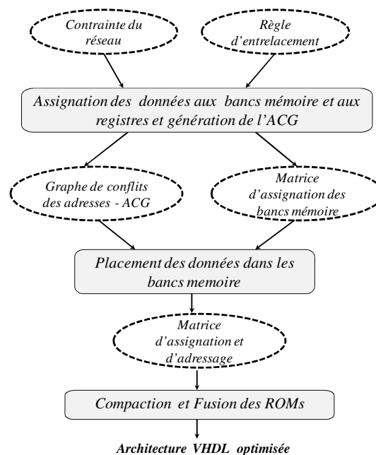
Figure 5. 2 Flot de conception générique
