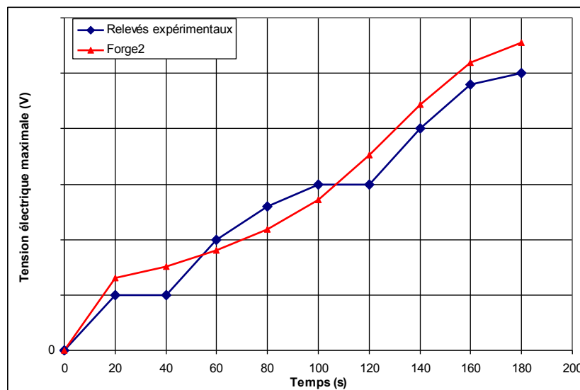
Figure 30 : Comparaison de la tension mesurée et calculée pendant le procédé d'électrorefoulage
