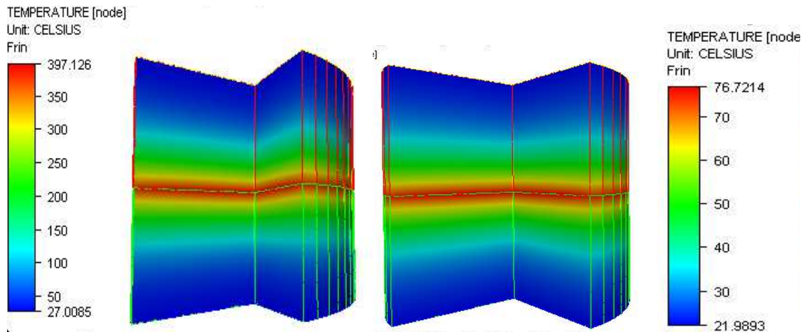
Figure 34 : Influence de la résistance électrique de contact sur le champ de température, à gauche cette résistance vaut 7 \times 10^{-7} \Omega \cdot m^2 , à droite = 1 \times 10^{-7} \Omega \cdot m^2 [C 20]
