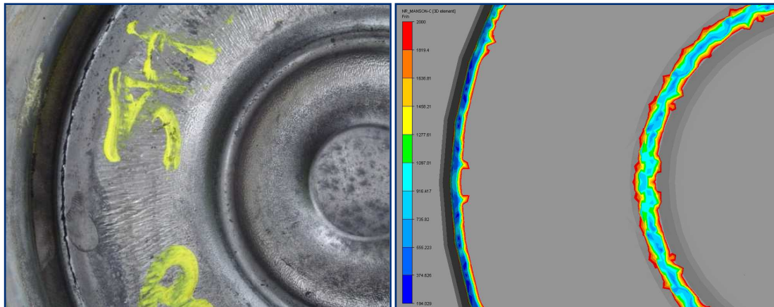
Figure 28 : Comparaison de localisation de fissuration d'outils avec la prédiction de durée de vie numérique
