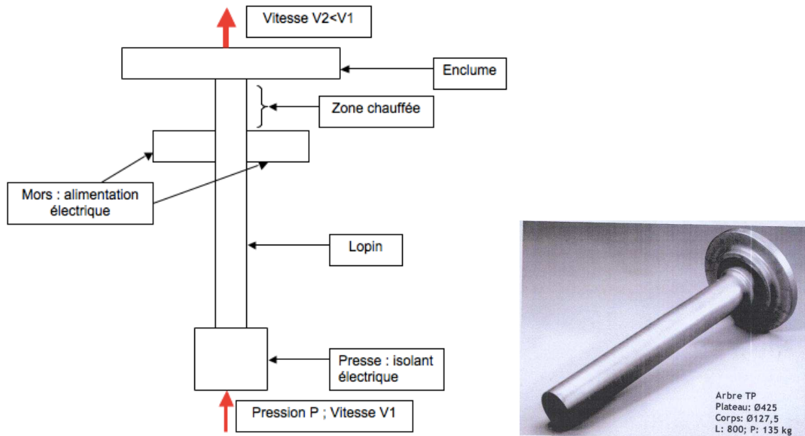
Figure 29 : Schéma de principe du procédé d'électrorefoulage et exemple de pièce concernée
