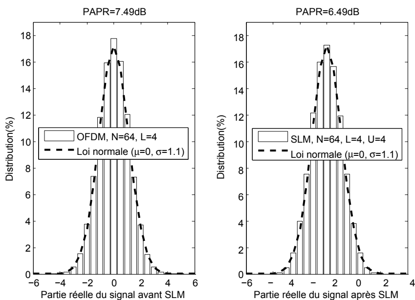
FIGURE 2.2 – Les distributions du signal avant et après le SLM comparées avec celle d'une loi gaussienne.
