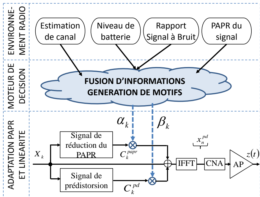
FIGURE 4.17 – Principe de l’approche conjointe dynamique par ajout de signal
