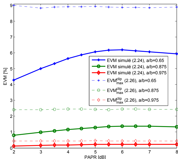
FIGURE 2.9 – L'EVM en fonction du PAPR pour a/b = 0.65, 0.875 et 0.975 lorsque le clipping est utilisé pour réduire le PAPR
