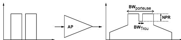
FIGURE 1.4 – Calcul du NPR
