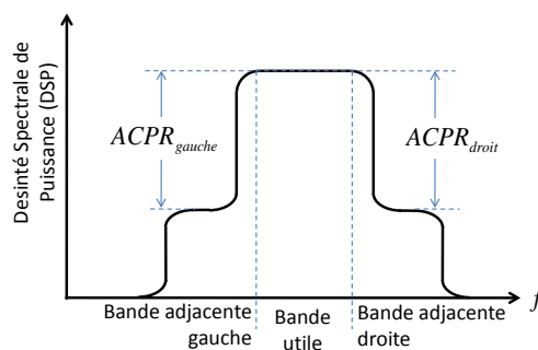
FIGURE 1.3 – Calcul de l'ACPR
