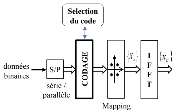
FIGURE 1.24 – Principe conceptuel de la technique de codage
