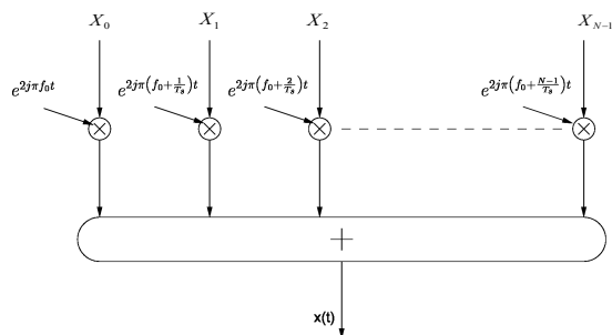
FIGURE 1.16 – Représentation schématique d’un symbole OFDM
