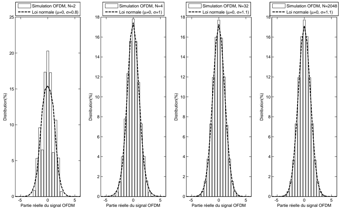
FIGURE 2.1 – Comparaison de la distribution de la partie réelle du signal OFDM et de la loi gaussienne (i.e Normale) pour plusieurs valeurs de N (2, 4, 32 et 2048).
