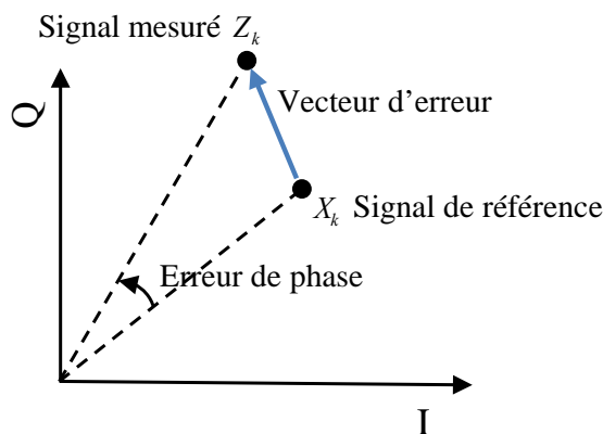
FIGURE 1.5 – Illustration du calcul de l'EVM
