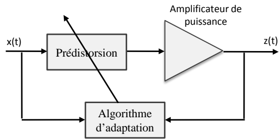
FIGURE 1.14 – Principe de l'adaptation directe
