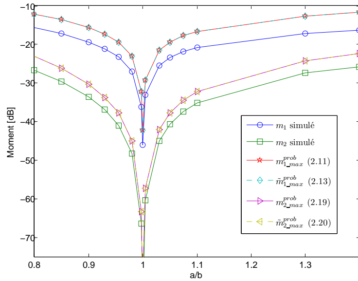
FIGURE 2.5 – Moments du premier et du second ordre de l'erreur de prédistorsion \epsilon^{pd} lorsque le SLM est utilisé comme technique de réduction du PAPR
