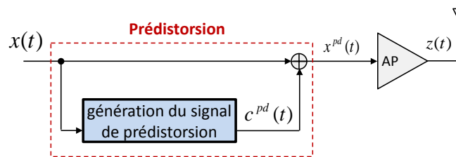
FIGURE 4.1 – Schéma de principe de la prédistorsion par ajout de signal
