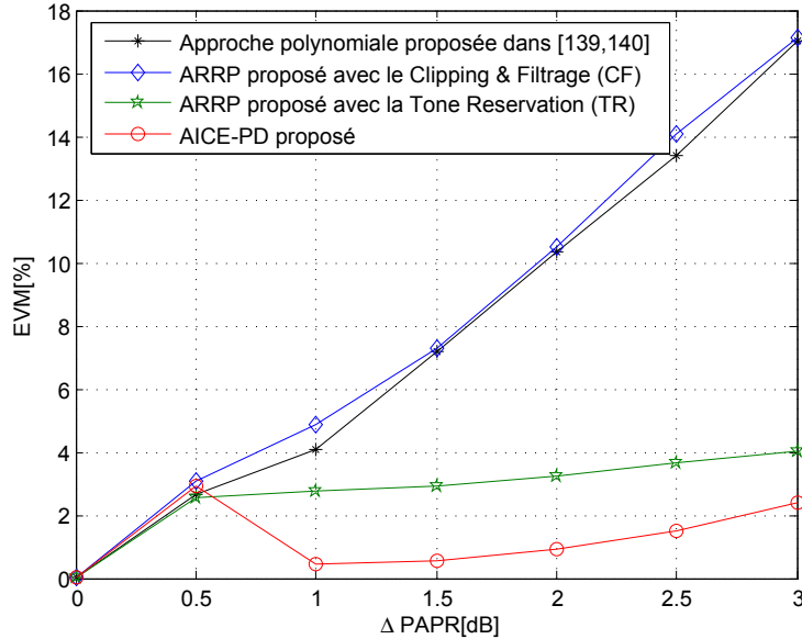
FIGURE 5.18 – Résultats de simulations comparatives de l’approche polynomiale et de l’approche conjointe unifiée par ajout de signal
