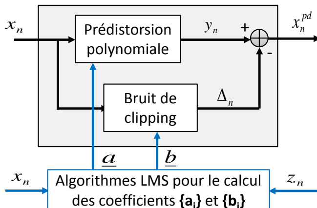
FIGURE 3.19 – Principe de fonctionnement de l'approche conjointe polynomiale
