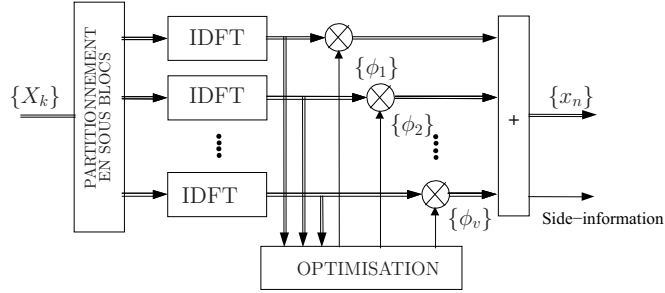
(b) Principe du modulateur PTS
