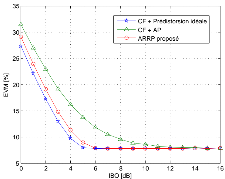
FIGURE 5.9 – EVM de l’approche conjointe unifiée par ajout de signal basée sur l’ARRP.
