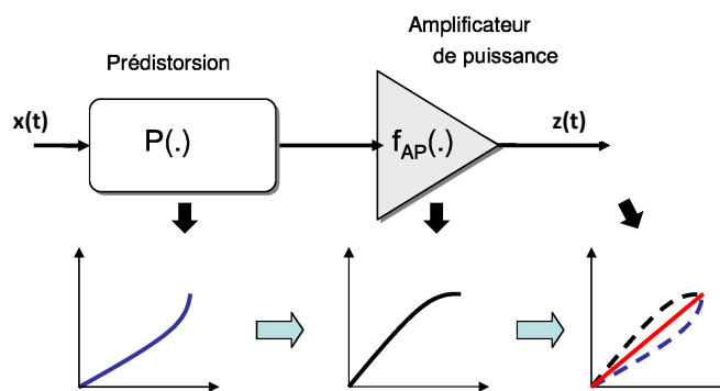
FIGURE 1.12 – Principe des techniques de Prédistorsion
