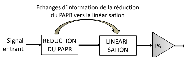
FIGURE 3.6 – Approche conjointe collaborative unidirectionnelle qui adapte la linéarisation en fonction de la réduction du PAPR
