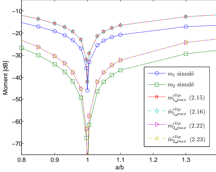
FIGURE 2.6 – Moment de premier et second ordre de l’erreur de prédistorsion lorsque le clipping est utilisé comme technique de réduction du PAPR
