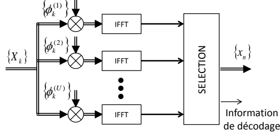
FIGURE 1.22 – Schéma de base d'un modulateur SLM
