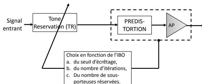
FIGURE 3.13 – Adaptation des paramètres de la TR (a-seuil d'écrêtage, b-nombre d'itérations, c-nombre de sous-porteuses réservées) en fonction de l'IBO de l'amplificateur "linéarisé" [88, 90, 137]
