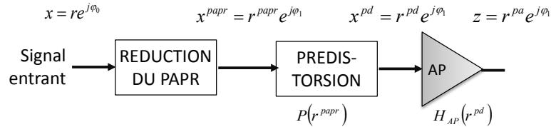
FIGURE 2.4 – Modèle simplifié du système de transmission
