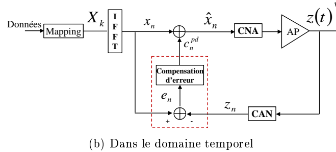
FIGURE 4.5 – Diagramme en blocs de l’AICE pour la génération du signal additionnel de prédistorsion
