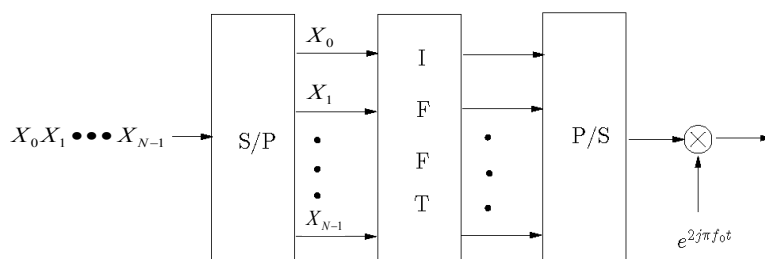
FIGURE 1.18 – Architecture de base d'un modulateur numérique OFDM
