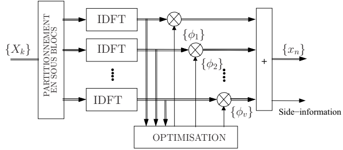
(b) Principe du modulateur PTS
