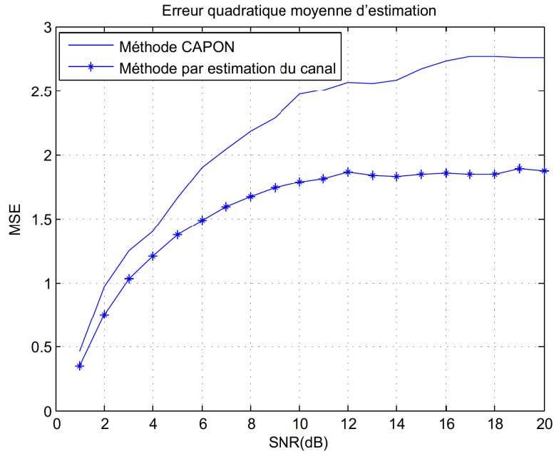
FIGURE 5.7 – Estimation du rapport signal sur bruit
