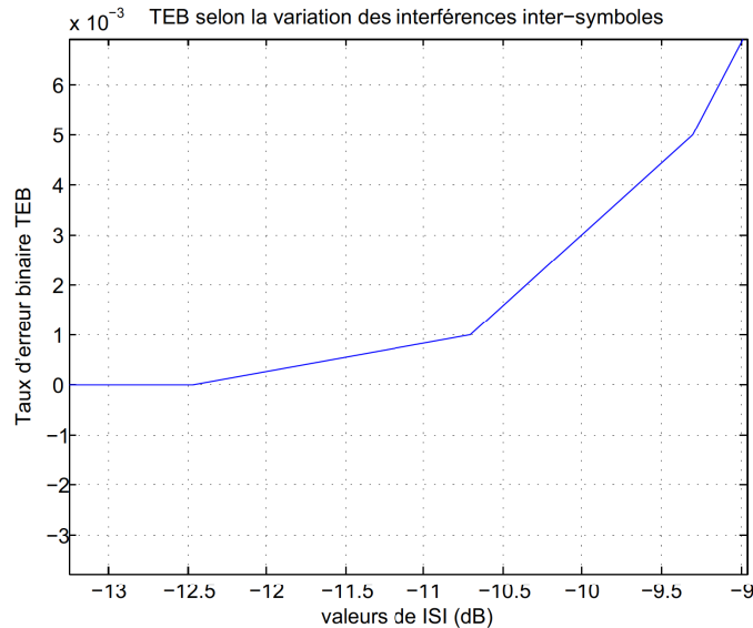
FIGURE 4.4 – Variation du taux d'erreur binaire selon la puissance des interférences inter-symboles TEB = f(ISI)
