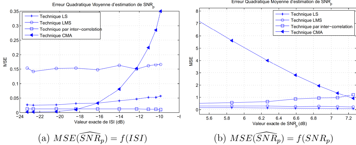
FIGURE 4.2 – Erreur quadratique moyenne de \widehat{SNR}_p
