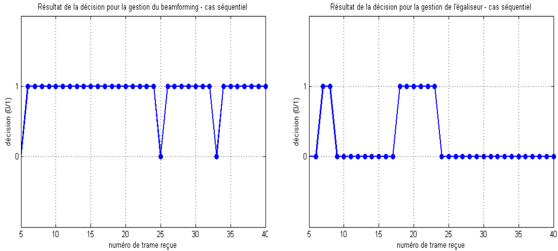
(a) Décisions pour le beamforming '0' : Activer le beamforming '1' : Désactiver le beamforming (b) Décisions pour l'égaliseur après beamforming '0' : Activer l'égaliseur '1' : Désactiver l'égaliseur
