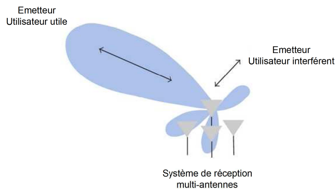
FIGURE 5.1 – Principe du beamforming en réception
