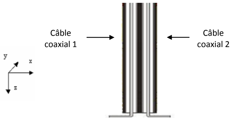
Figure 37 : Sonde pour capter la composante E_{x+} et E_{x-} du champ électrique
