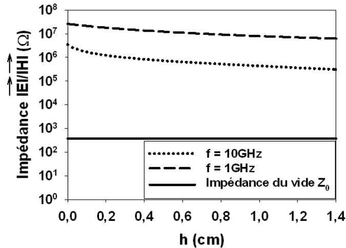
Figure 50 : Rapport \frac{|E|}{|H|} de la sonde E_z
