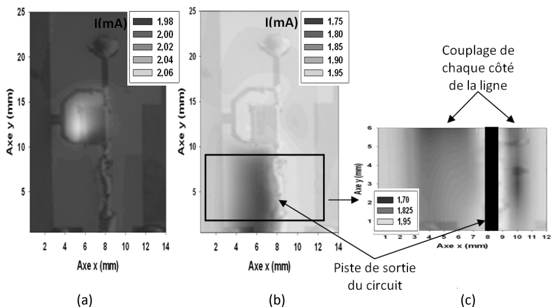
Figure 144 : Cartographies en agression via la sonde Hz1 à une hauteur h = 2.5 \text{ mm} du circuit imprimé aux fréquences (a) f = 2.5 \text{ GHz} et (b) 1.12 \text{ GHz} . (c) Cartographie de la sortie du circuit lorsque la sonde est à une hauteur h = 0.5 \text{ mm} du circuit imprimé à la fréquence de 1.12 \text{ GHz} .
