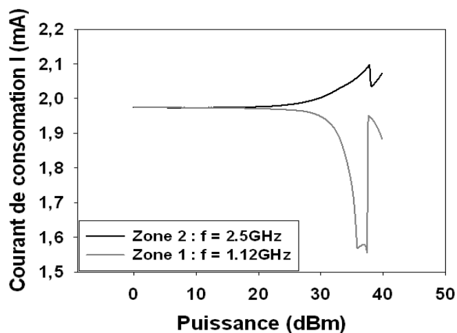
Figure 145 : Variation du courant de consommation I en fonction de la puissance du signal d'agression lors de l'injection de l'agression en zone 1 et 2 pour des fréquences respectives de 1.12 \text{ GHz} et 2.5 \text{ GHz}
