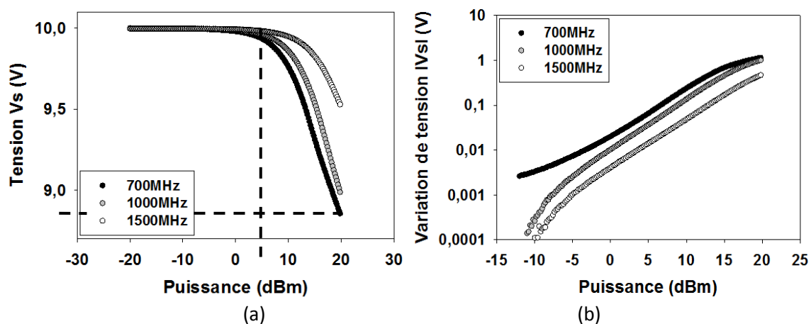
Figure 130 : Influence de la puissance du signal d'agression sur la tension de sortie V_s pour trois fréquences différentes
