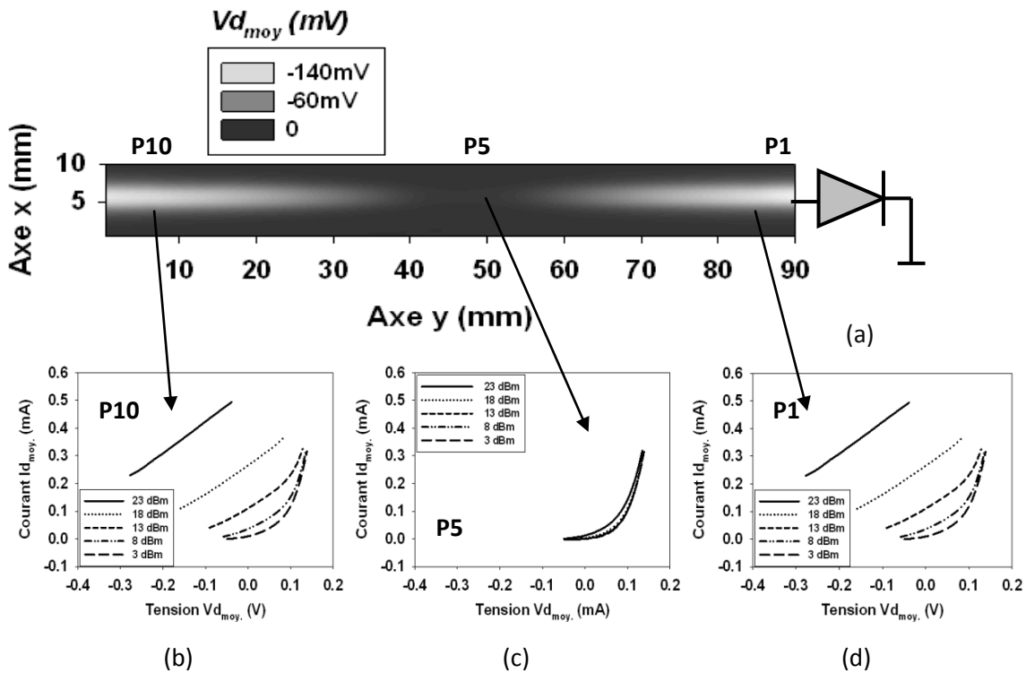
Figure 115 : Influence de la position du point d'injection via la sonde Ez3 : (a) cartographie en injection à f = 1.07 \text{ GHz} de la ligne micro-ruban devant la diode, injection d'un signal d'agression (b) en P10, (c) en P5, (d) en P1
