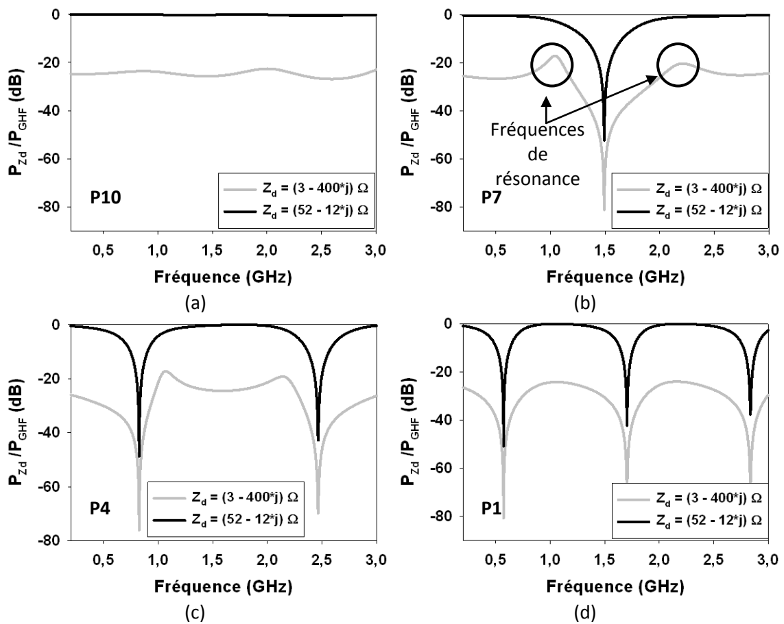
Figure 99 : Module du coefficient de transmission entre le système d'injection en mode conduit et la ligne micro-ruban simulé pour différents points d'injection et différentes impédances Z_d : (a) P10, (b) P7, (c) P4, (d) P1
