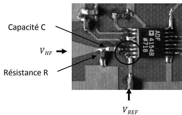
Figure 204 : Photographie du routage de l'ADF4154
