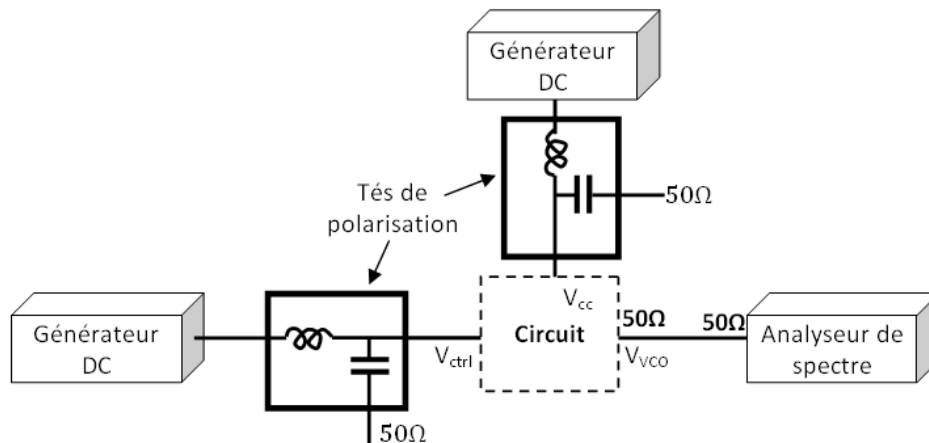
Figure 151 : Schéma du montage de mesure
