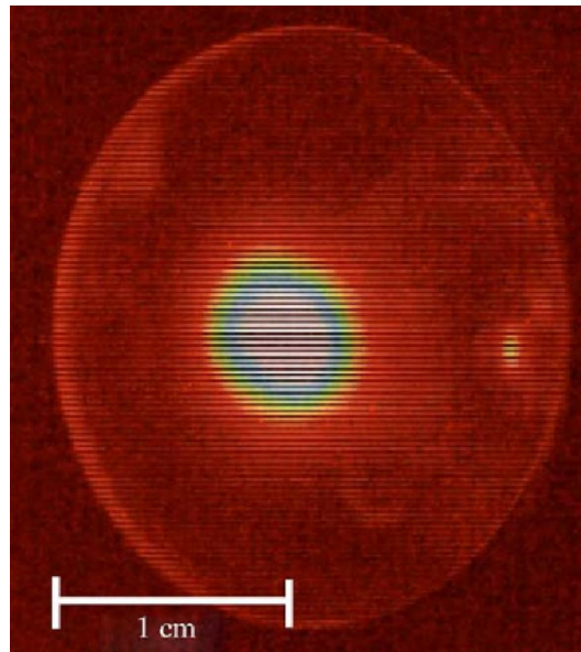
Figure III. 11 section efficace du faisceau d'électrons sur une lame de YAG/Ce enregistrée par une caméra CCD. La lumière observée sur la lame est la lumière Cerenkov. 9
