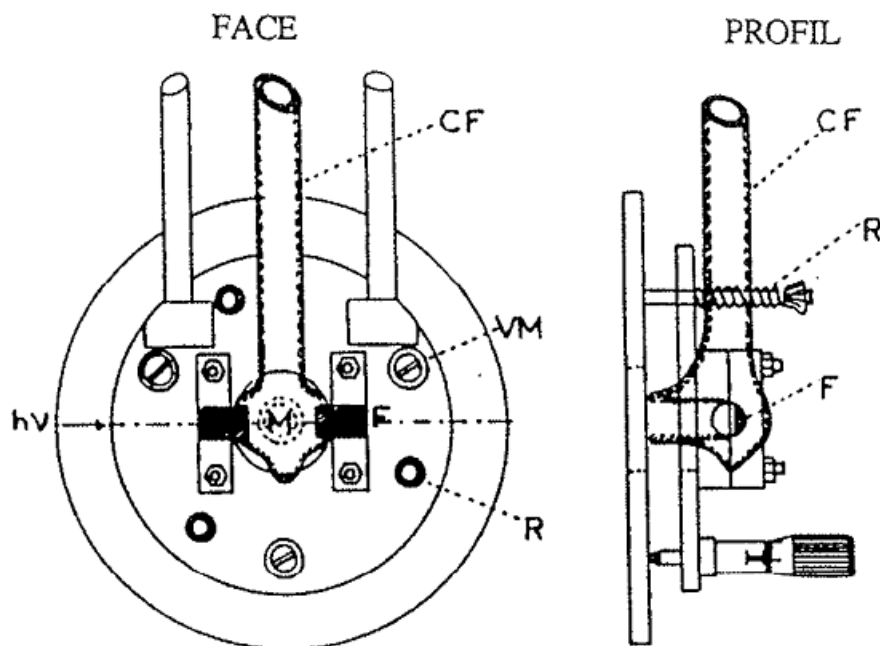
Figure III. 3 Montage de la cellule d'irradiation utilisée dans les expériences de radiolyse pulsée nanoseconde. La figure montre la vue de face de la cellule ainsi que sa vue de profil. CF : Cellule Febetron, VM : Vis Micrométrique, F : Fenêtre optique, R : Ressort de positionnement de la cellule. 18
