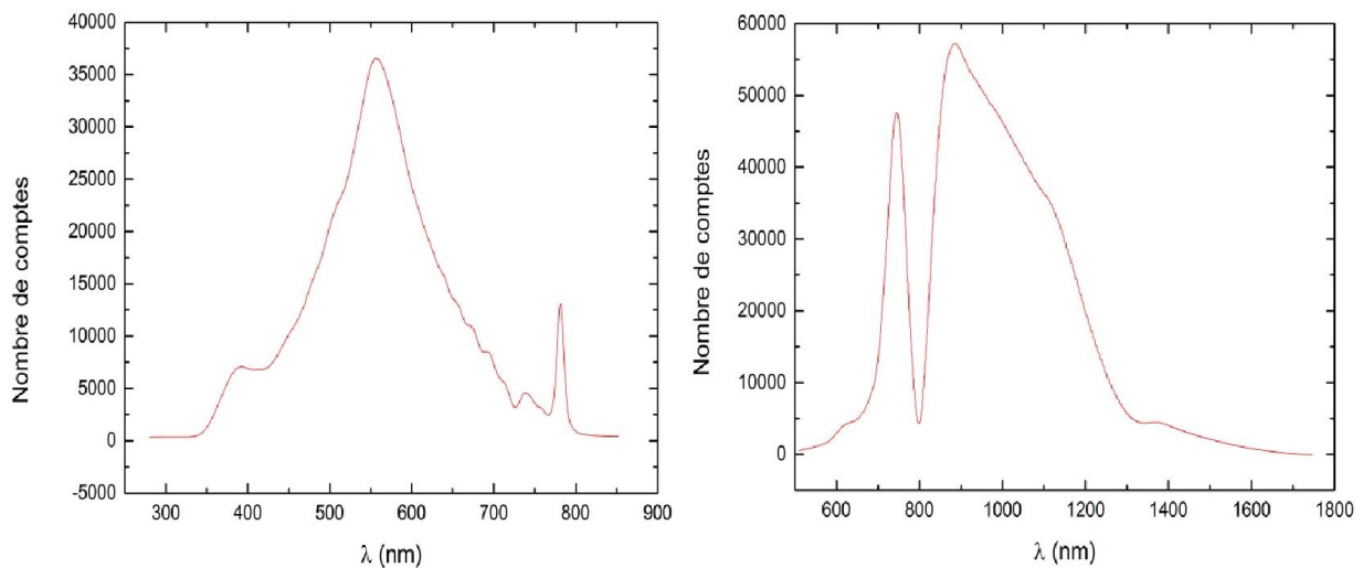
Figure III. 13 Spectres des supercontinuum. Figure gauche : spectre du supercontinuum visible généré dans le cristal \text{CaF}_2 , Figure droite : spectre du supercontinuum IR généré dans le cristal YAG, un filtre spécial permet de couper la longueur d'onde fondamentale du laser autour de 800 nm.
