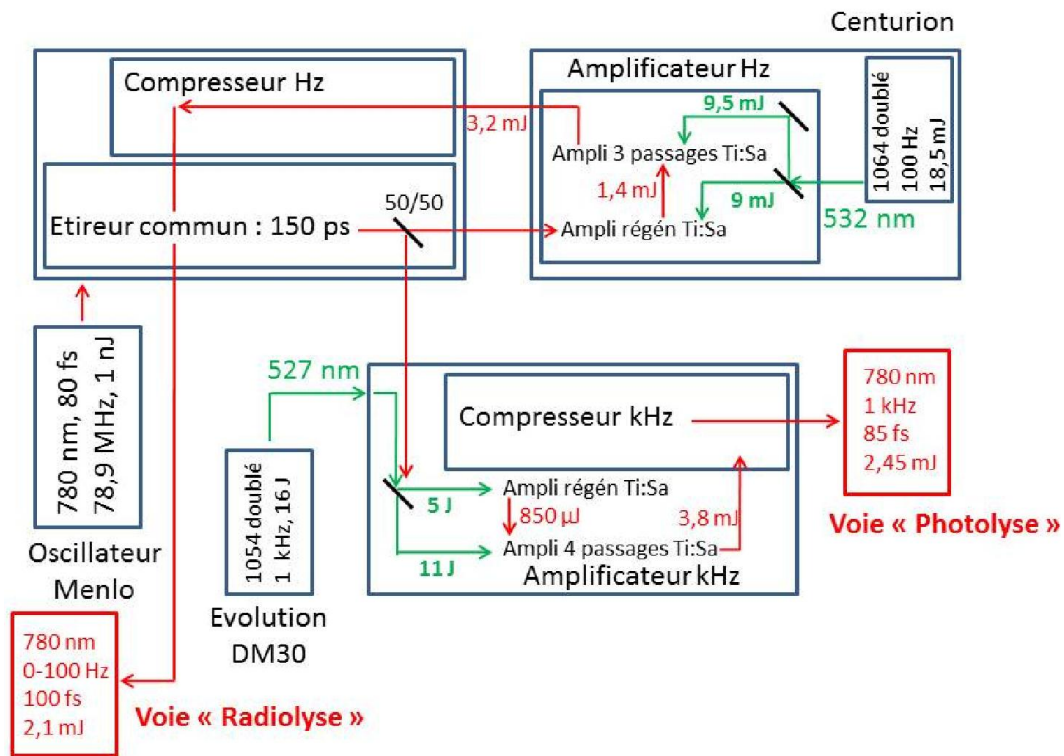
Figure III. 6 Schéma général de la chaîne laser femtoseconde d'ELYSE.
