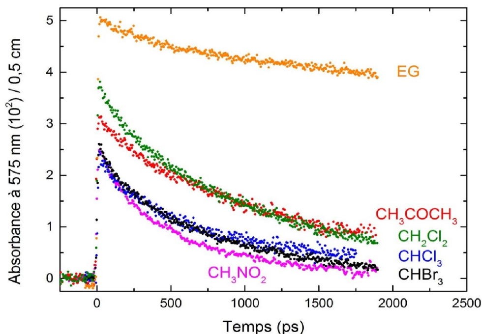
Figure VI. 13 Cinétiques de déclin de l'électron solvaté enregistrées à 575 nm dans EG en présence de 0,4 mol L -1 de capteur. L'absorption transitoire des fenêtres de la cellule d'irradiation a été soustraite de l'absorption transitoire totale.
