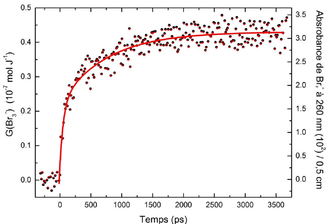
Figure V. 28 Rendement radiolytique de formation de \text{Br}_3^- dans la solution de \text{NaBr} 6 \text{ mol L}^{-1} en fonction du temps.
