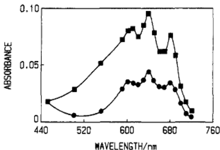
Figure II. 20 Spectre d'absorption du radical \text{NO}_3^\bullet dans l'acide nitrique à 6 \text{ mol L}^{-1} (■) et dans le nitrate de sodium à 6 \text{ mol L}^{-1} (●), 100 ns après le passage du faisceau d'électrons. 125
