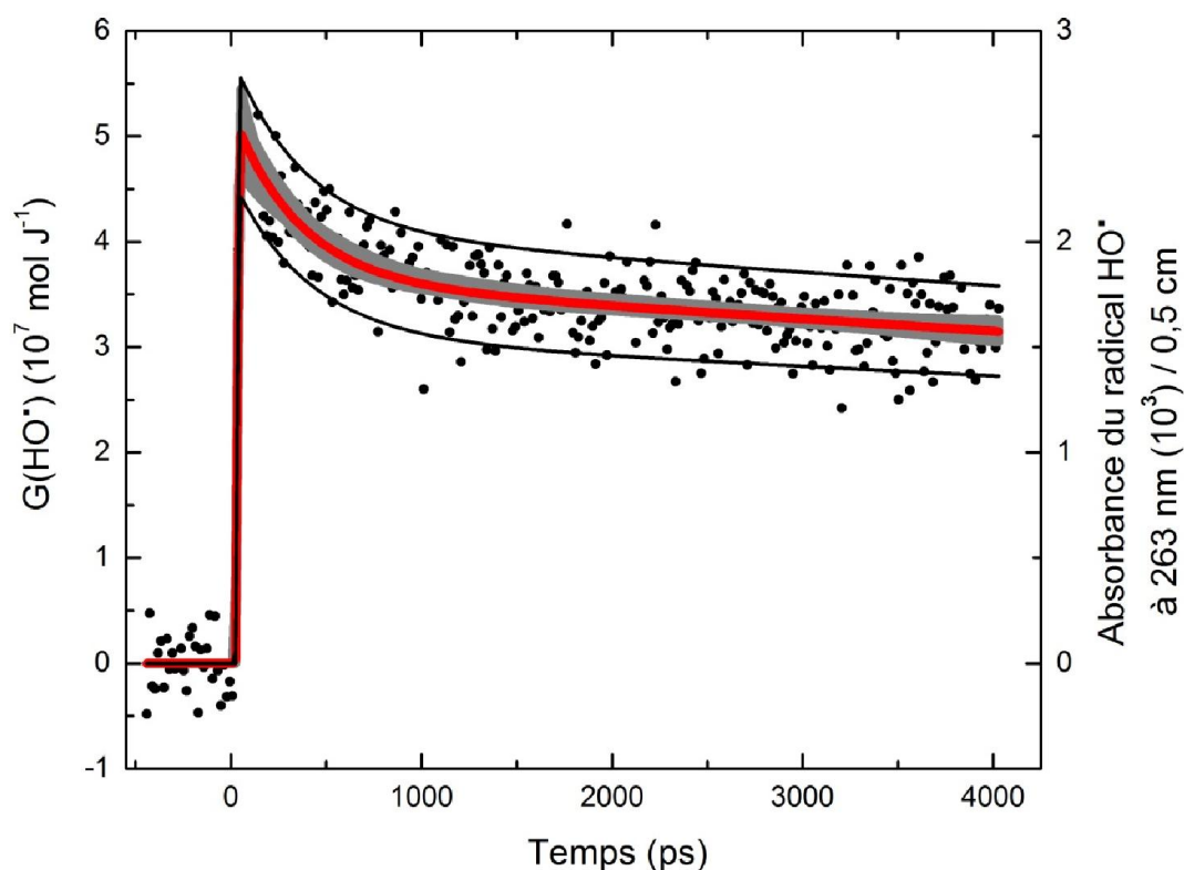
Figure IV. 12 Rendement radiolytique dépendant du temps (axe des ordonnées à gauche) et absorption transitoire (axes des ordonnées à droite) du radical HO• à temps long. La ligne rouge représente le meilleur ajustement des données expérimentales selon une fonction biexponentielle et la région grise représente l'incertitude de l'enregistrement. Les lignes noires représentent le déclin du radical HO• en considérant un rapport des coefficients d'absorption molaire du radical HO• et de l'électron hydraté 10 % plus ou moins élevé que les valeurs reportées dans la littérature. 20
