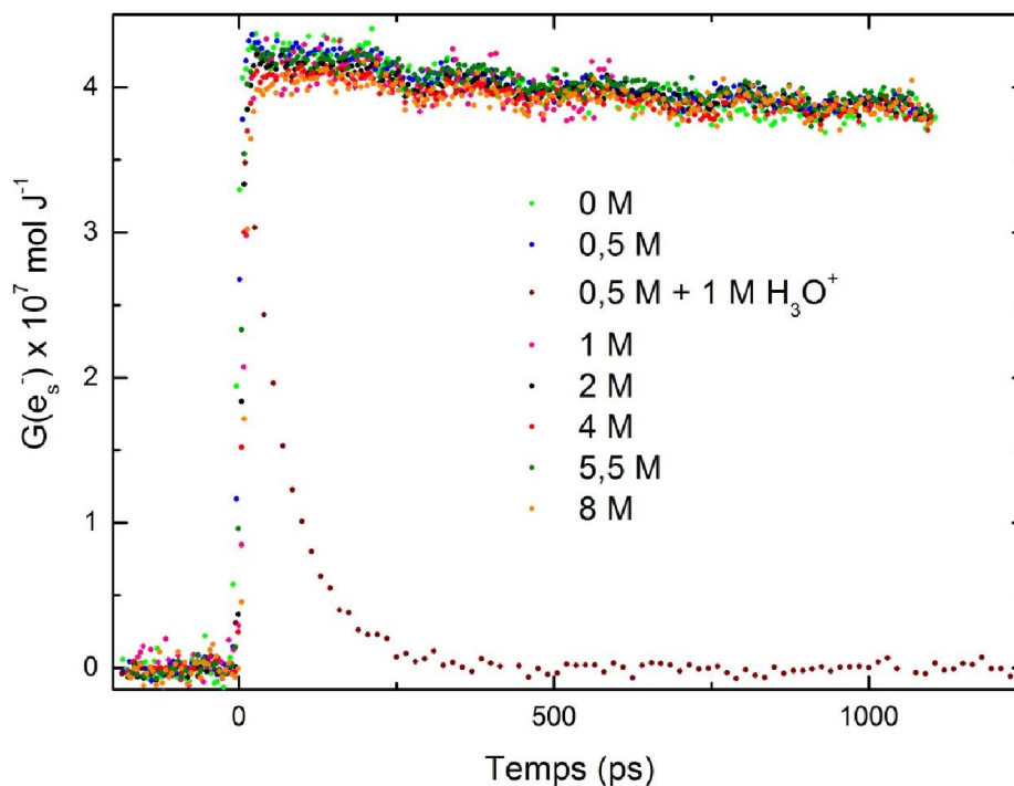
Figure V. 12 Rendement radiolytique de l'électron hydraté dépendant du temps, calculé pour diverses solutions aqueuses. Ce rendement est obtenu après la normalisation par le facteur F et en tenant compte du degré de déplacement de la bande d'absorption (changement de coefficient d'absorption molaire).
