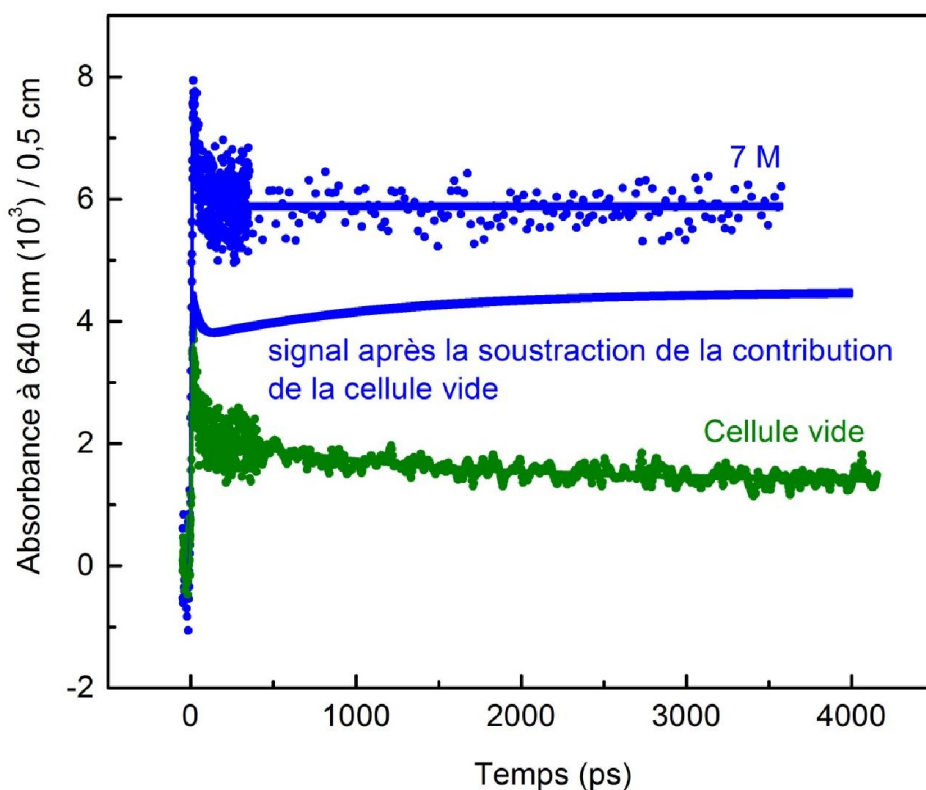
Figure V. 5 Cinétique enregistrée à 640 nm dans la cellule vide (vert) et en présence de solution d'acide nitrique de 7 mol L -1 (bleu). La ligne bleue représente la contribution du radical NO 3 • après la soustraction de la contribution de la cellule vide.
