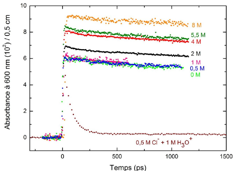
Figure V. 9 Déclins non normalisés observés dans des solutions aqueuses et dans l'eau pure, enregistrés à 600 nm mais après soustraction de la contribution des fenêtres de la cellule d'irradiation. 30
