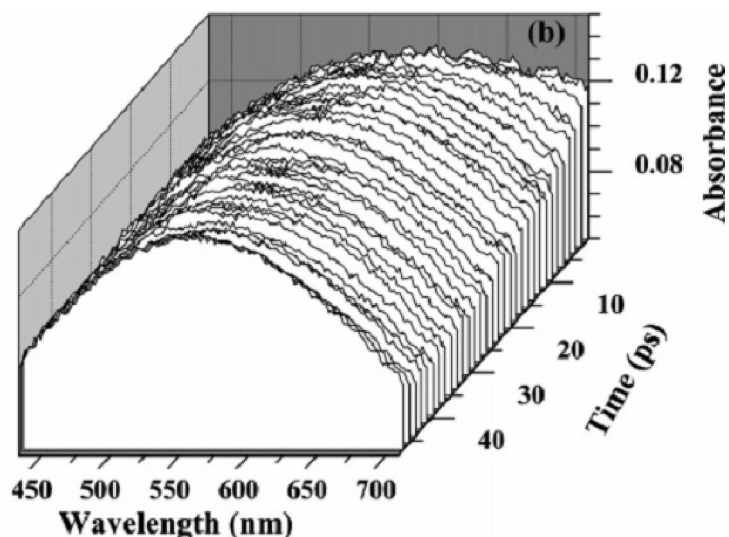
Figure II. 21 Evolution temporelle du spectre d'absorption de l'électron solvate dans l'éthylène glycol, après la photoionisation de ce dernier à 263 nm. 139
