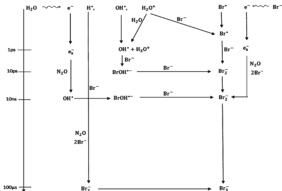
Figure II. 18 Mécanisme d'oxydation directe et indirecte des ions \text{Br}^- suite à l'irradiation de solutions aqueuses concentrées de bromure de sodium saturée en \text{N}_2\text{O} . L'oxydation directe est obtenue suite à l'interaction du rayonnement ionisant avec les ions \text{Br}^- alors l'oxydation indirecte est le résultat des réactions chimiques entre les produits radicalaires de la radiolyse de l'eau et ions \text{Br}^- . 122
