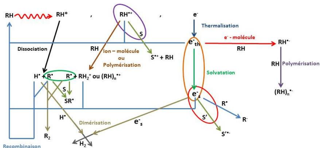
Figure II. 23 Schéma résumant les processus chimiques déclenchés par l'absorption d'un rayonnement ionisant par un solvant noté RH. Les cercles désignent les processus étudiés au courant de cette thèse.
