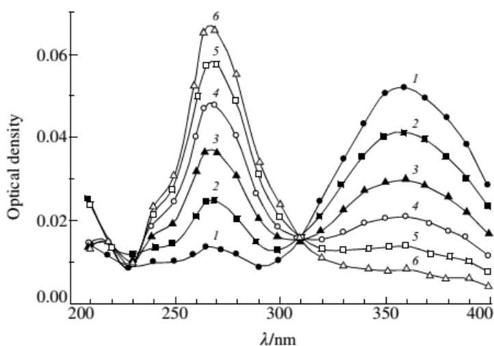
Figure II. 17 Spectres d'absorption d'une solution de NaBr à 0,1 \text{ mol L}^{-1} , saturée en \text{N}_2\text{O} à un pH de 3,3 correspondant à (1) : 1, (2) : 8, (3) : 24, (4) : 50, (5) : 100 et (6) : 250 ms après l'impulsion d'électrons. 121
