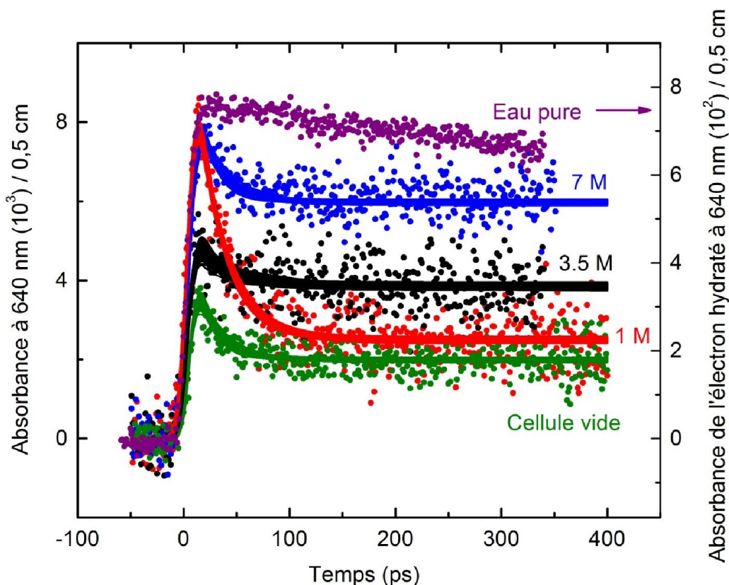
Figure V. 3 Cinétiques à 640 nm enregistrées directement après le passage du faisceau d'électrons dans l'eau (axe des ordonnées à droite), dans des solutions de \text{HNO}_3 à 1 ; 3,5 et 7 mol \text{L}^{-1} , ainsi qu'au sein de la cellule vide (axe des ordonnées à gauche). Les lignes ont été tracées par analyse bayésienne utilisant une équation multi-exponentielle associée à une fonction de réponse gaussienne. L'épaisseur des lignes représente les incertitudes du modèle.
