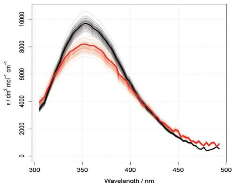
Figure II. 16 Spectres d'absorption des espèces \text{Br}_2^{\cdot-} (noir) et \text{BrOH}^{\cdot-} (rouge) obtenues par analyse bayésienne. Les meilleurs fits sont représentés par les lignes en gras. 109
