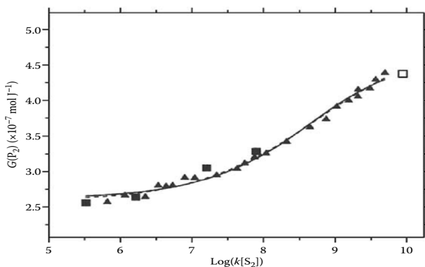
Figure II. 10 Valeurs prédites du rendement radiolytique du radical HO • en fonction du pouvoir de capture. La ligne solide représente le meilleur ajustement des données. 25
