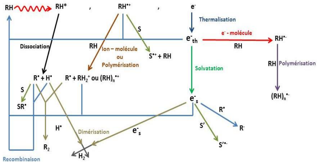
Figure II. 2 Schéma résumant les processus chimiques déclenchés par l'absorption d'un rayonnement ionisant par un solvant noté RH. 7,25
