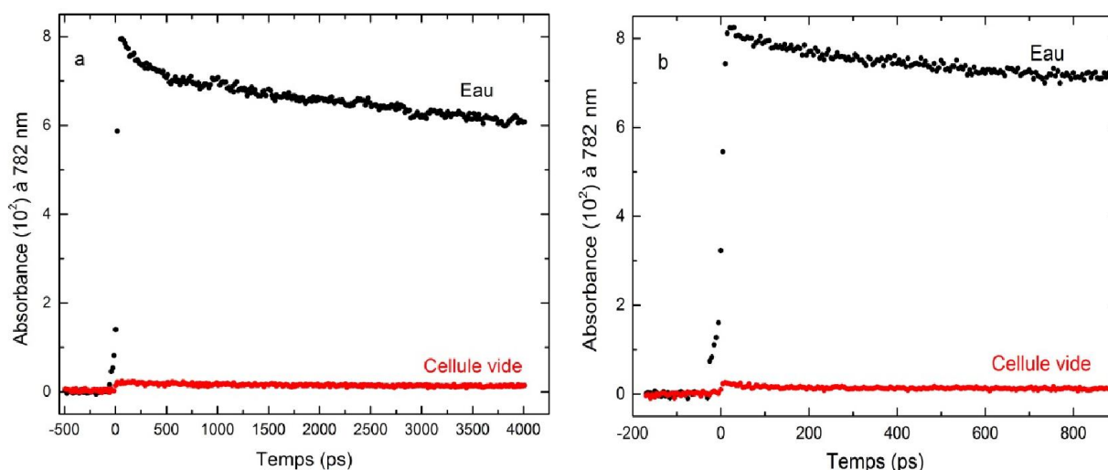
Figure IV. 8 Mesures pompe-sonde à 782 nm de la cellule optique en absence (rouge) et en présence d'eau (noir). Les mesures longues (figure a) et courtes (figure b) sont effectuées sous les mêmes conditions expérimentales avec les données enregistrées chaque pas de 15 et 5 ps respectivement. 20
