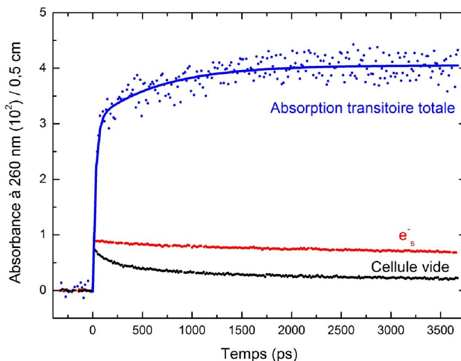
Figure V. 26 Absorption transitoire totale enregistrée à 260 nm (bleu) ainsi que les contributions de l'électron hydraté (rouge) et de la cellule vide (noir). La ligne bleue représente un guide pour l'oeil.
