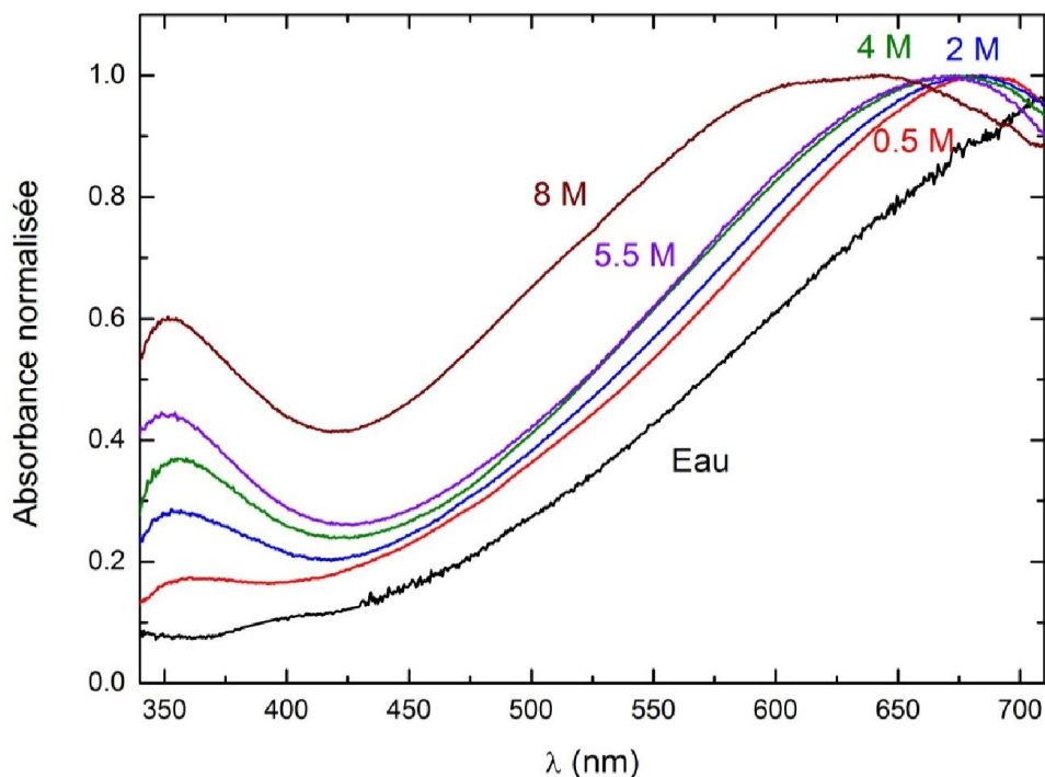
Figure V. 8 Spectres d'absorption transitoire normalisés des différentes solutions de chlorure, enregistrés directement après le passage du faisceau d'électrons picoseconde.
