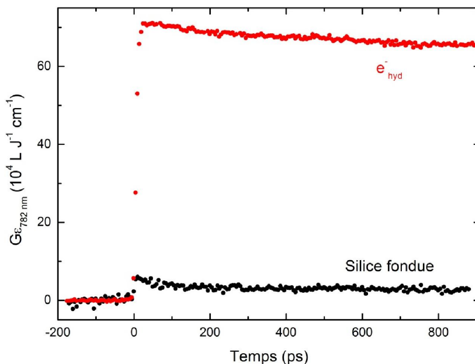
Figure IV. 6 Produit \epsilon_\lambda G(t) à 782 nm en fonction du temps. Comparaison entre l'électron hydraté dans la cellule de silice et la silice fondue seule. 17
