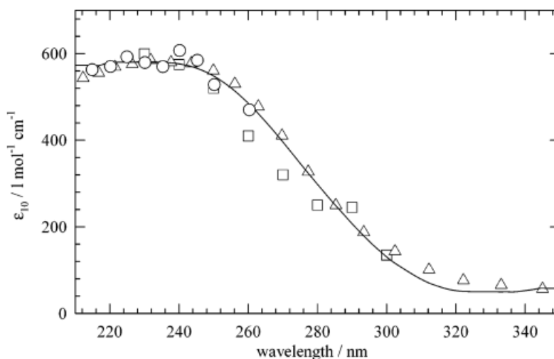
Figure II. 9 Spectre d'absorption du radical HO • dans l'eau, (-) : Hesper et Herrmann, (□) : Jayson et al. , (○) : Nielsen et al. , (Δ) compilé par Hartmut Herrmann. 67
