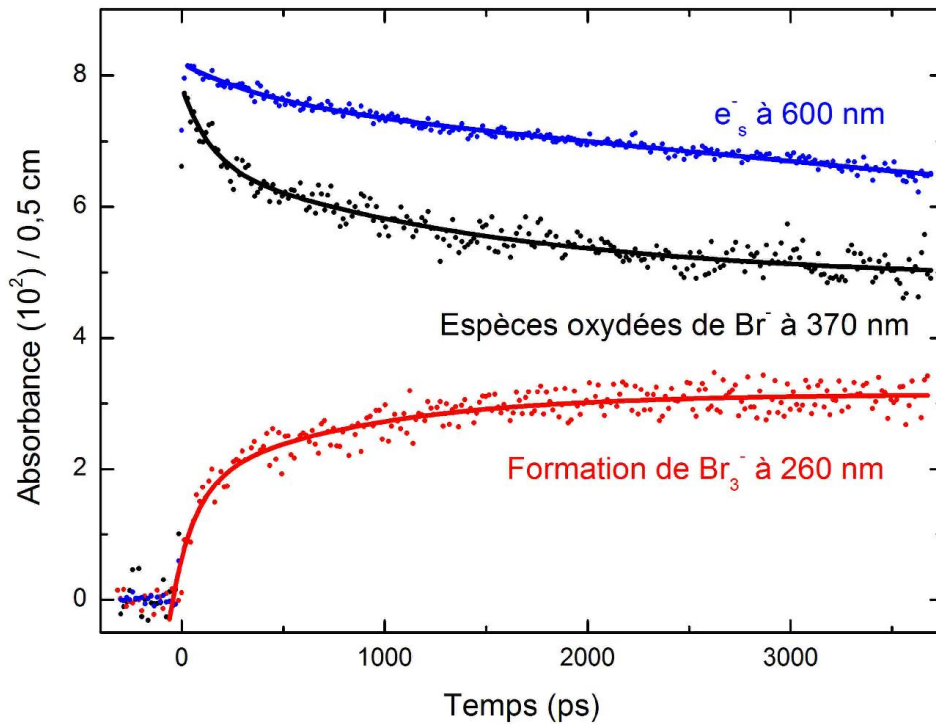
Figure V. 27 Cinétiques enregistrées à 600, 370 et 260 nm concernant respectivement le déclin de l'électron solvaté (bleu), le déclin des espèces oxydées de l'ion Br - (noir) et la formation de Br 3 - (rouge).
