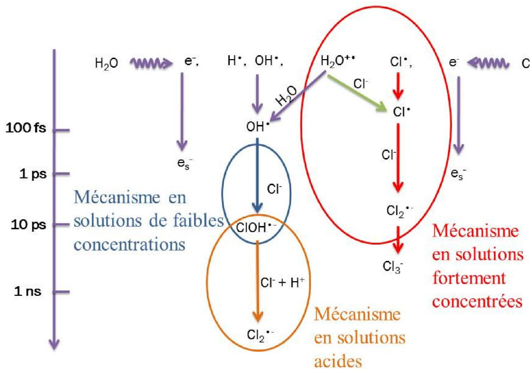
Figure V. 18 Mécanisme d'oxydation des ions Cl - dans les solutions chlorées aqueuses diluées et concentrées.
