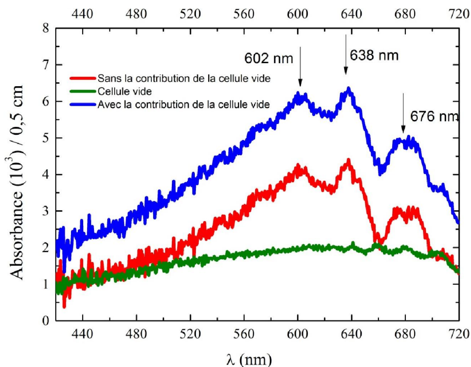
Figure V. 2 Spectres d'absorption transitoires enregistrés à 200 ps après le passage du rayonnement ionisant au sein d'une solution d'acide nitrique à 7 \text{ mol L}^{-1} (bleu) et des fenêtres de la cellule de circulation vide (vert). Le spectre rouge, provenant de la solution d'acide nitrique est obtenu par soustraction de la contribution de la cellule vide à partir du spectre bleu.
