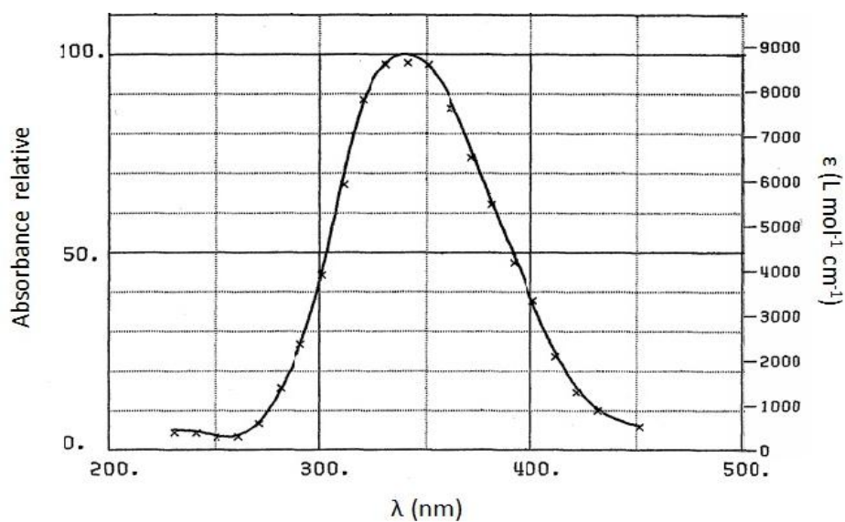
Figure II. 14 Spectre d'absorption de \text{Cl}_2^{\cdot-} obtenu par irradiation d'une solution de \text{NaCl} à 3 \text{ mol L}^{-1} en milieu neutre saturé soit par \text{N}_2\text{O} soit par \text{O}_2 . 77 Les valeurs des coefficients d'absorption molaires « \epsilon » sont corrigées par Buxton et al. 79
