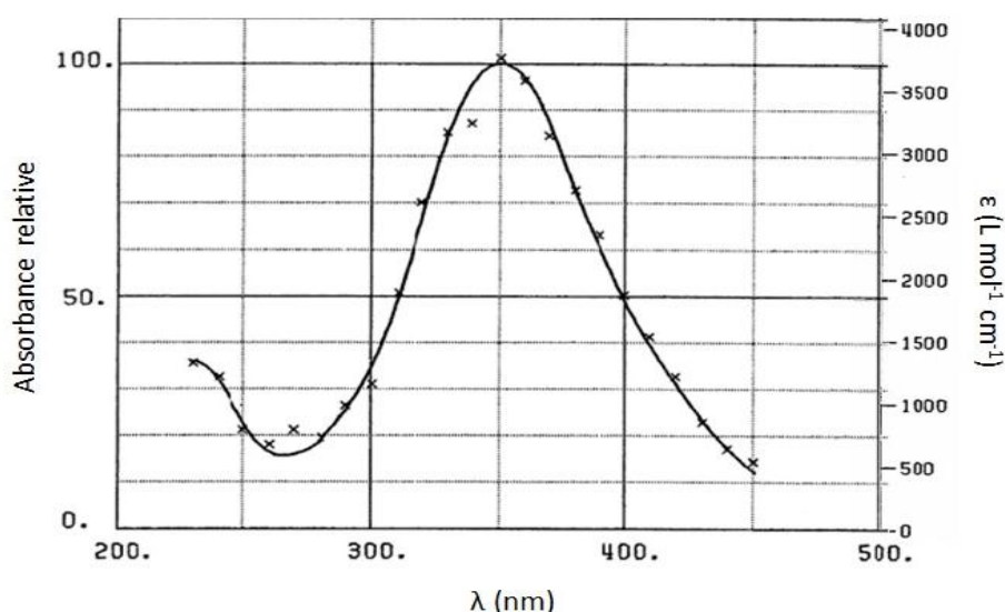
Figure II. 13 Spectre d'absorption de \text{ClOH}^{\cdot-} obtenu par irradiation d'une solution de \text{NaCl} à 3 \text{ mol L}^{-1} en milieu neutre saturée soit par \text{N}_2\text{O} soit par \text{O}_2 . 77 Les valeurs des coefficients d'extinction molaires « \varepsilon » sont corrigées par Buxton et al. 79
