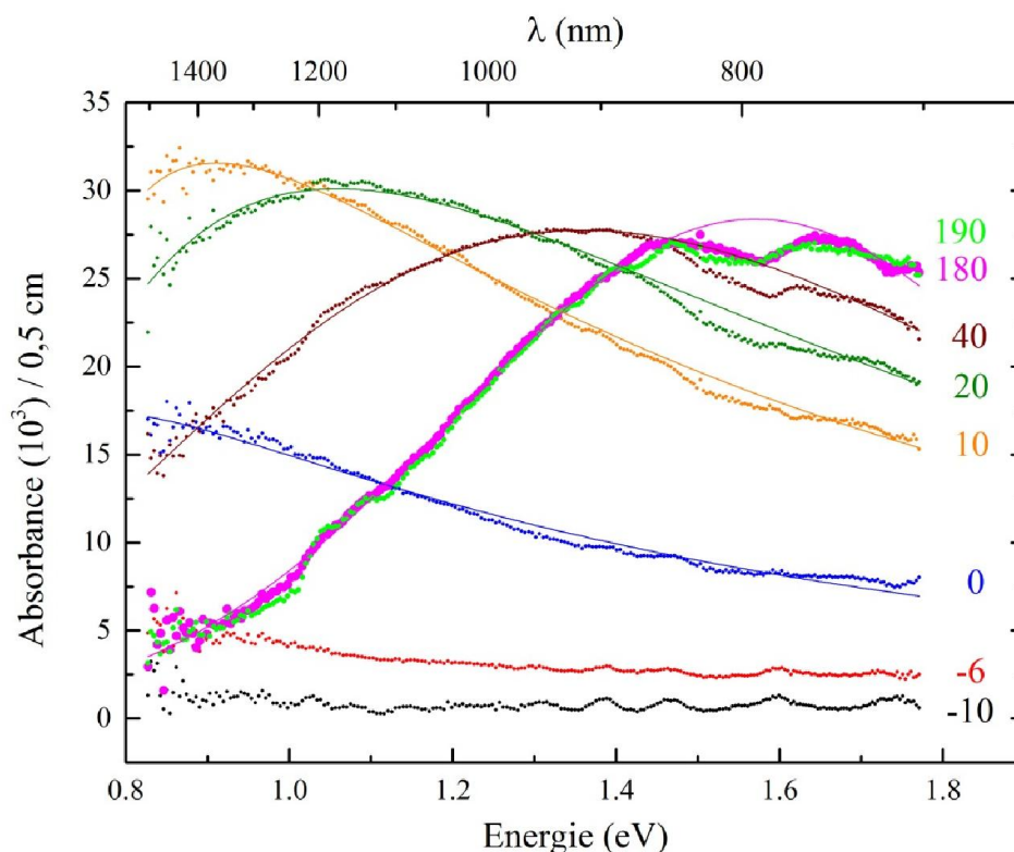
Figure VI. 2 Quelques spectres d'absorption transitoire de l'électron dans le propan-2-ol en fonction du temps. L'axe des abscisses du bas montre les valeurs de l'énergie en eV de la transition alors que celui du haut affiche les longueurs d'onde correspondantes.
