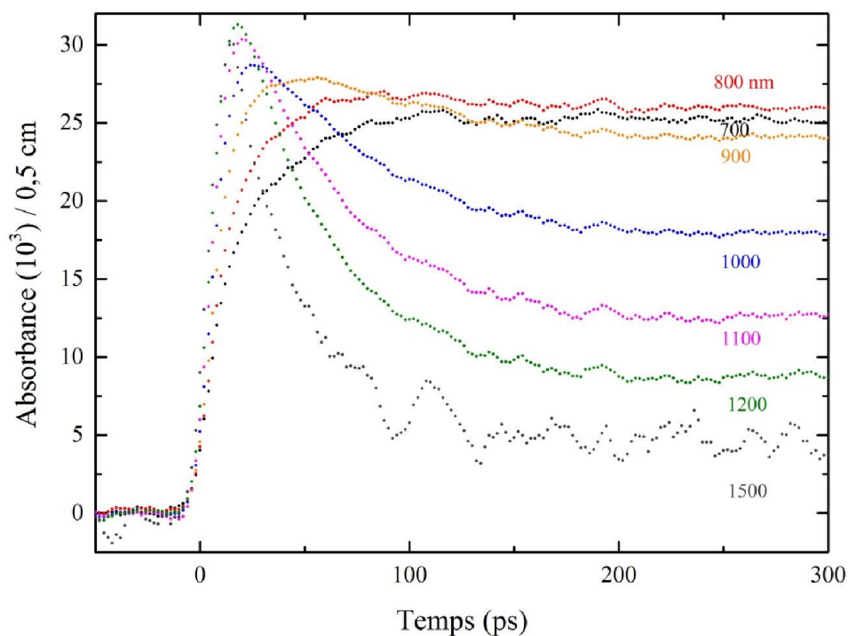
Figure VI. 3 Cinétiques de la solvatisation de l'électron dans le propan-2-ol en fonction de la longueur d'onde.
