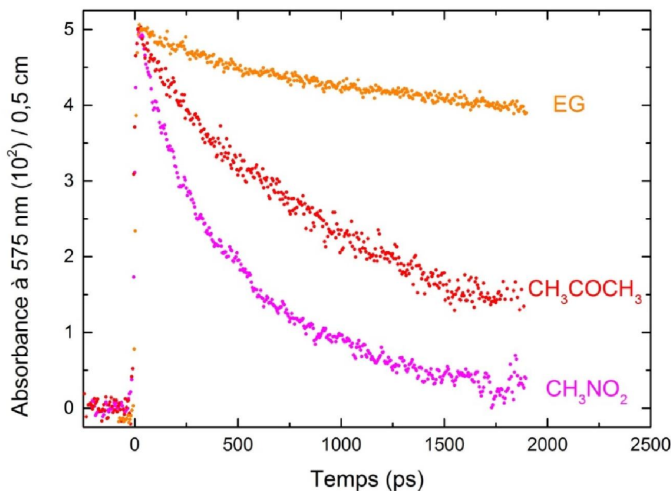
Figure VI. 14 Comparaison des cinétiques de déclin de l'électron solvaté enregistré dans l'éthylène glycol à 575 nm en absence et présence de \text{CH}_3\text{COCH}_3 ou de \text{CH}_3\text{NO}_2 . Les absorbances initiales ont été normalisées à celle enregistrée dans le solvant pur.
