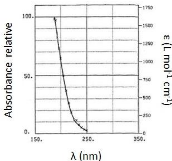
Figure II. 11 Spectre d'absorption du radical H^\bullet en solution aqueuse contenant 3,39 \times 10^{-4} \text{ mol L}^{-1} de HClO_4 , 2,82 \times 10^{-2} \text{ mol L}^{-1} de H_2 et 4,5 \times 10^{-5} \text{ mol L}^{-1} de H_2O_2 . 39,59
