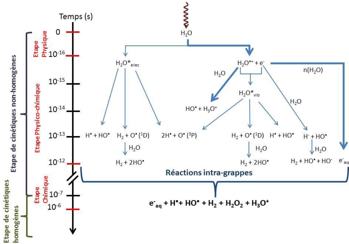
Figure II. 3 Schéma général de la radiolyse de l'eau 29,32 . L'épaisseur des flèches indiquent les voies réactionnelles majeures. Les traits rouges au niveau de l'axe des temps définissent les débuts et les fins des différentes étapes de la phase de la cinétique non-homogène puis homogène.
