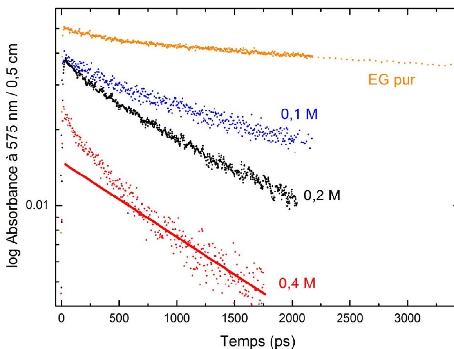
Figure VI. 12 Représentation logarithmique des cinétiques de déclin de l'électron solvaté observées à 575 nm dans l'éthylène glycol pur et en présence de trichlorométhane à différentes concentrations. La ligne solide représente la partie linéaire de la cinétique.
