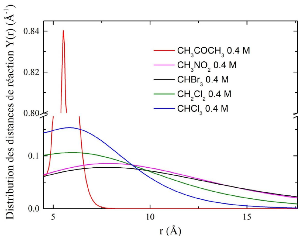
Figure VI. 18 Distribution des distance de réaction Y(r) en présence de 0,4 \text{ mol L}^{-1} de capteurs organiques. La distance de contact est fixée à 4 \text{ \AA} .
