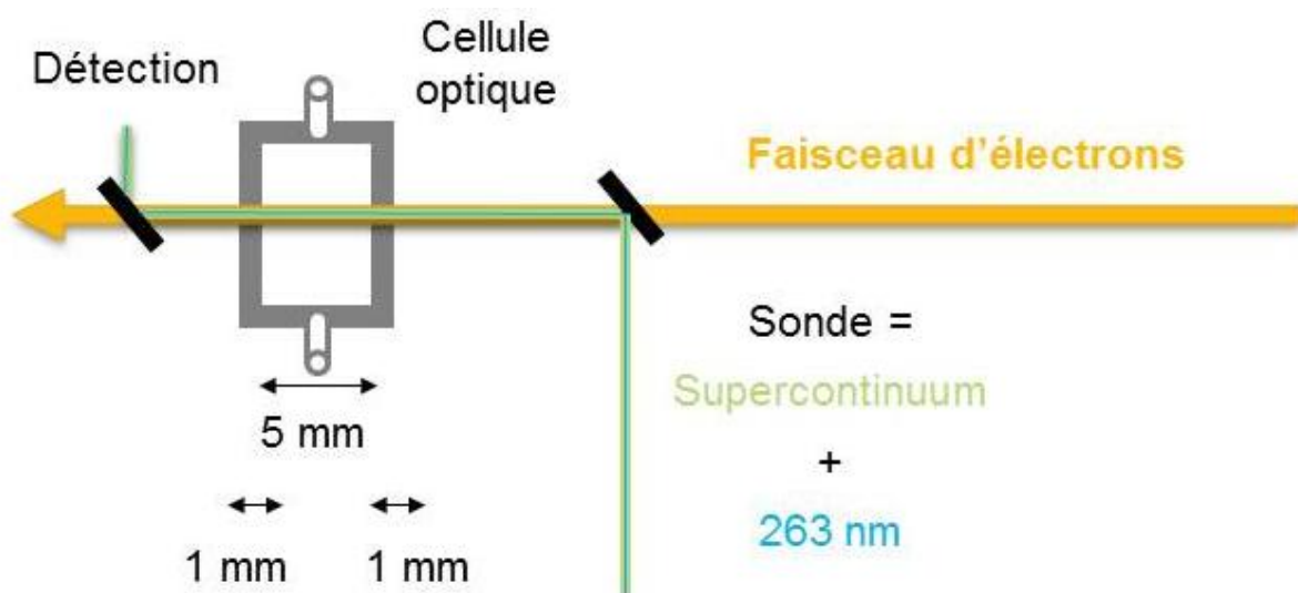
Figure IV. 2 Montage pompe-sonde utilisé dans les mesures d'absorption transitoire picoseconde de la silice fondue. La trait jaune représente le faisceau d'électrons, la trait vert représente le supercontinuum issu du faisceau fondamental du laser par effet d'optique non linéaire et le trait bleu représente la lumière sonde à 266 nm.
